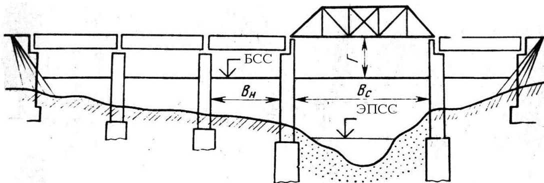
60-rasm. Ko`priknı prolyotlarga bo`lish va kema qatnashi uchun prolyotlar ajratish
