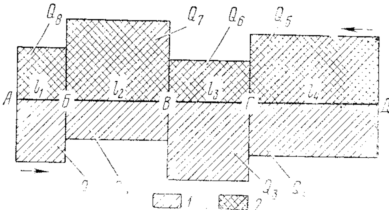
30-rasm. Yukli zo'riqish epyurasi.
