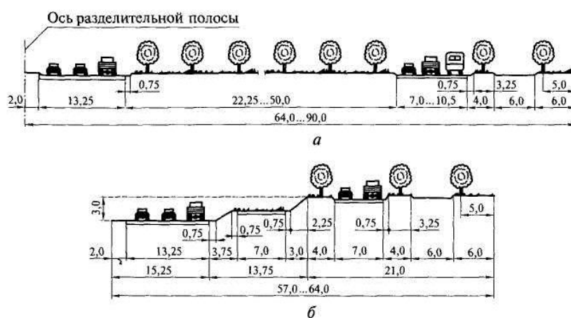
9-rasm. Tezyurur shahar yo'llari ko'ndalang kesimi (o'lchamlar m da): a – bir satxda; b – o'ymada.
