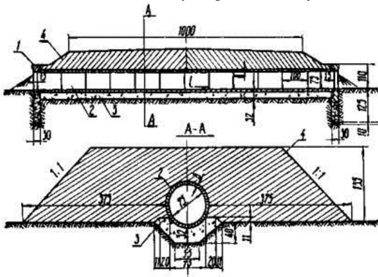
56-rasm. Quvur sxemasi: 1 - kallak, 2 – quvur zvenosi, 3 - qum-shag`alli yostiqla, 4 – tuproq bilan to`ldirilgan
