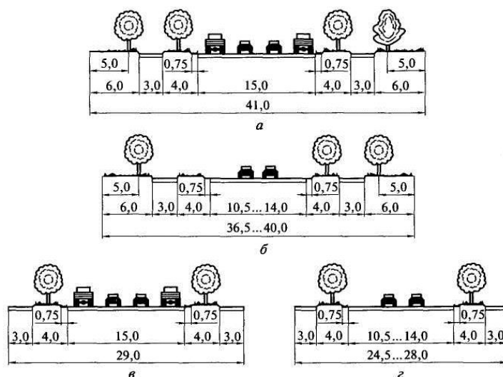
10-rasm. Tuman ahamiyatidagi magistral ko'cha ko'ndalang kesimi ( a, v ) va ( b, g ) aholi yashash ko'chalari: a, b – ko'kalamzorlashgan tasma bilan; v, g – ko'kalamzorlashgan tasmasiz
