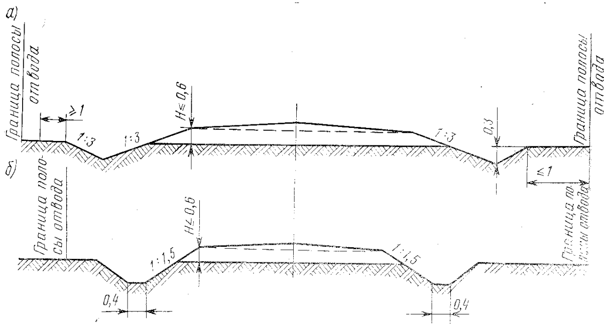
18-rasm. Balandligi 0,6 metrgacha bo'lgan uymaning bo'ylama qirqimi (profil) a) uchburchak kesim yuzali arig'i bilan; b) trapetsiya kesim yuzali arig'i bilan.
