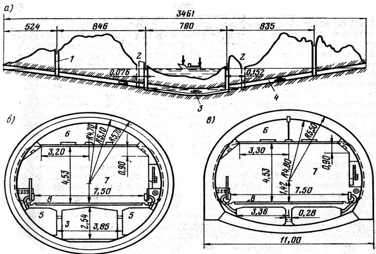
66-rasm. Suvosti tonneli:
