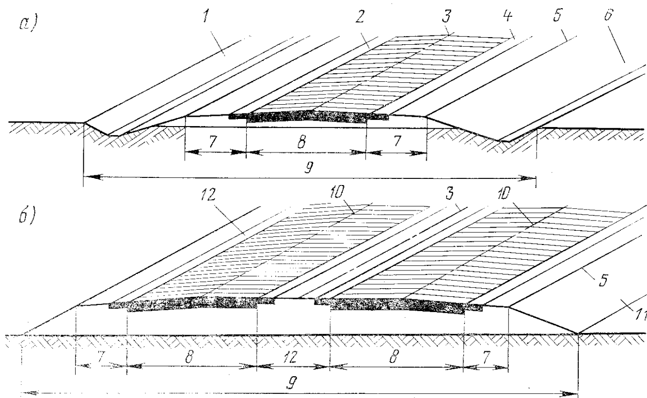
16-rasm. Yo`lning ko`ndalang kesim bo`yicha qism (element)lari.
