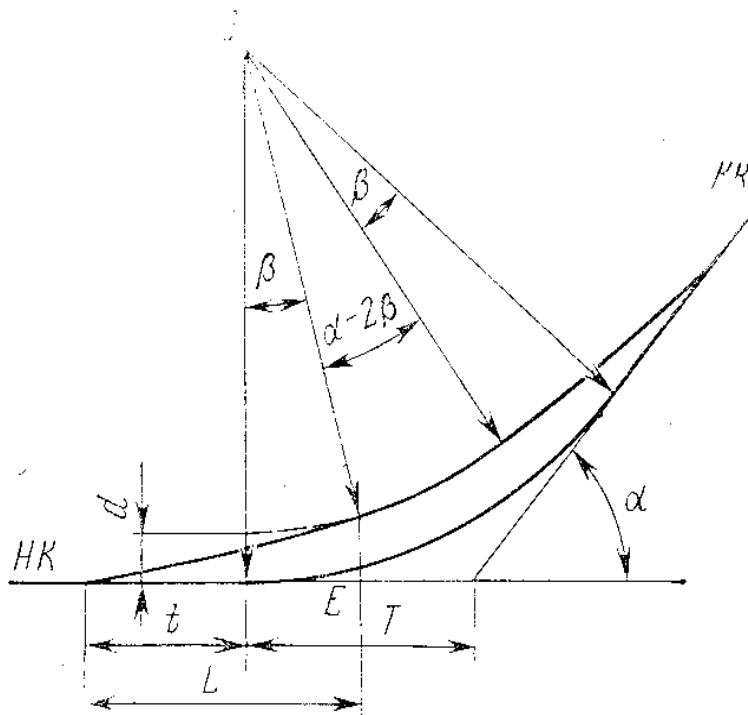
26-rasm. Oʻtkinchi egrilikni qilinayotgan egrilik bilan joylashtirish chizmasi.
