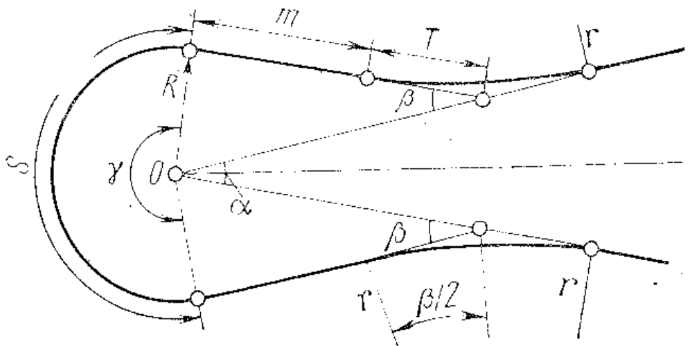
27-rasm. O'tkinchi egri chizikli simmetrik serpantin.
