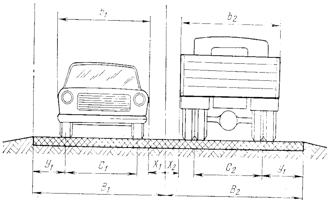
21-rasm. Harakat bo`lagi kengligini aniqlovchi shakl.
