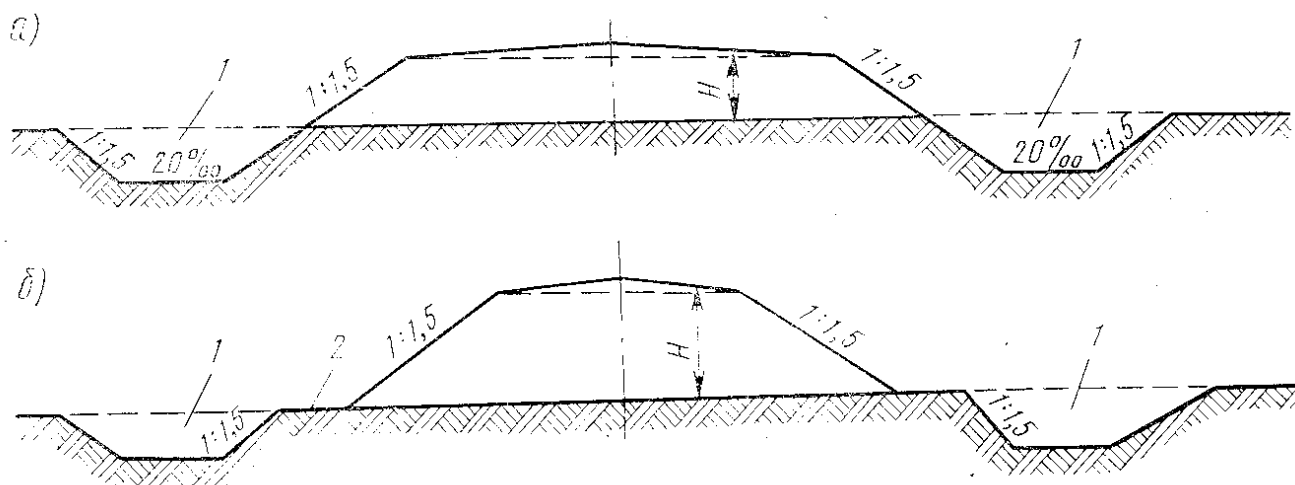
19-rasm. Balandligi 0,6 metrdan yuqori bo'lgan uymaning bo'ylama qirqimi. 1 – zahira; 2 –supacha.
