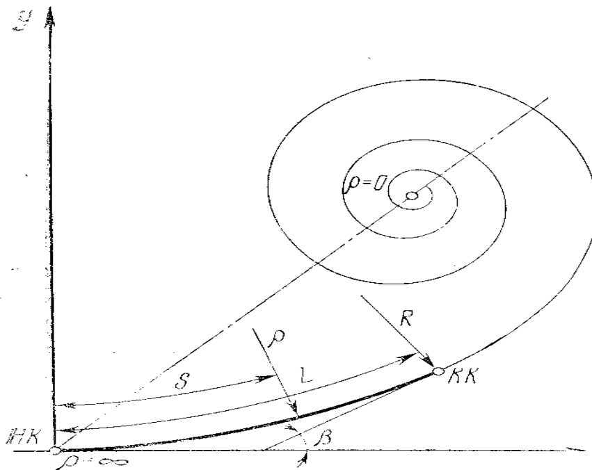
25-rasm. Klotoida.
