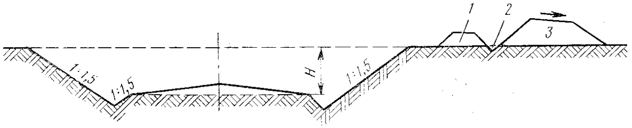
20-rasm. O'yib olingan qismning ko'ndalang qirqim shakli (profil)
