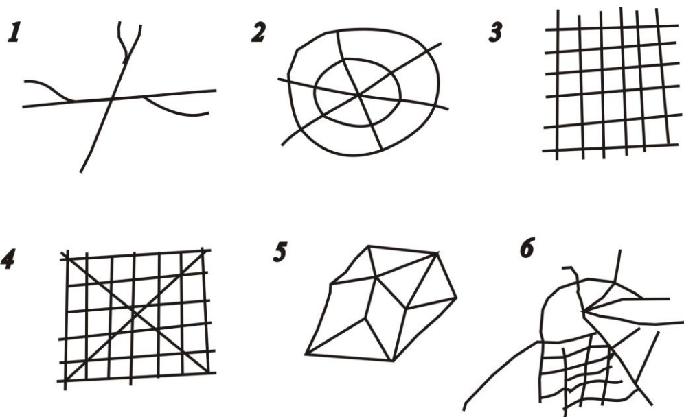
11-rasm. Shahar ko`cha-yo`l tarmoqlari joylashish sxemalari.
