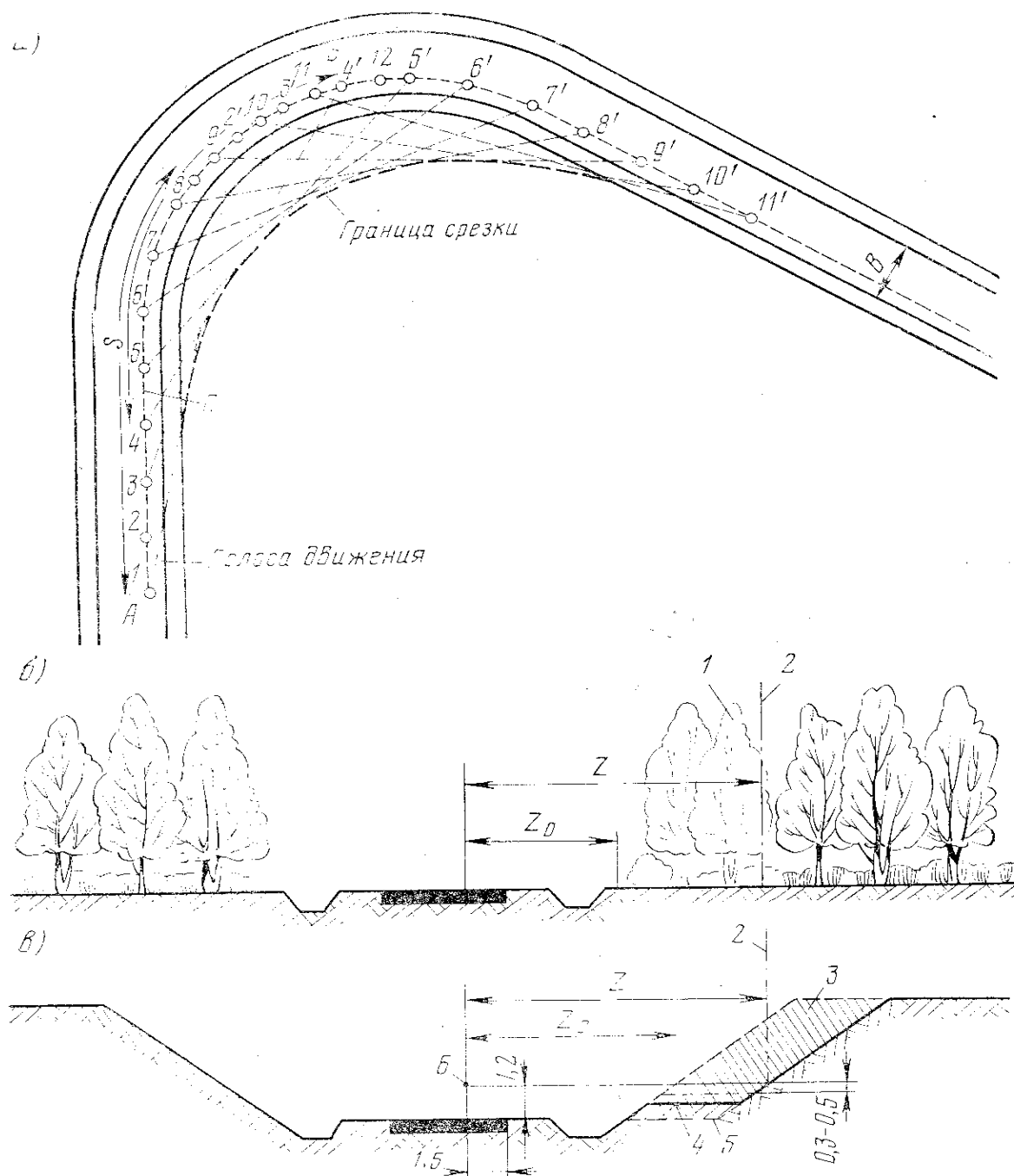
29-rasm. Yo'lning egri qismidagi ko'rinishni umumiy shakl (plan)da ta'minlash. a) Ko'rinish qirqim chegarasini chizmalı ifodasi; b) Daraxtzorlarni kesib tashlash chegara; v) Qirqib tashlash va o'yib olish; V – qatnov qismi kengligi, P – avtomobilning harakatlanish bo'lagi, 1-daraxtlardan tozalash qismi, 2-ko'rinish
