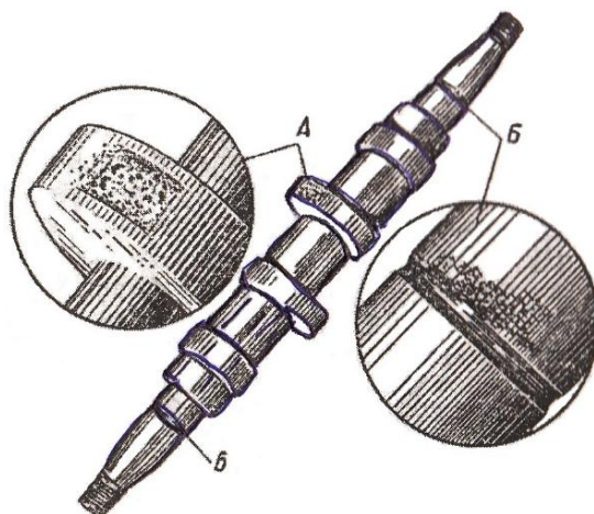
3.2-rasm. Yonilg'i nasoslari kulachokli valining eyilishi:
