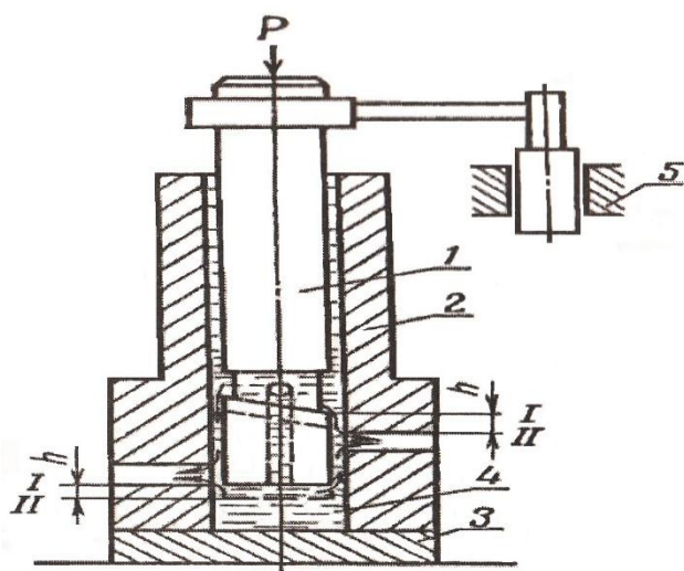
3.5-rasm. Plunjer juftligining germetikligini tekshirish asbobining sxemasi:
