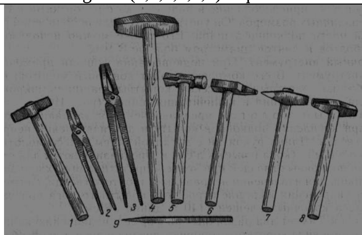
Temirchilik asboblari: (13-rasm)
