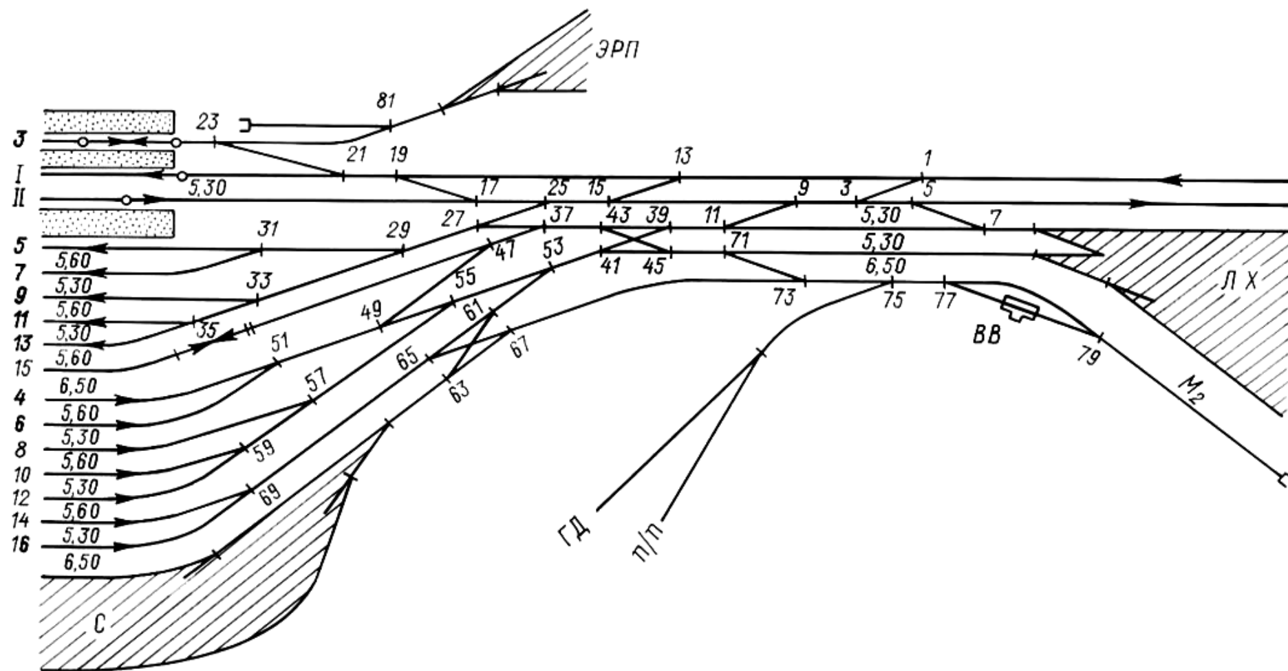
6-rasm. Ikki yo`lli liniyaning ko`ndalang tipdagi uchastka stansiyasi markaziy «bo`g`iz»i sxemasi
