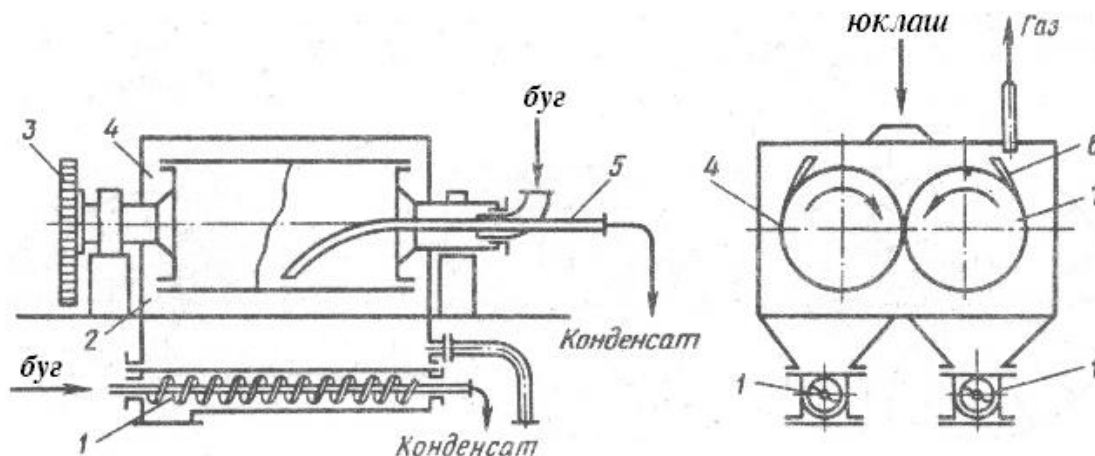
21-расм. Жували қуриткич.
