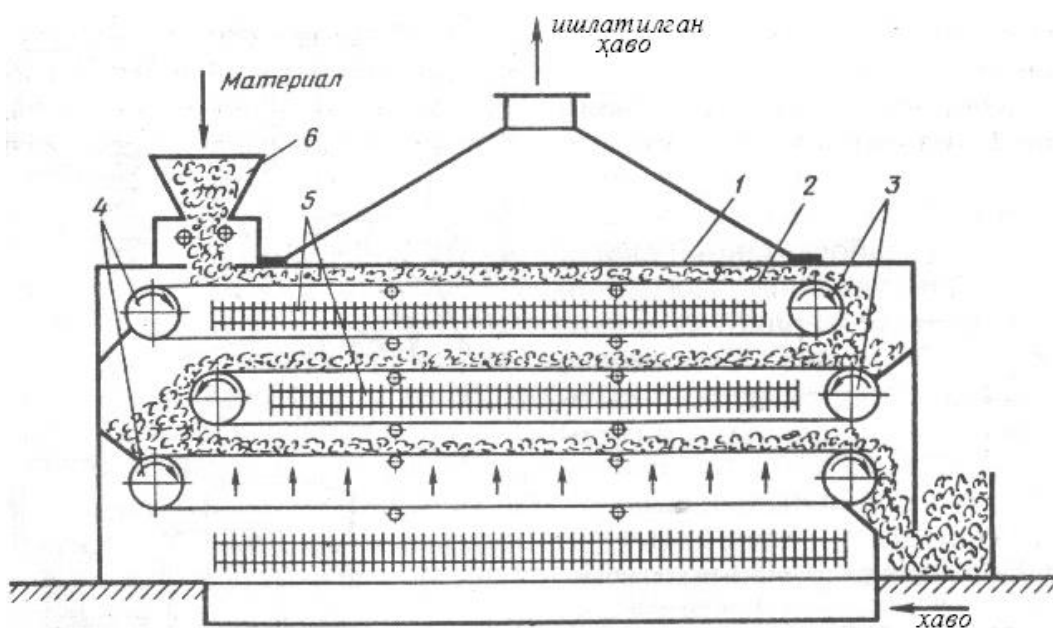
14-расм. Лентали куриткич.
