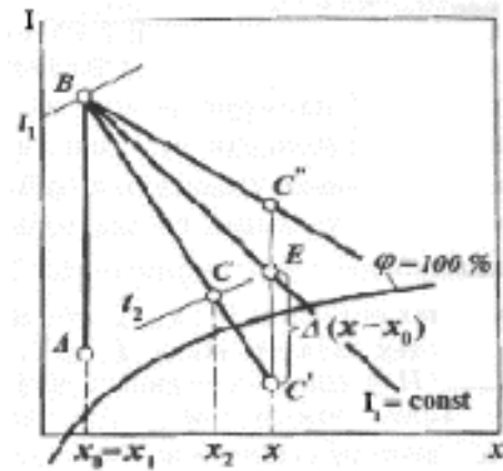
11а-расм. I-x диаграммада қуритиш чизигини аниқлаш.
