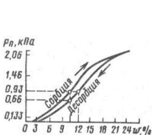
5-расм. Крахмал намлигининг сорбция – десорбция изотермалари.
