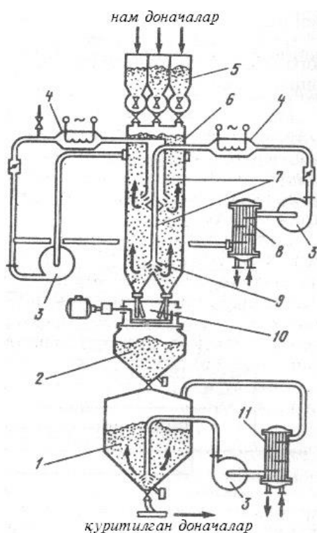
15-расм. Сочилувчан, донатор материалларни қуритиш учун шахтали қуриткич.
