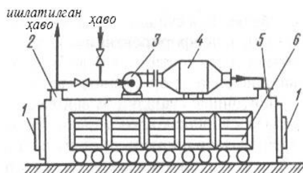
13-расм. Туннелли куриткич.
