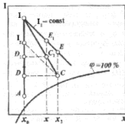
10-расм. Қуритиш жараёнининг ишчи чизигини I-x диаграммада тасвирлаш.
