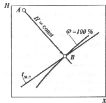
4.в-расм. I - x диаграммада хўл термометр температурасини аниқлаш.
