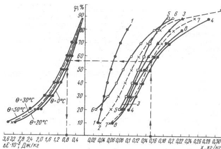
7-расм. Турли маҳсулотларда намликни боғланиш энергиясини аниқлаш чизмаси.
