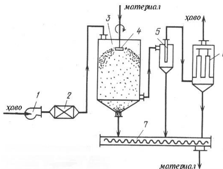
22-расм. Пурковчи қуриткич. 1 - вентилятор; 2 - калорифер; 3 - қуритиш камераси; 4 - диск; 5 - циклон; 6 - енгли филтър; 7 - қуритилган материални тўқувчи шнек.
