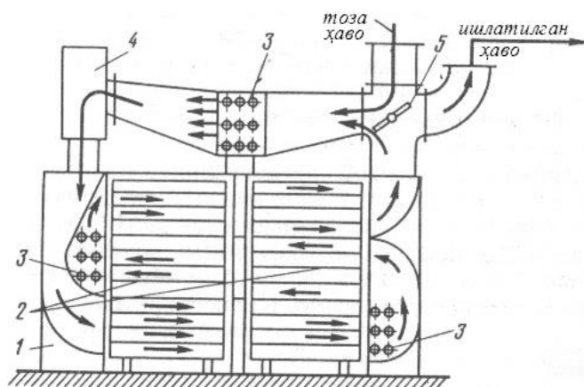
12-расм. Камерали куриткич.
