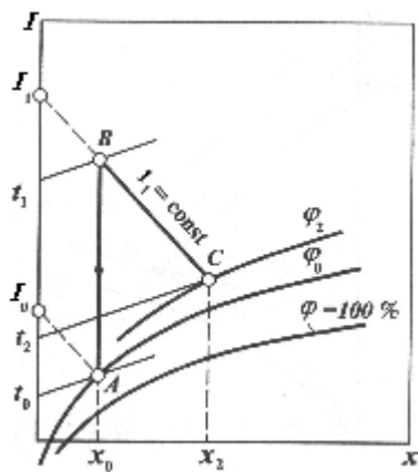
9-расм. I-x диаграммада назарий қуритиш жараёни-нинг график тасвири.
