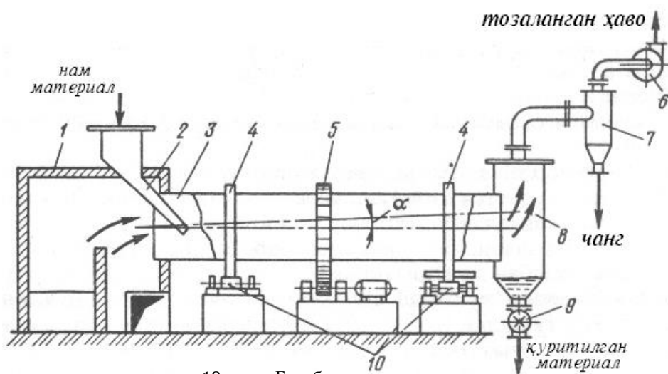
18-расм. Барабанли куриткич.
