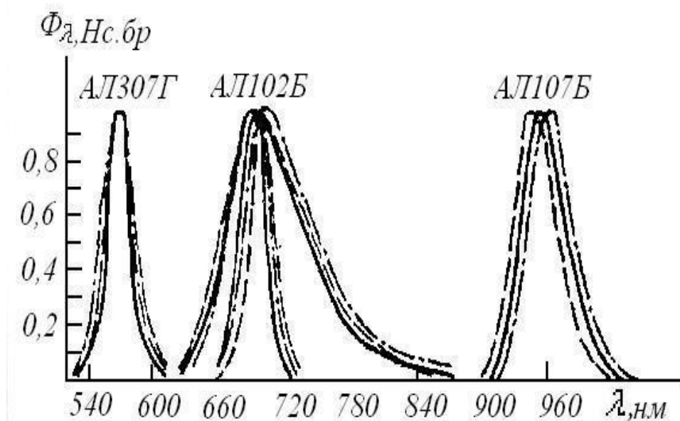
2.1.6.-расм. Ёруғлик диодининг спектрал характеристикасининг температурaviй тарқоқлиги.
