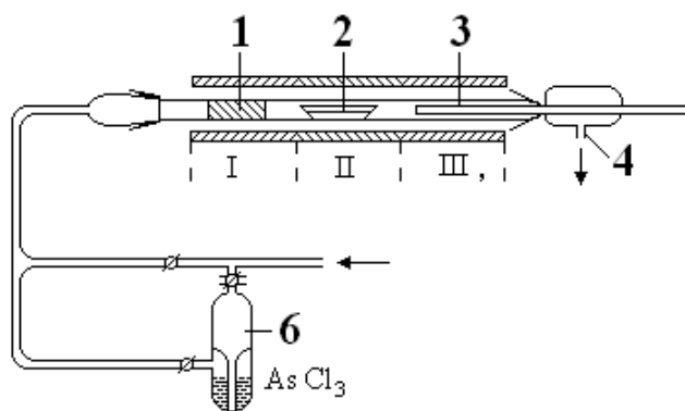
2.3.1-расм. Ga-AsCl 3 -H 2 тизимида GaAs эпитаксиал қатламлар олиш учун қурилма схемаси: 1-асений зонаси 425 0 С (I); 2-галлий зонаси 800 0 С (II); 3-тағлиқ зонаси 750 0 С-900 0 С (III); 4-реакция маҳсулотлари чиқиши; 5-водород кириши; 6-AsCl 3 ли барботер.
