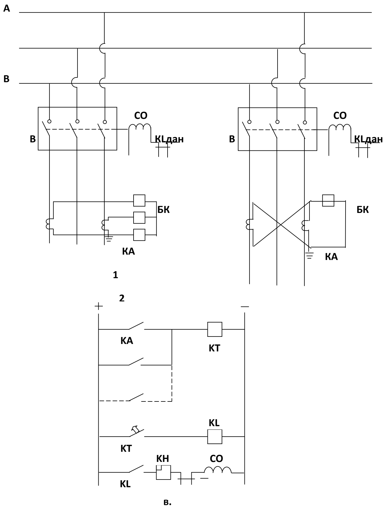
Расм - 5. Максимал ток ҳимояларининг икки фазали схемалари: а-икки релели; б-бир релели в-оператив ток схемаси.
