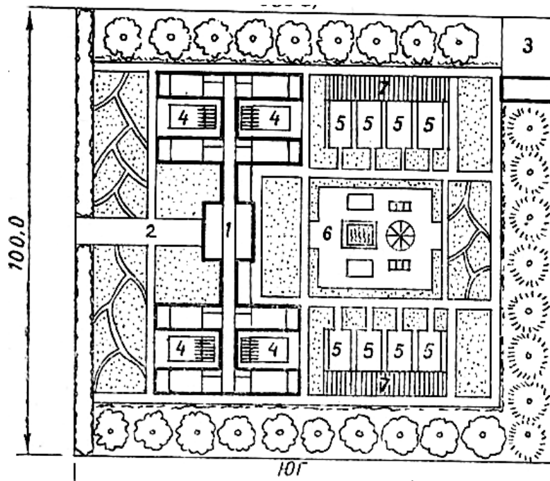
6-расм. Мактабгача болалар муассасалари ҳудудларини ташкил этиш схемаси. 1 – Мактабгача болалар муассасалари биноси, 2 – кириш аллеяси, 3 – хўжалик ҳовлиси, 4 – ясли ёшидаги болалар учун майдонча, 5 – гурҳли ўйин майдончалари, 6 –ўйинлар учун умумий майдонча, 7 – соя тушурувчи айвонлар.
