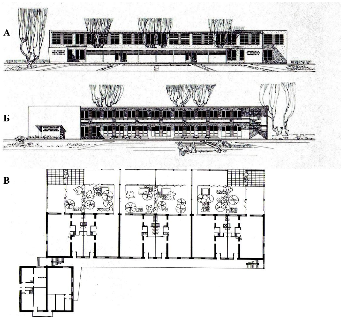
5-расм. Ўзбекистон турар-жой тузилмаларининг оммавий қурилишида 140 ўринга мўлжалланган галерея типигаги болалар ясли – боғчасининг типли лойиҳаси
