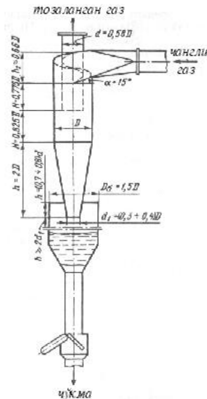
4-расм. НИИОГаз циклон.
