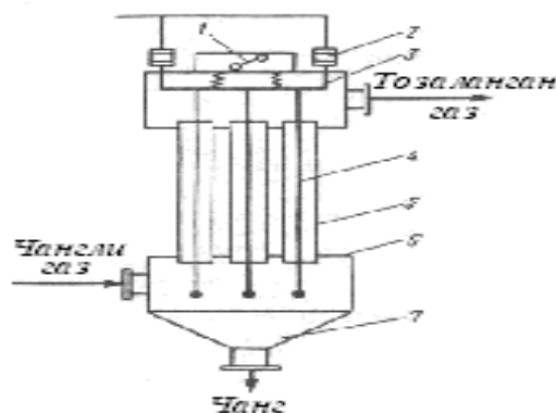
12-расм. Трубади электрофилтр.
