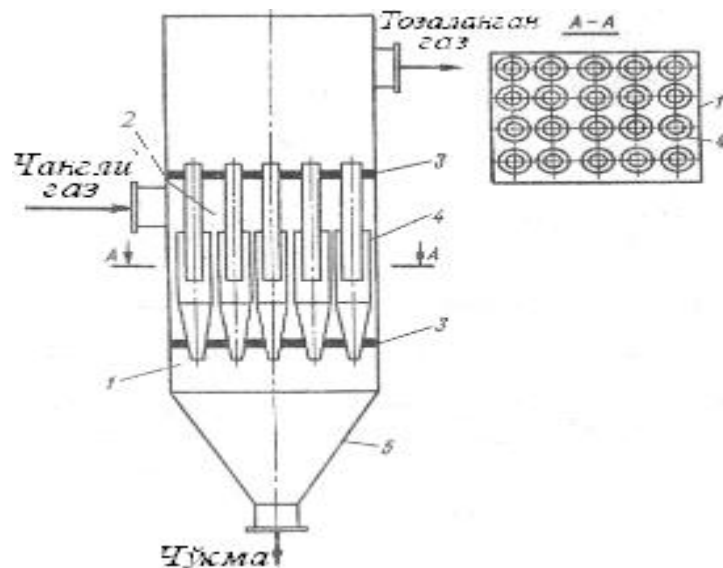
5-расм. Батарейли циклон.
