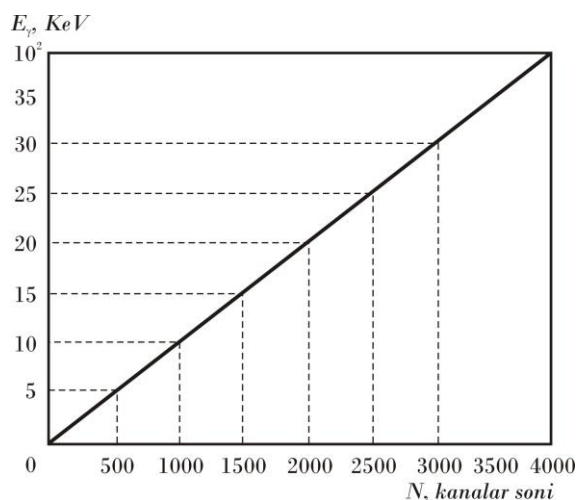
22-rasm. Yarimo 'tkazgichli spektrometrlarning energiya bo'yicha gradirovkasi.
