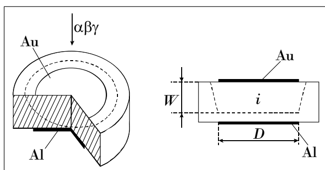
16-rasm. To'siq sirtli Si(Au)-detektorining parametri va tuzilishi.
