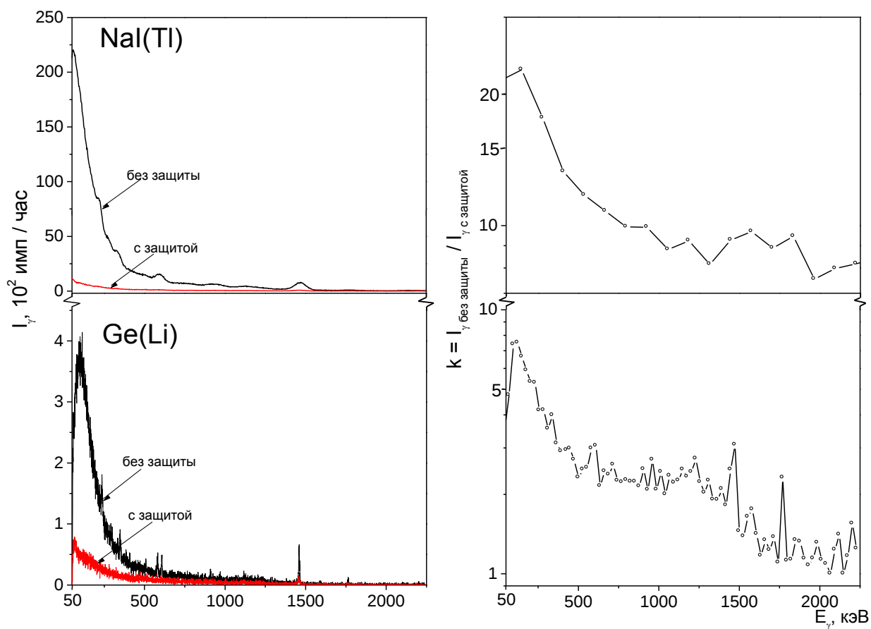
28-rasm. Ge(Li) detektori orqali tabiiy fonni himoya ekransiz va himoyalovchi ekran bilan olingan spektrlari. Himoyalovchi ekran fonni susaytiradi
