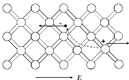
2-rasm. Kremniy panjarasida elektron o‘tkazuvchanlik va teshikning paydo bo‘lishi.
