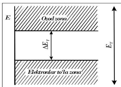
10-rasm. Zonalarning bir-biridan taqiqlangan zona bilan ajralib turishi.
