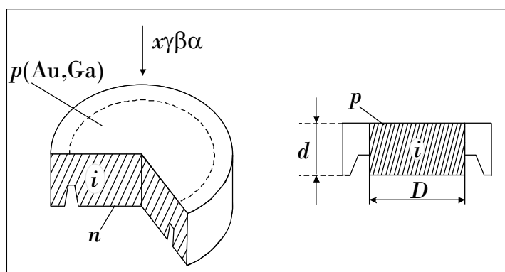
15-rasm. Toʻsiq sirtli Si(Li)-detektorining parametri va tuzilishi.
