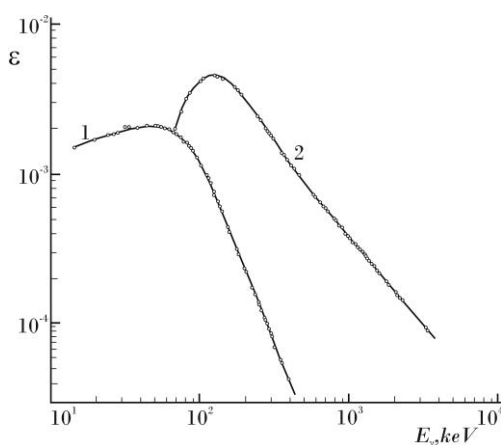
24-rasm. Hajmlari 200\text{mm}^2 \times 5\text{mm} (1) va 38\text{sm}^3 (2) bo‘lgan Ge(Li)-spektrometrlarining nisbiy effektivliklari.
