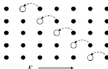
3-rasm. Teshik o‘tkazuvchanlik-ning umumiy ko‘rinishi.
