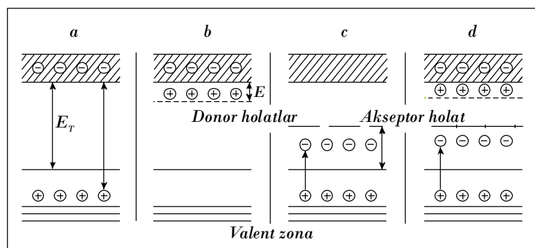
17-rasm. Yarimoʻtkazgichlarda turli xil oʻtkazuvchanlikda energetik holatlarining joylashish sxemasi.
