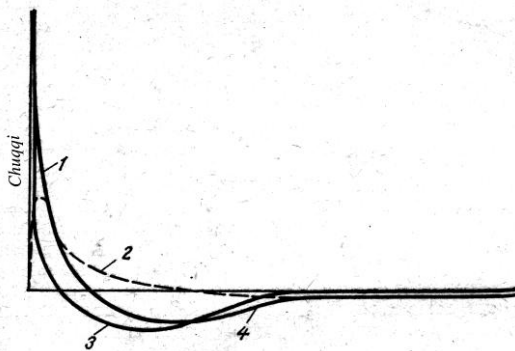
4-rasm. Bir fazali harakat potentsiallarining kelib chiqish mexanizmini tushuntiradigan chizma.
