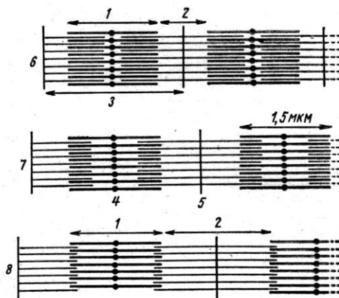
1- rasm. Sut emizuvchilar muskul to'qimasining qisqarish va cho'zilishdagi tuzilishining o'zgarishi.
