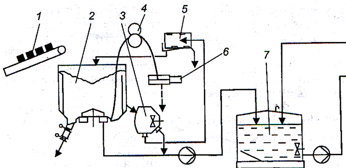
7-расм. Макулатурани титувчи қурилма схемаси: 1 – макулатурани юклаш; 2 – гидропарчалагич; 3 – қўшимча титиш аппарати; 4 – арқонни чиқариб олгич; 5 – сараловчи барабан; 6 – арқон кесгич; 7 – масса ҳавзаси
