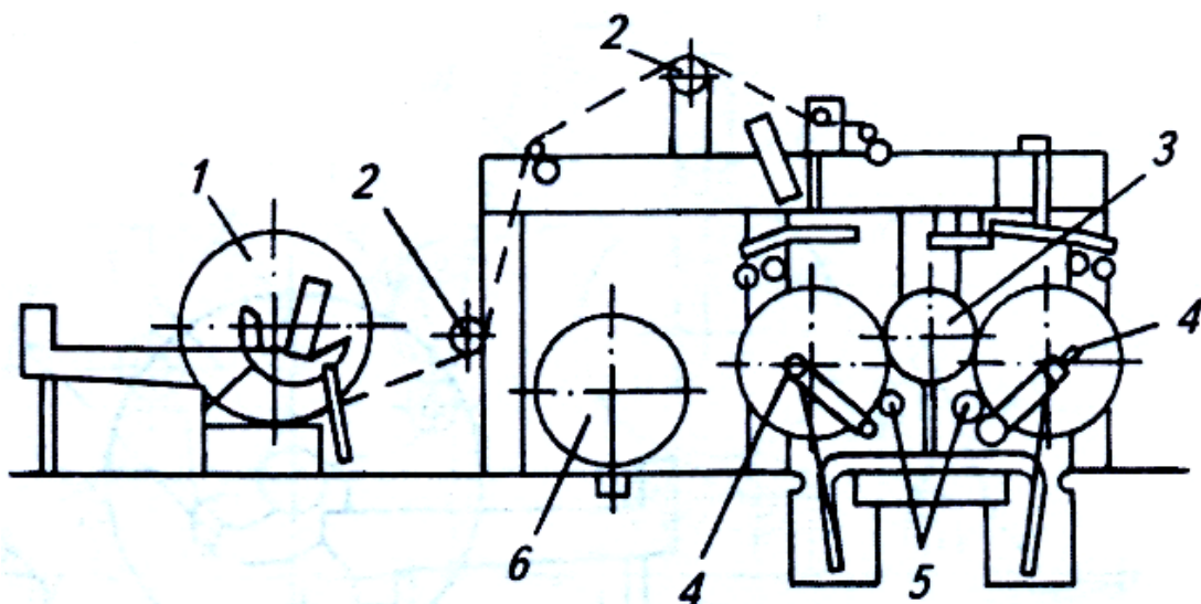
15-рasm. Иккиланган узинасига қирқиш дастгоҳ схемаси:
