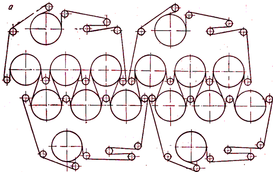
23-расм. Қоғоз қуйиш жихозининг қуритиш қисми
