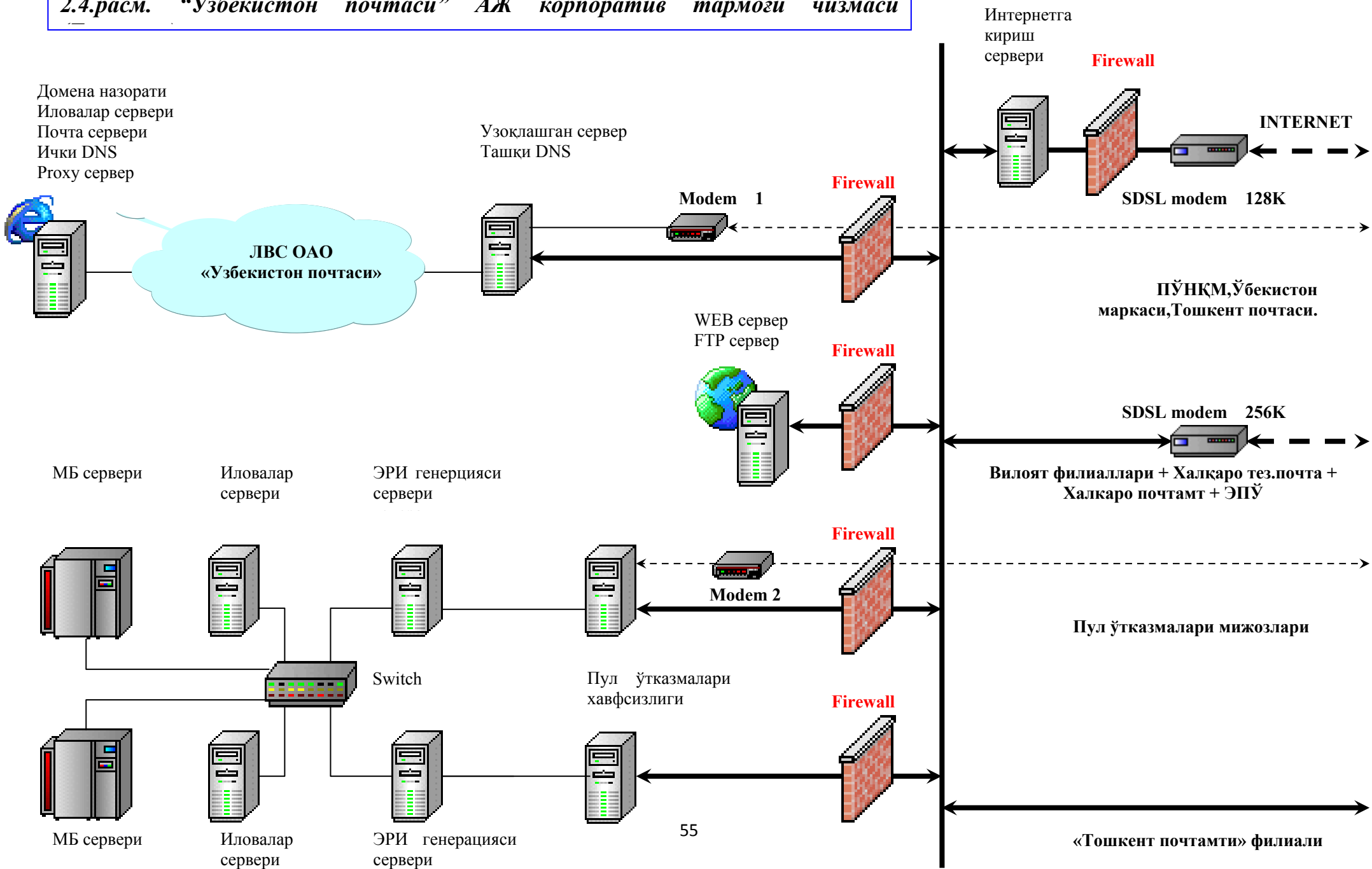
2.4.расм. “Ўзбекистон почтаси” АЖ корпоратив тармоги чизмаси
