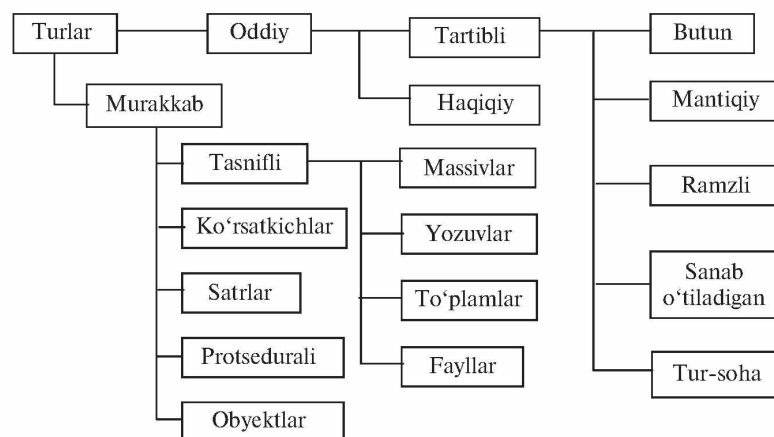
5.1-chizma. Statik ma'lumot turlarining tasnifi.
