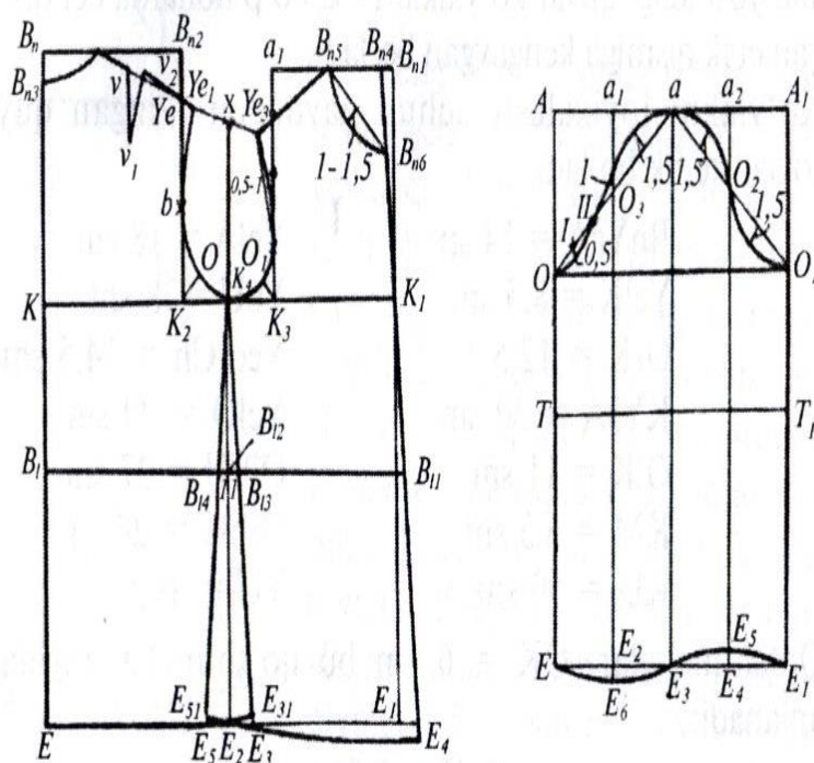
38-rasm. Qiz bolalar ko'ylagi va yengining chizmasi.
