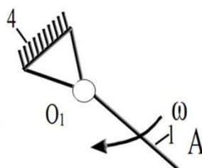
7-расм. O_1 таянч билан кривошипнинг боғланиш схемаси.
