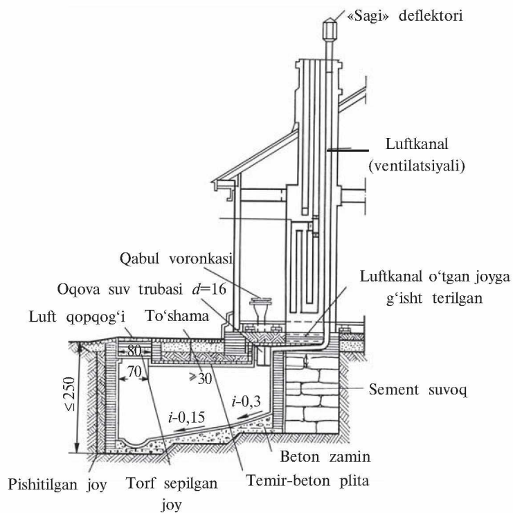
3-rasm. Luftklozet (kesmasi).
