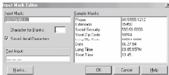
4.17-rasm. Telefon raqamlarini kiritish uchun niqobni yaratish.
