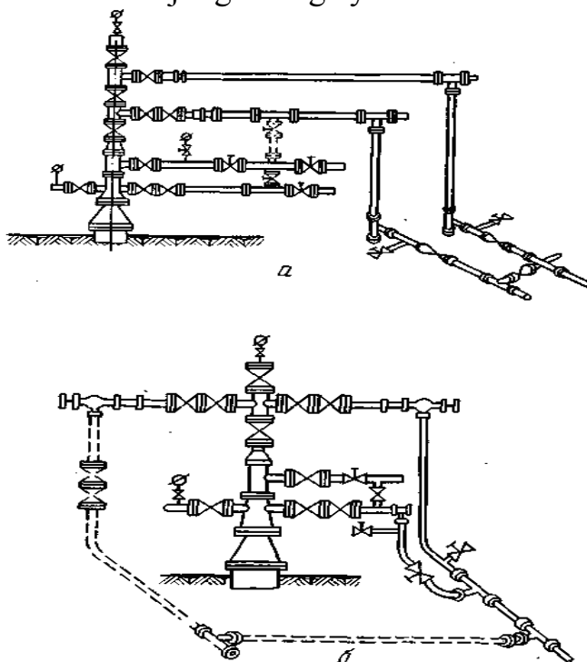
17.4-rasm.a) Ikki qator ko'targich uchun uchlik turidagi favvor armaturasi tarxi. b) Ikki qator ko'targich uchun to'rtlik turidagi favvor armaturasi tarxi
