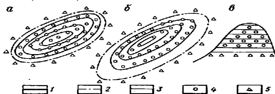
3.1-rasm. Kontur ortidan suv haydash ishlatish tizimi.
