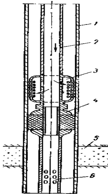
13.4-rasm. Qatlamni gidravlik yorishda er osti jixozlarining joylashish tarxi.
