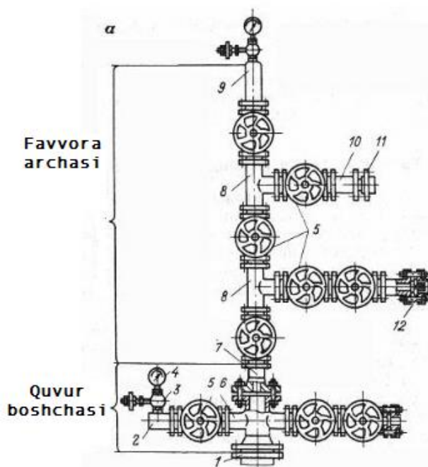
17.2-rasm: Sinash bosimi 250 kg/sm 2 bo'lgan ikki qatorli ko'targichlar uchun uchlik turidagi flansli favvora armaturasi.
