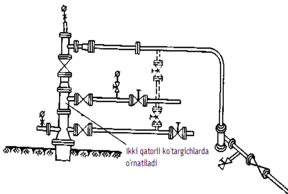
21-rasm. Kompressor qudug'i usti jixozlanish tarxi.
