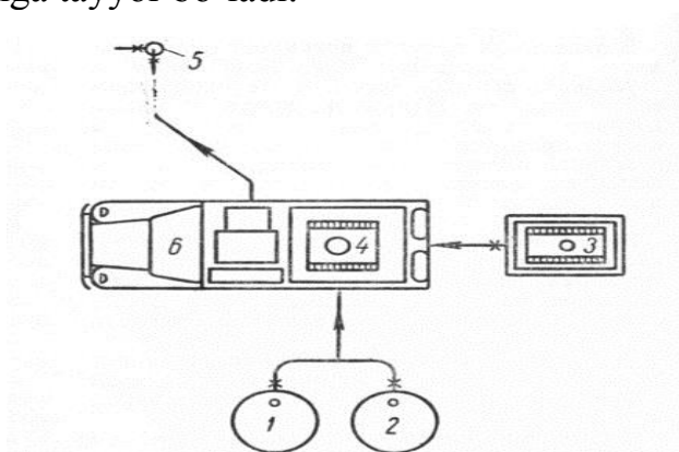
13.1-rasm: Oddiy ishlov berishda jixozlarni joylashish tarxi: 1- Azinmash nasos agregati; 2-Agregatga o'rnatilgan kislota idishi; 3-Tirkamaga o'rnatilgan kislotali idish; 4-Kislota uchun idish; 5-Bostiruvchi suyuqlik uchun idish; 6-Quduq usti.
