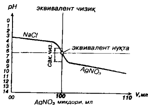
39-расм. NaCl нинг 0,1 н эритмасини AgNO_3 нинг 0,1 н эритмаси билан титрлаш эгри чизиги
