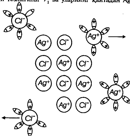
14-расм. \text{AgCl} нинг чўкма ҳосил қилиш схемаси.
