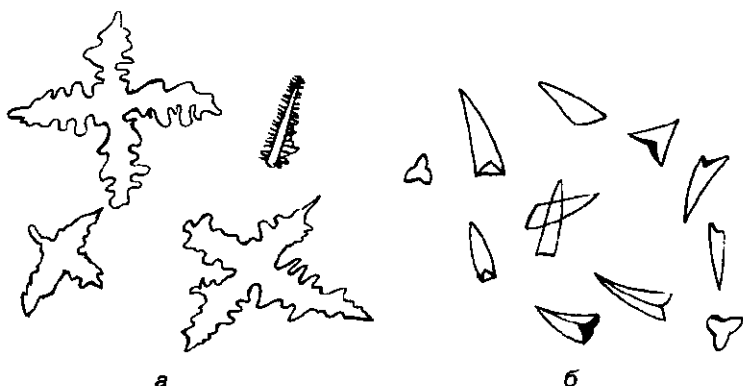
18-расм. а — \text{Zn}[\text{Hg}(\text{CNS})_4] кристаллари, сирка кислотали муҳитда ҳосил бўлган кристаллар б — \text{Zn}[\text{Hg}(\text{CNS})_4] кристаллари, минерал кислотали муҳитда ҳосил бўлган кристаллар.
