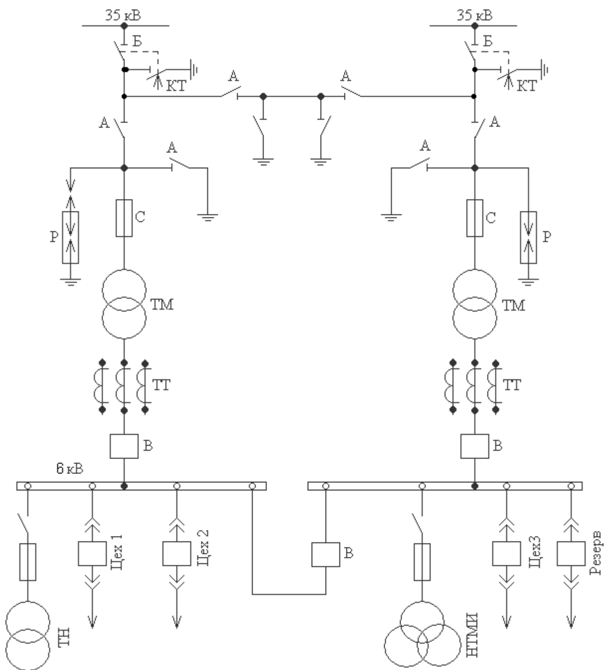
7-расм.Подтанцияни бир чизиқли схемаси
