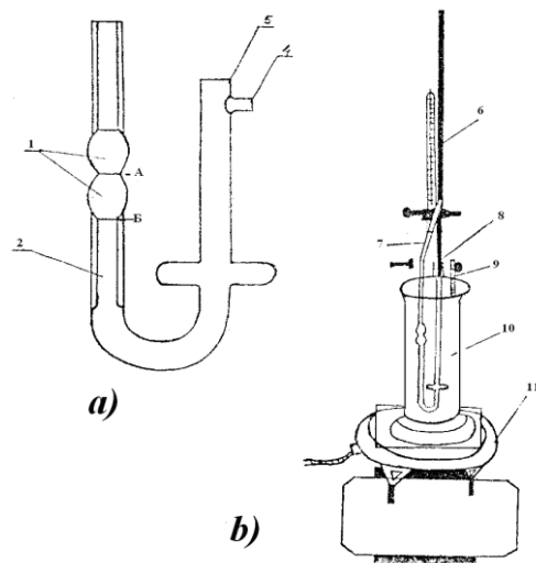
3-rasm. Ostvol d- 'inkevich viskozimetri.
