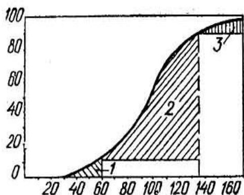
2.5-rasm. Benzinning fraktsion tarkibi: 1-yurgizish fraksiyasi; 2-ishchi fraksiya; 3- og'ir fraksiya
