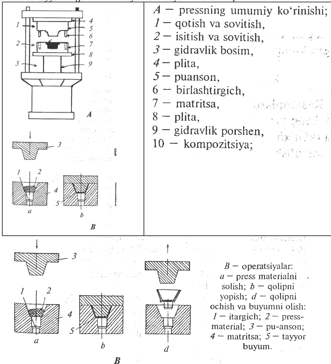
6-rasm. Com'ression 'resslash o'ratsiyalari sxemasi
