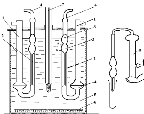
7-rasm. Suvli termostatga o'rnatilgan viskozimetrni umumiy ko'rinishi.
