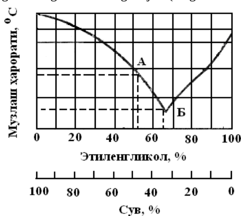
10-rasm 'ast haroratda muzlaydigan etilin glikolli suyuqlik larning muzlash haroratini etilenglikol tarkibiga boglash grafigi
