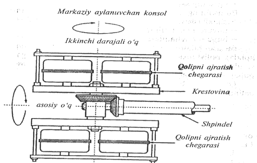
7- rasm. Ikki uqli rotatsion shakllash moslamasi.
