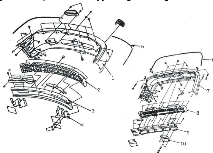
3.8-rasm. NEXIA avtomobilining oldi va orqa bamperlari:
