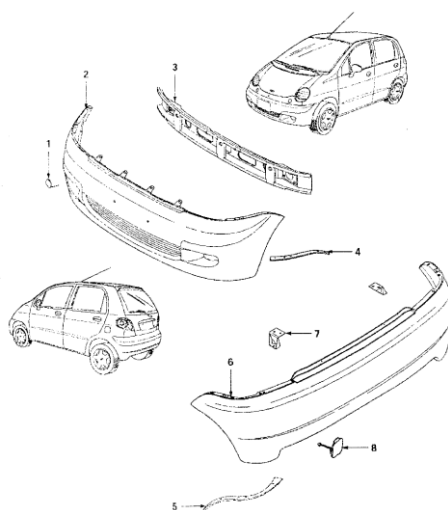
3.7-rasm. MATIZ avtomobilining oldi va orqa bamperlari
