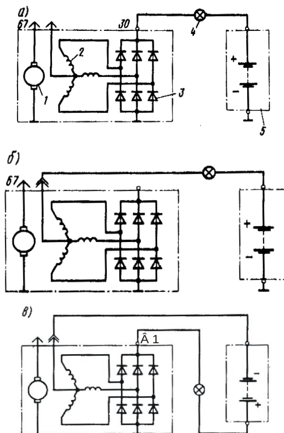
3.4-rasm. To'g'rilagich diodlarini tekshirish sxemasi.
