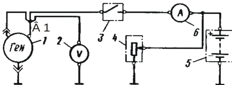
3.5-rasm. Generatorni tekshirish sxemasi.
