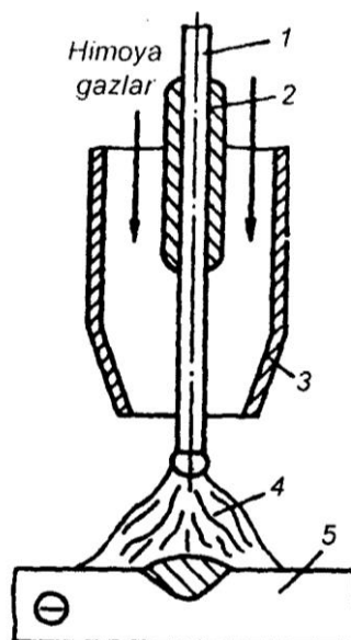
4.2-rasm. Eriydiganelektrodbilanhimoyagazlarmuhitida payvandlashjarayoniningchizmasi:
