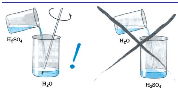
45-сүрөт. Сульфат кислотасынын эритмесин даярдоо
