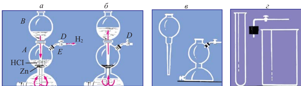
26-сүрөт. Кипп аппаратынын курамдык бөлүктөрү жана аппаратын иштеши (а,б,в), анын ордун басуучу атайын прибор (г).
