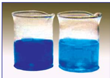
32-сүрөт. Туздар (а) жана алардын эритмелери (б)
