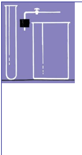
44-сүрөт. Сульфат кислотасынын жыгачка тийгизген таасири
