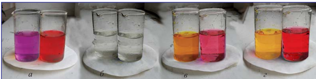
24-сүрөт. Кислоталардын эритмелеринин индикаторлорго тийгизген таасири:
