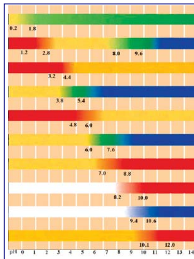
51-сүрөт. Индикаторлордун көрсөткүчтөрү
