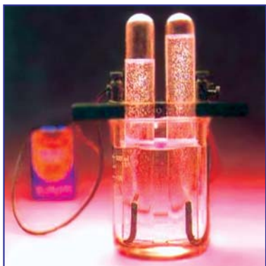
18-сүрөт. Суунун электролизинде 2 көлөм суутек жана 1 көлөм кычкылтек алынат
