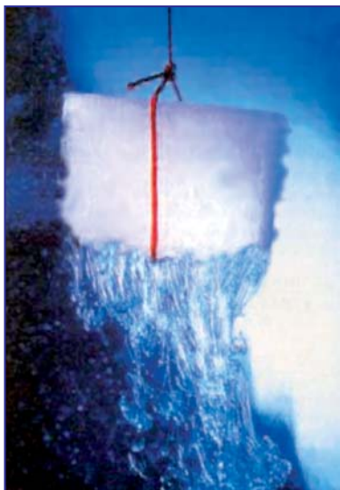
30-сүрөт. Канттын сууда эриши
