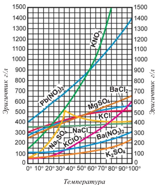
31-сүрөт. Ар түрдүү туздардын эригичтигинин ийри сызыктары
