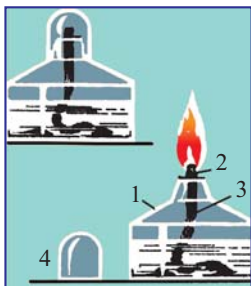
4-сүрөт. Спиртовка
