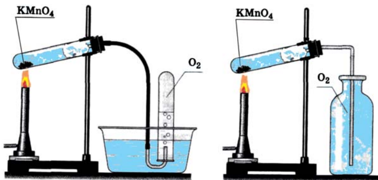
22-сүрөт. Кычкылтек алуу үчүн даярдалган аспап.
