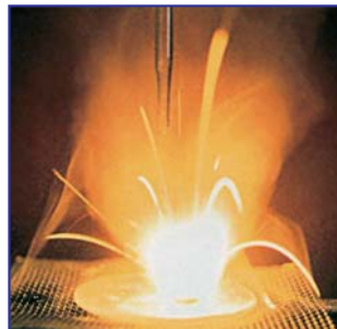
40-сүрөт. Na га суунун таасири
