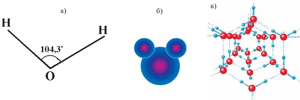
27-сүрөт. Суунун графикалык (а), көлөмдүк түзүлүшү (б) жана ассоциациялык абалы (в).
