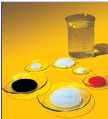
29-сүрөт. Ар түрдүү заттардын сууда эриген салыштырмалуу сандары:
