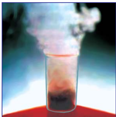
19-сүрөт. H_2O_2 ин MnO_2 нин катышуусунда ажырашы
