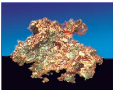
36-сүрөт. Табигый жездин бөлүгү
