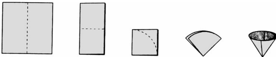
12-сүрөт. Фильтрди даярдоо
