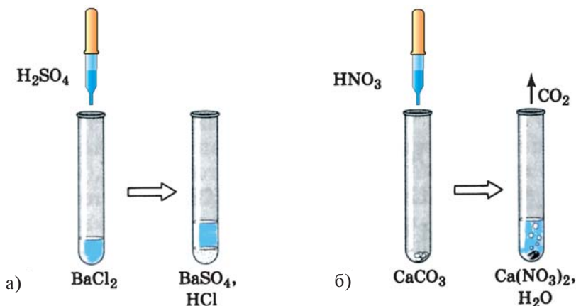
16-сүрөт. Тунманын жана газдын пайда болушу
