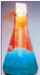
43-сүрөт. Жездин жана башка металлдардын ар түрдүү кислоталар менен таасирдешүүсү
