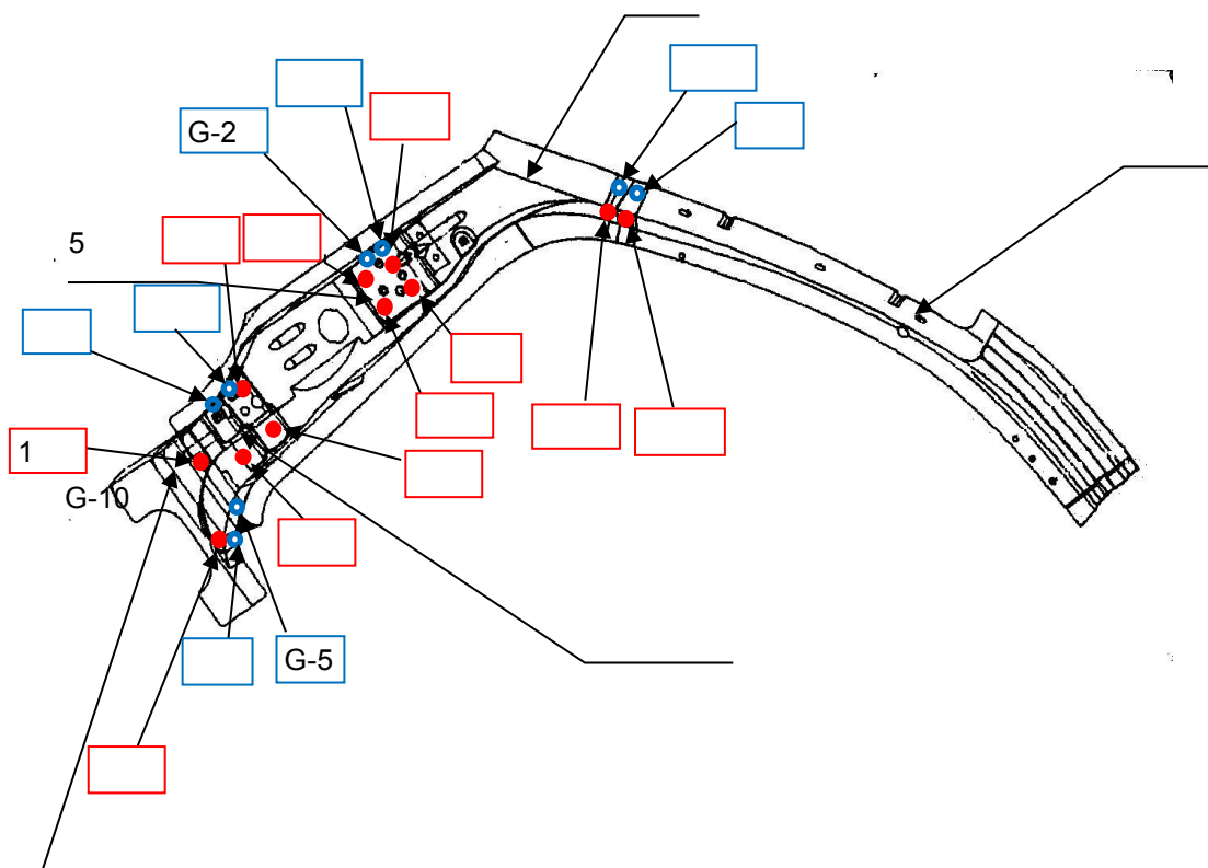
8-расм Матиз автомобилнинг REINF A-FRONT PULLAR, LH / RH панели
