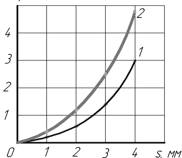
1-расм. Электр энергияси сарфининг материал қалинлигига боғлиқлиги графиги.
