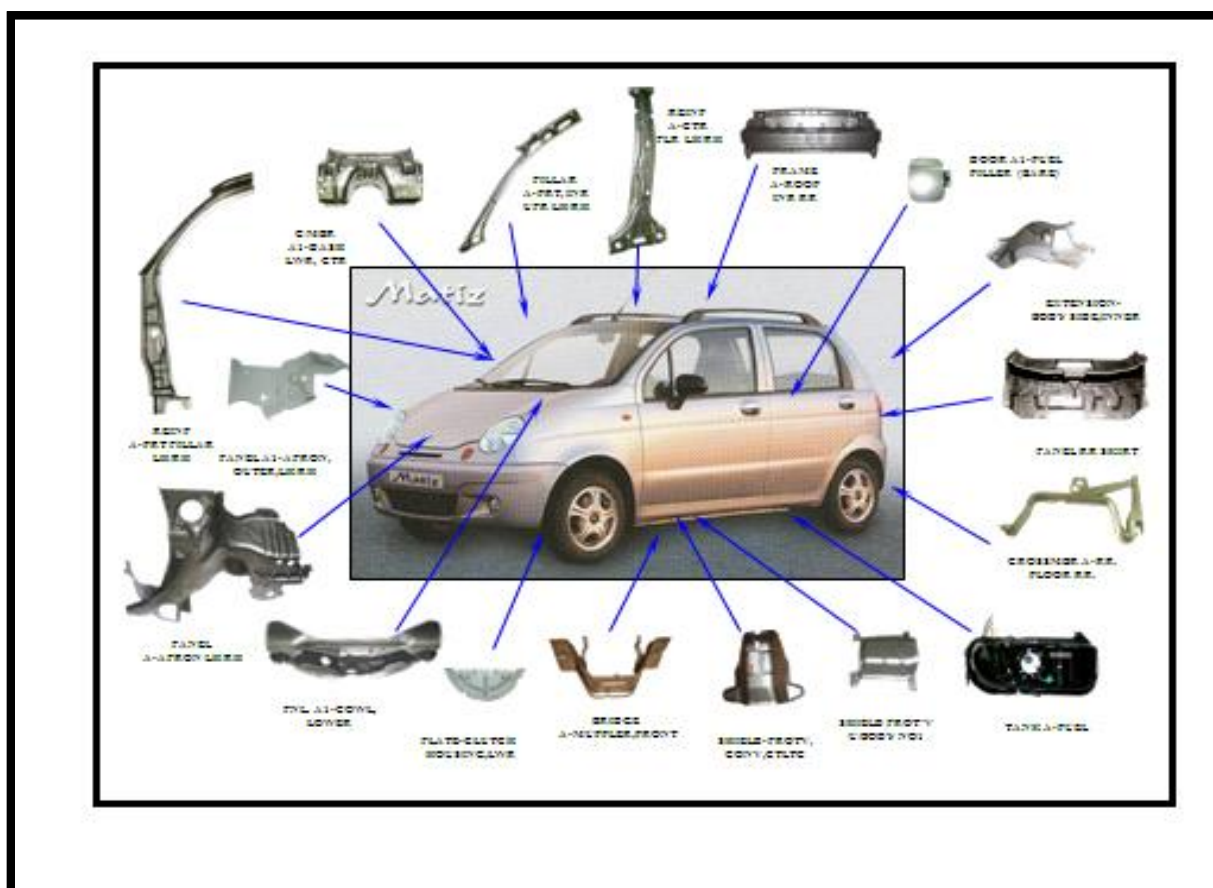
6-расм. Матиз автомобили учун “Uz-SaeMyung Co.” кўшма корхонасида ишлаб чиқариладиган 17 хил панел ишлаб чиқарилади панелларнинг турлари
