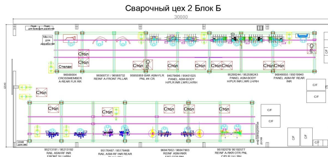
14-расм пайвандлаш сеҳи схемаси.
