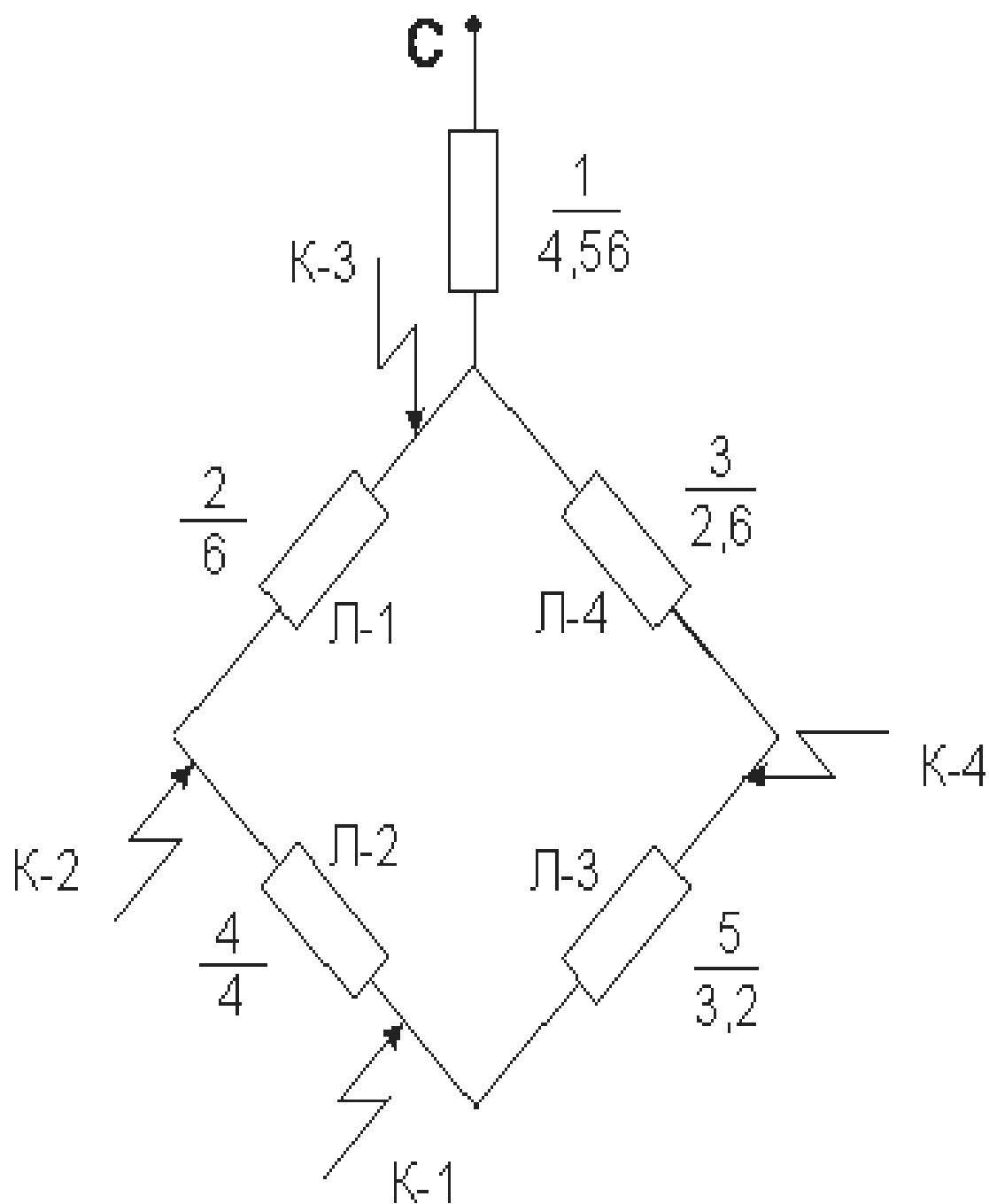
Б) Тармоқнинг алмаштириш схемаси
