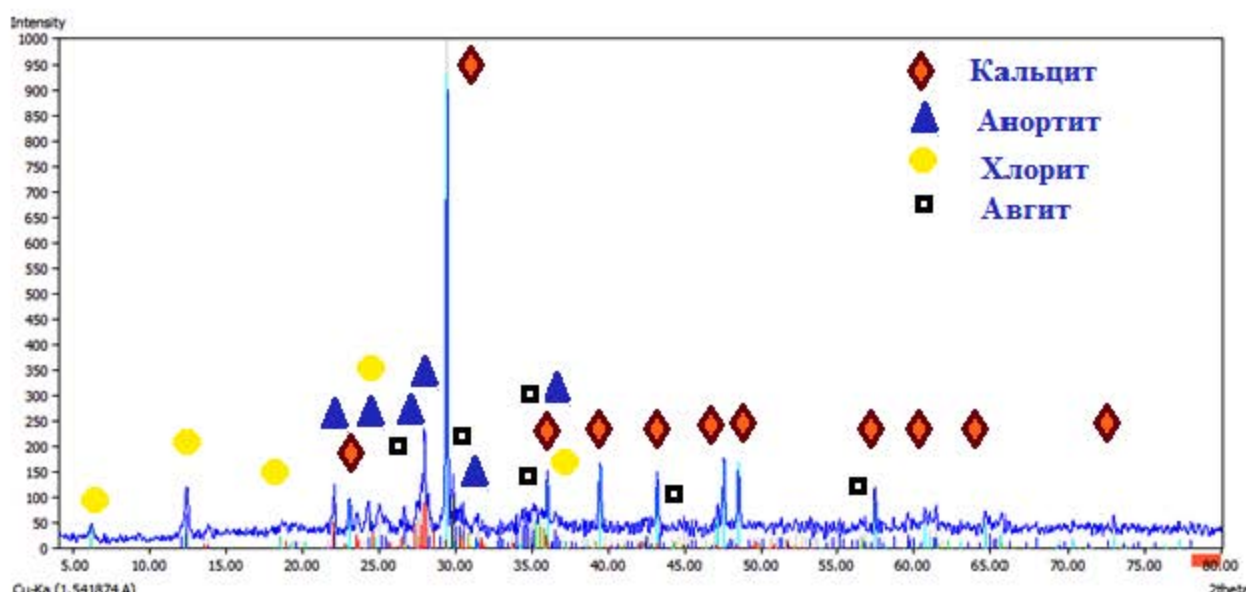
Рис. 2. Рентгенограмма образца базальта участка Каракия.
