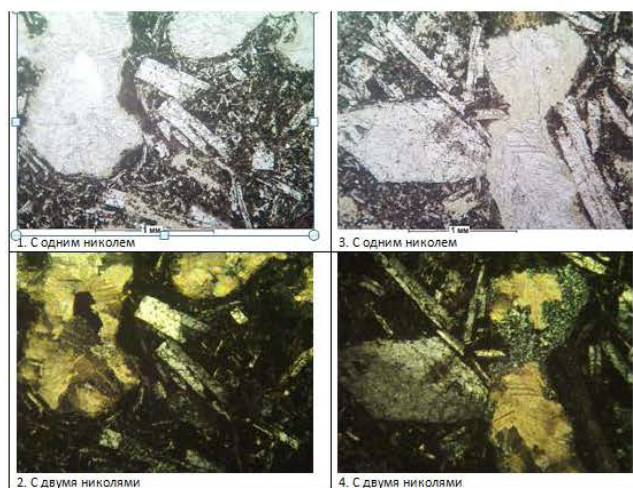
Рисунок 1. Результаты микроскопического исследования базальта: базальт миндалевидный. Порфировые выделения плагиоклаза составляют 2-3, лейсты плагиоклаза (альбита) 7-10, микролиты альбита 20-25, миндалины кальцита 5-7, миндалины хлорита 2-3, роговая обманка базальтическая бурая 2-3, стекло чёрное непрозрачное 50-55, магнетит 1-1,5 мас. %.
