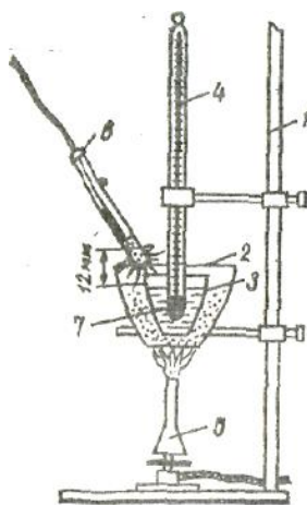
12-раем. Битумсымон материал парнинг ёниш температура-сини аниқлашда . ишлатн.чади-ган асбоб: 1 — штатив, 2 — кумли иситгич, 3 — битум солинган кичик тунука тигель, 4 — термометр. 5 — горелка, 6 — аланга битуми, 7 — битум намуна
