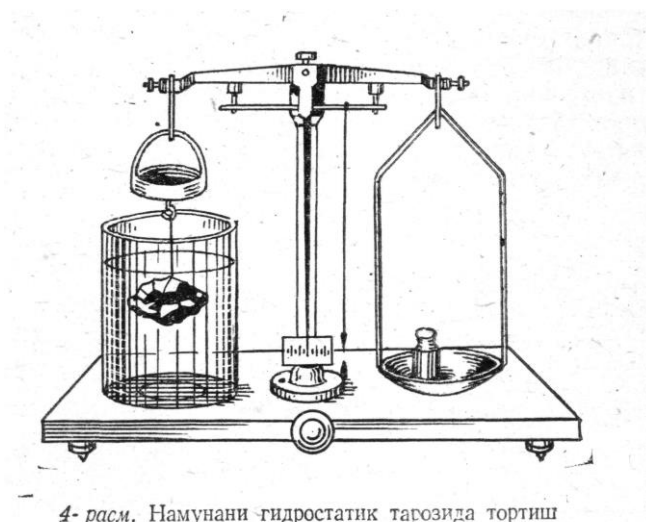
4- расм. Намунани гидростатик тарозида тортиш
