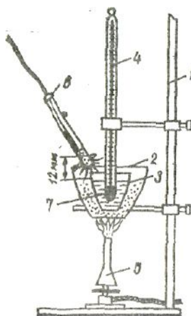
12-раем. Битумсмон материал парнинг ёниш температура-сини аниқлашда . ишлатиладиган асбоб:
