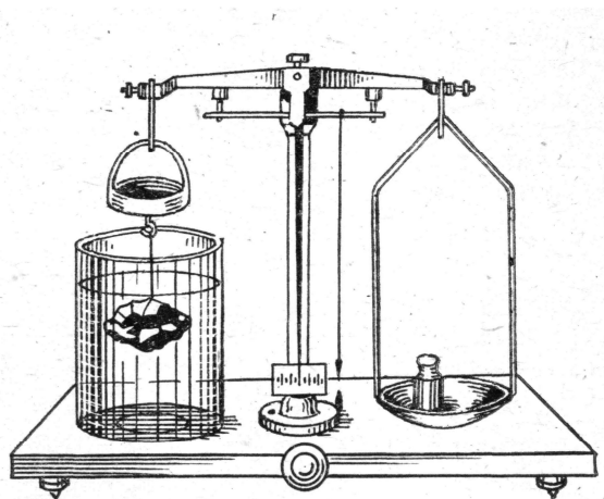
4- расм. Намунани гидростатик тарозида тортиш
