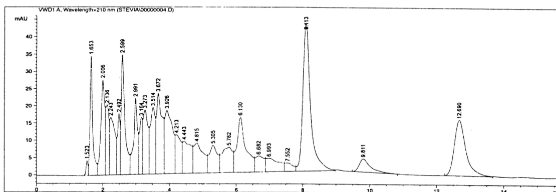
Хроматограмма испытуемого образца жидкого экстракта стевии
