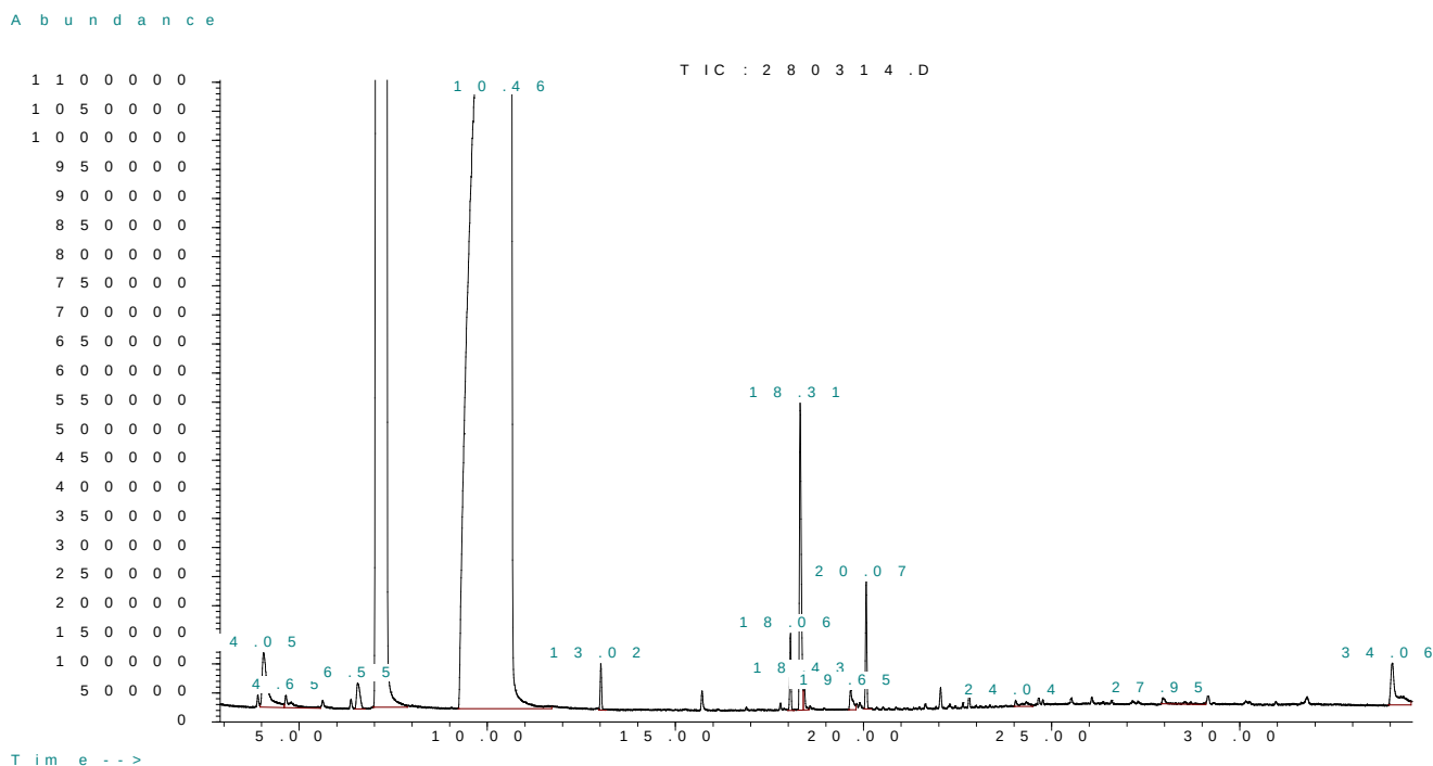
Рисунок. Хроматограмма раствора исследуемого жидкого экстракта “Урглисал”
