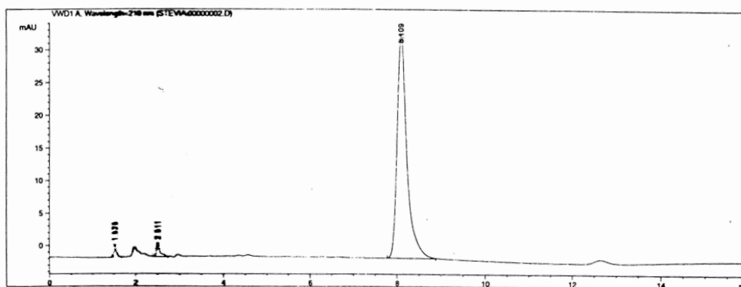
Хроматограмма раствора стандартного образца стевиозида
