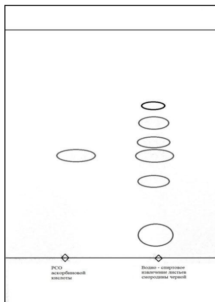
Рис. 1. Схема тонкослойной хроматограммы извлечения из листьев смородины черной.
