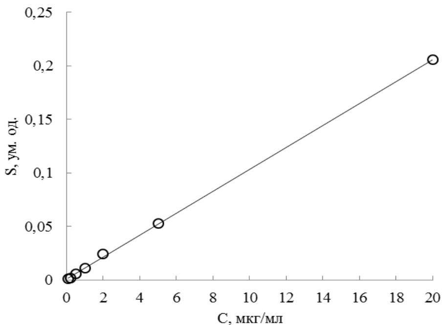
Рис. Графік градувальної залежності площі піку метанольного розчину глібенкламід у від концентрації
