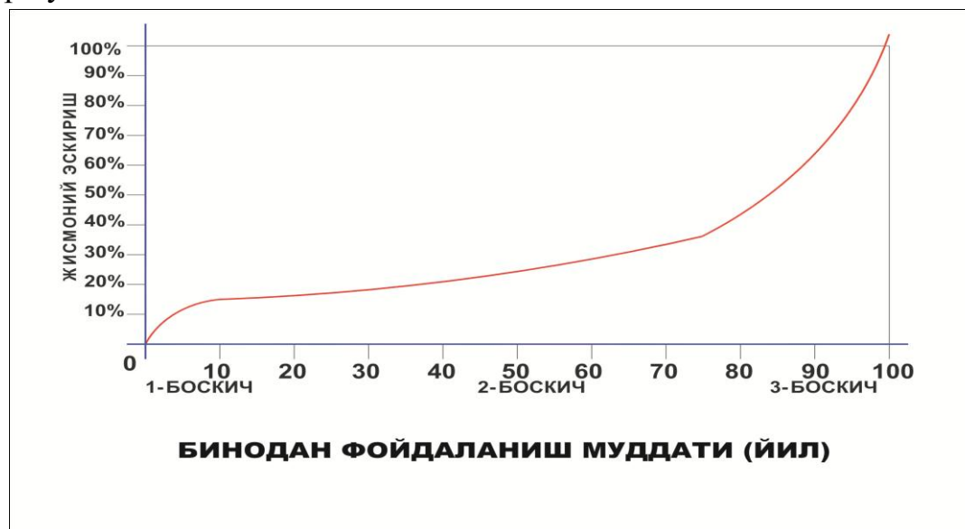
4-расм. Бинода жисмоний эскириши даражасининг ривожланиши. 10
