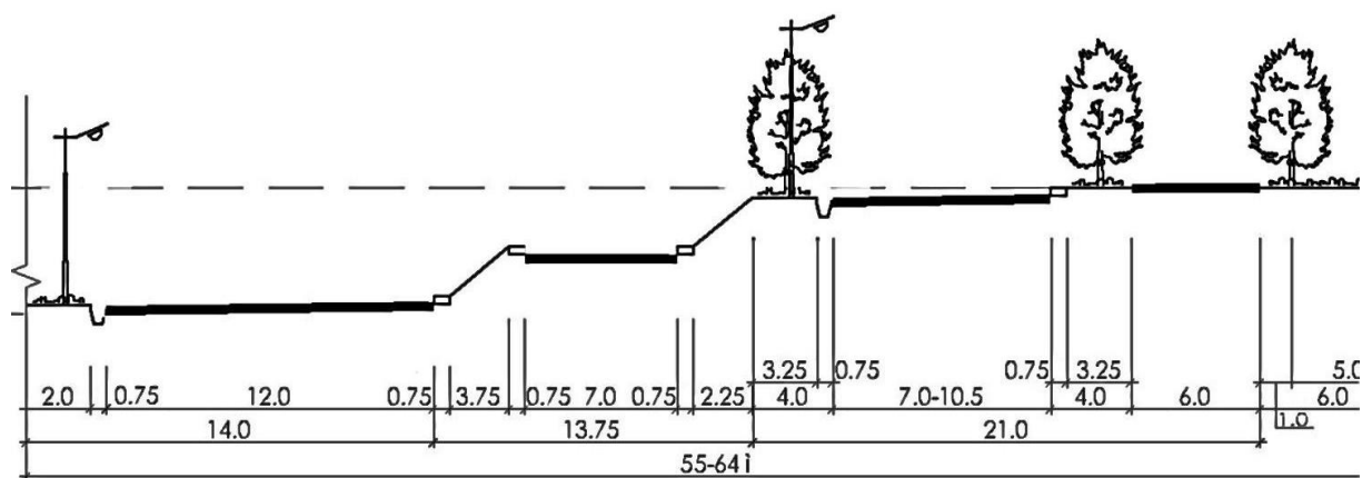
3.3-расм. Турли сатҳларда лойиҳаланган шаҳар тезкор йўллارининг кўндаланг кесими (йўлнинг ярми кўрсатилган).
