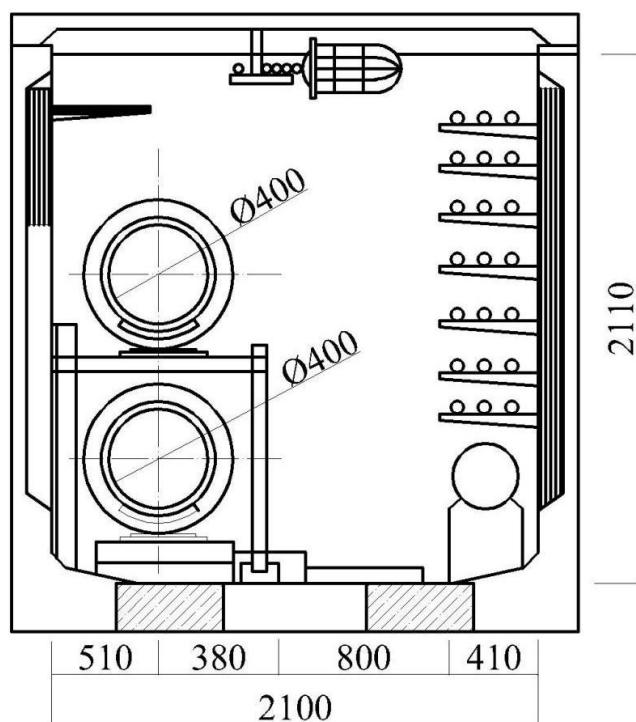
2.10 - расм. Йиғма темир бетонли коллектор
