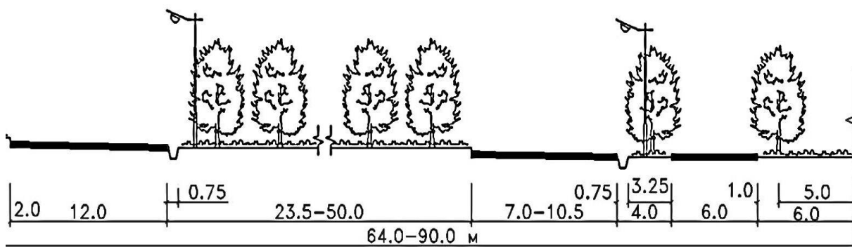
3.2-расм. 1 сатҳли шаҳар тезкор йўллари кўндаланг кесими (йўлнинг ярми кўрсатилган).
