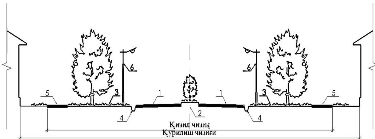
3.1- расм. Кўчаэлементлари:
