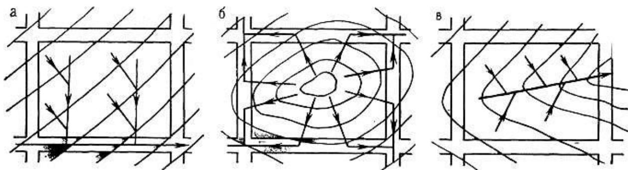
2.13-расм. Турар-жой масканлари худудида оқова сув тармоқларини ташкиллаштириш шакллари.
