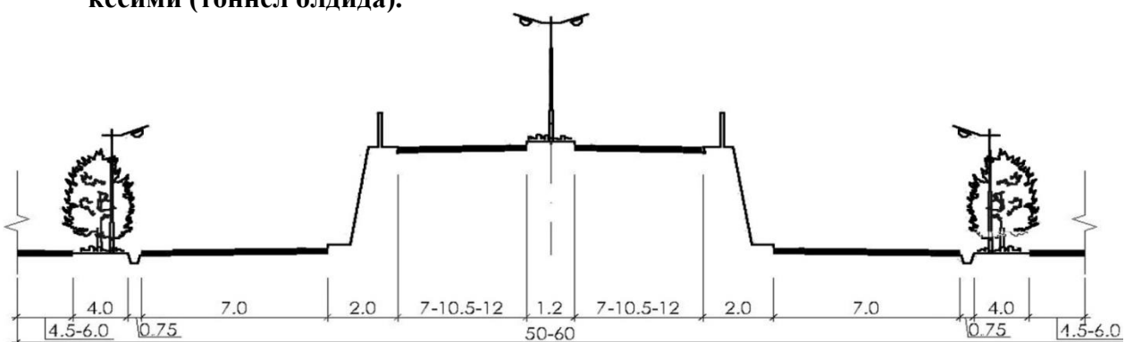
3.4-расм. Ҳаракати узлуксиз шаҳар магистрал кўчаларининг кўндаланг кесими (тоннел олдида).
