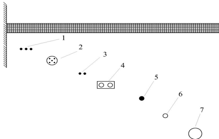
2.6–расм. Ер ости муҳандислик тармоқларининг бино пойдевори тарафидан кўчанинг ўқ чизигига қараб поғонама-поғона чуқурлашиб бориш тартиби.
