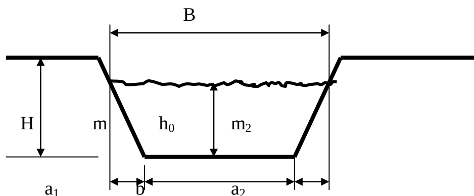
2.15- расм. Трапециякўринишидаги ариқкўндаланг кесимининг юзаси.
