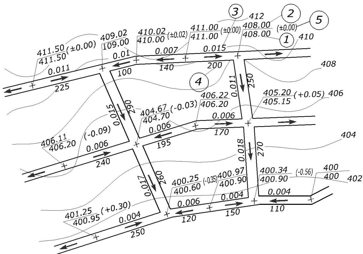
1.3-расм. Шаҳар ҳудудини вертикал режалаштириш схемалари фрагменти
