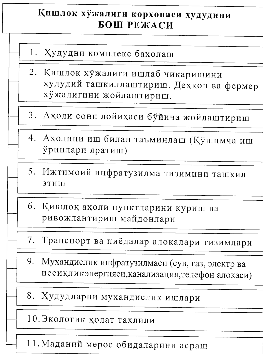
1.2-расм. ҚМК 2.07.04-06га мувофиқ Бош архитектуравий-лойиҳани асослашнинг 1-босқичи
