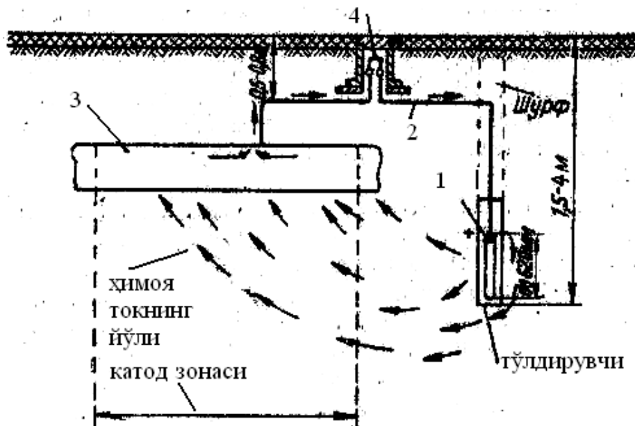
Протектор химояси схемаси . 1-анод; 2-кабель; 3-газ қуури; 4-назорат пункти.
