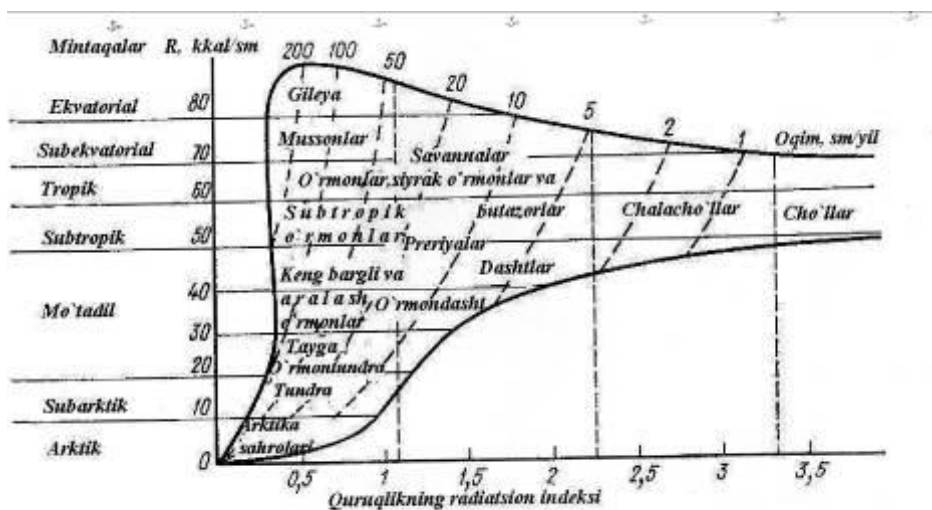
2 - chizma. Shimoliy yarim sharda quruqlik geografik zonalligining grafigi (A.A.Grigoryev va M.I.Budiko, 1956)
