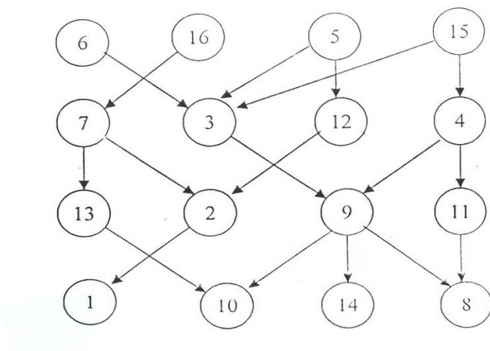
Рис. 4.10. Ярусный граф заданного набора задач
