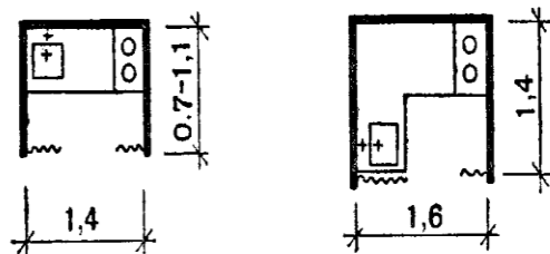
91-расм. Ошхона- тахмоннинг тархий ечимига доир мисол.
