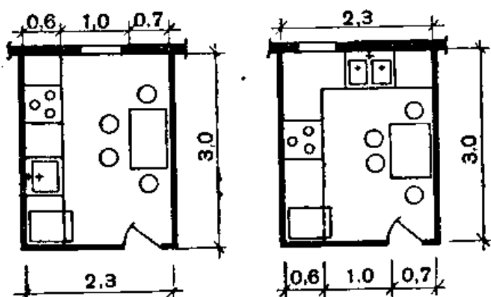
92 расм. Ошхона-ошхонанинг тархйй ечимига доир мисол.
