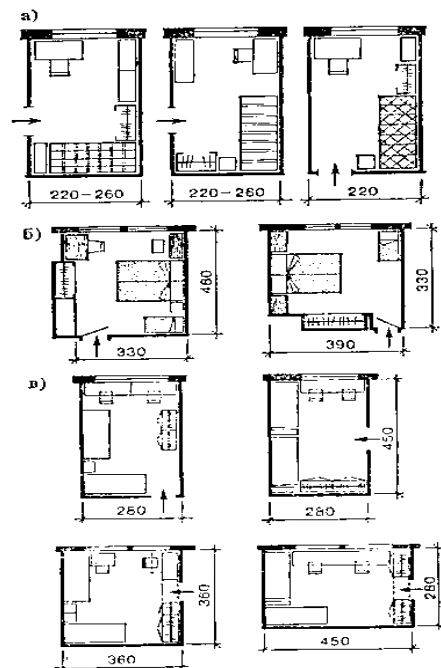
Хоналарнинг ўлчамлари ва нисбатларига боғлиқ равишда ётоқхоналарни ташкил этиш вариантлари: А- бир киши учун, Б- ота-оналар учун, В – ўрта ёшдаги иккита бола учун.
