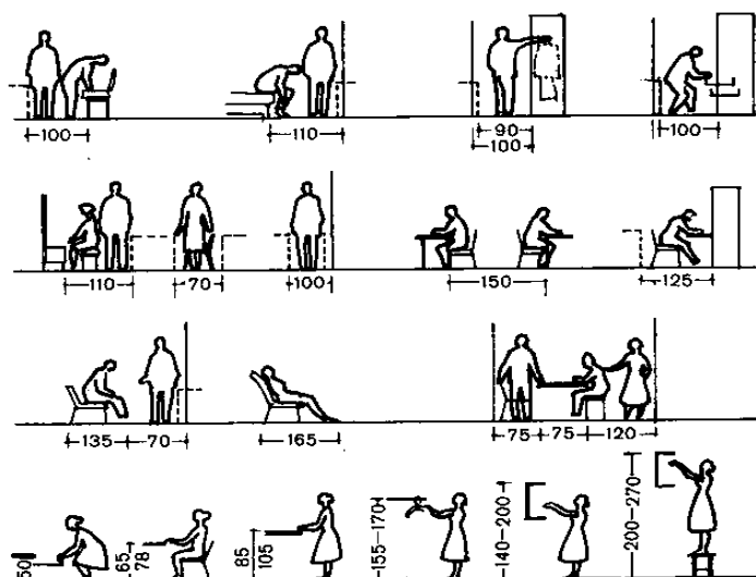
71 - расм. Турар-жой ячейкасининг фазовий ташкил этилиши. Қурилманинг юқори ўтиш ва юқори элементлари габаритлари.
