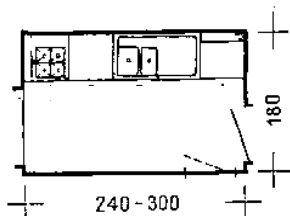
89 расм. Ошхона жиҳо-зини бир қатор қилиб жойлаштиришга
