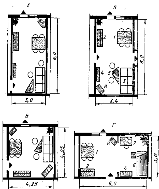
77 расм. Ҳар хил габаритли мебельларни умумий хона ва ошхонага жойлаштириш
