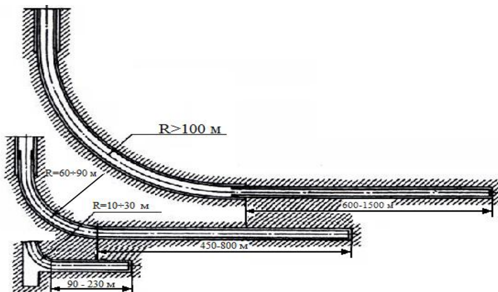
2.-расм.Горизонталкудукникатта ( R > 190 \text{ m} ), ўрта ( R = 60-90 \text{ m} ) вакичик ( R = 10-30 \text{ m} ) бурилишрадиусларибиланбурғилашсхемаси.
