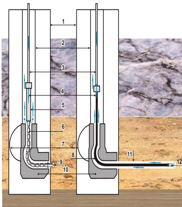
3.2-рasm. Қатламни радиал очиш схемаси
