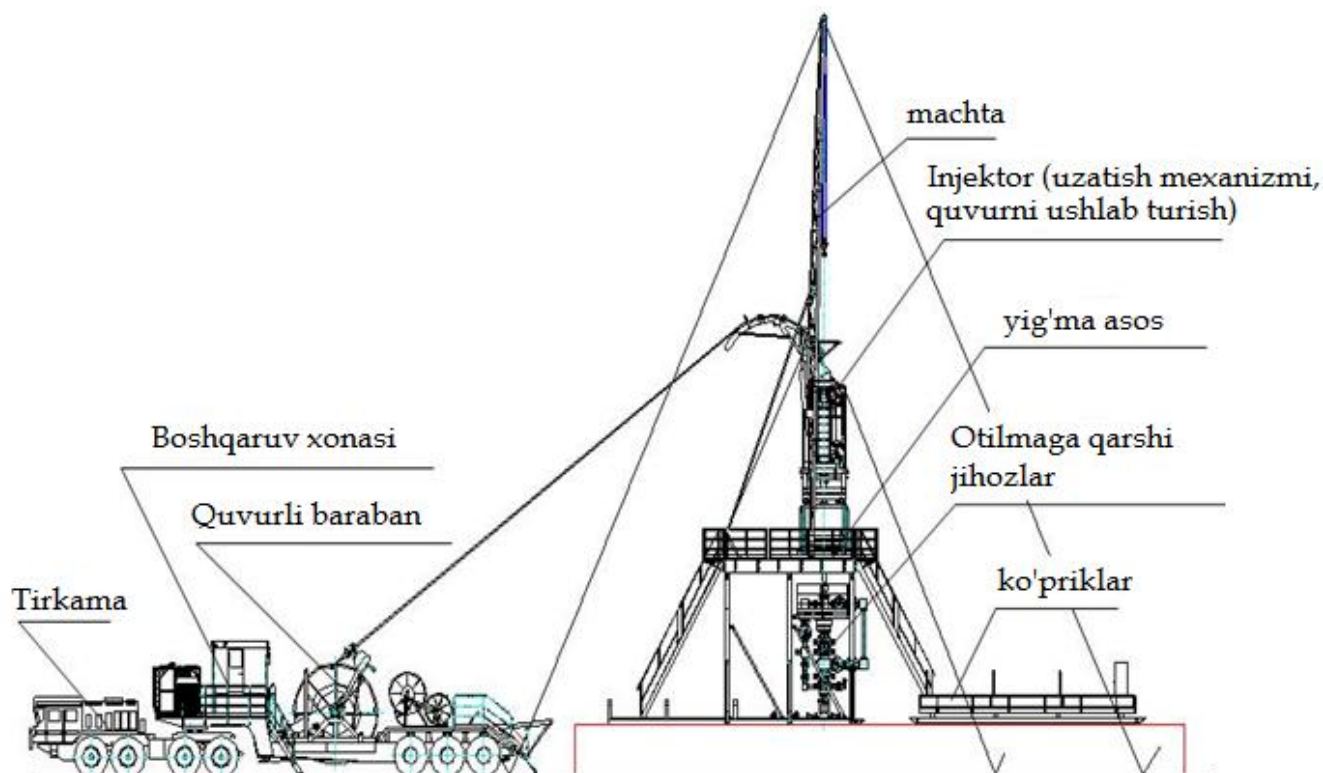
3.10-расм. Колтюринг қурилмасининг умумий кўриниши
