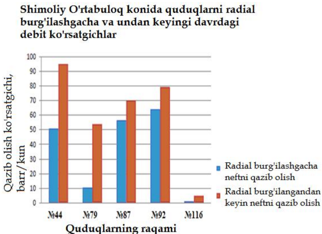
3.14-расм. Радиал бурғиланган қудуқларнинг кўрсаткичларини таққослаш диаграммаси
