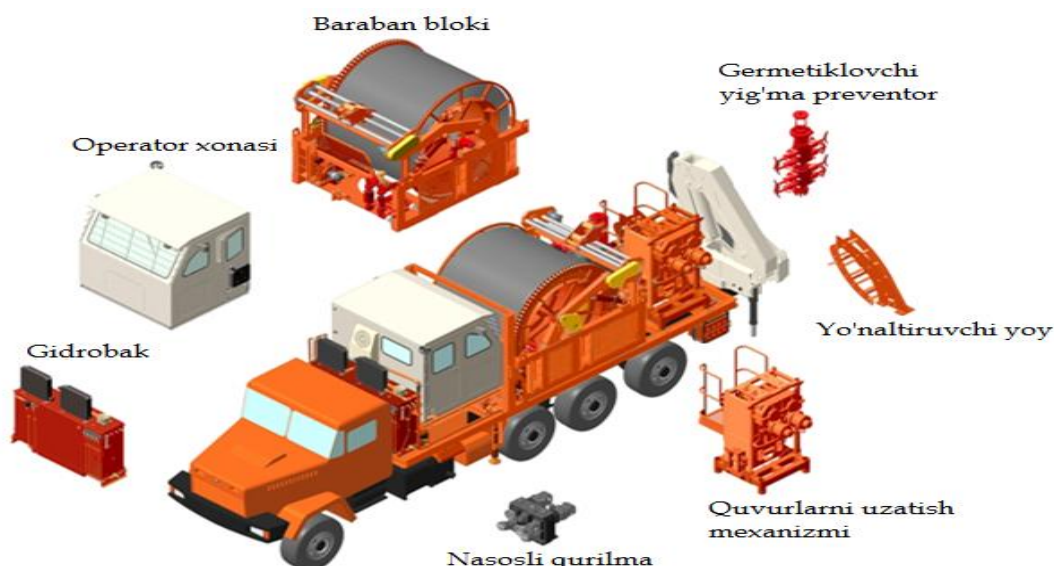
3.8 –расм. Махсус колтюбинг жамланмасининг умумий кўриниши
