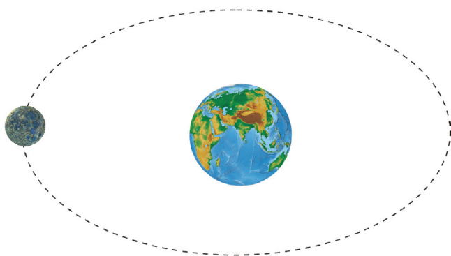
9-su'wret. Aydi'n' Jer a'tirapi'nda aylani'wi'.
