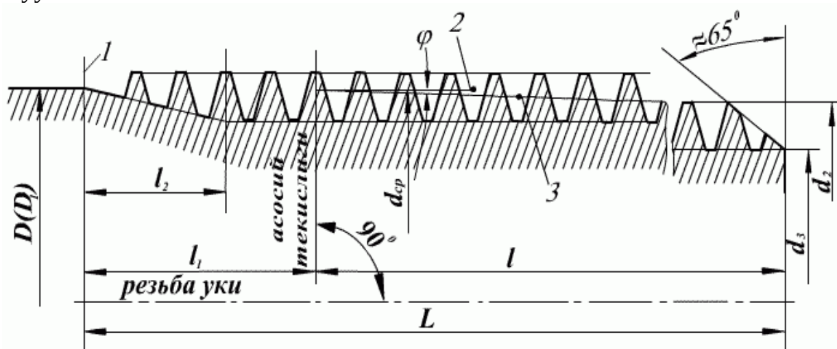
24-рasm. 1 va 2 turidagi burg‘ilash quvurlari uchburchak konussimon rezbalari kesimining o‘lchamlari.
