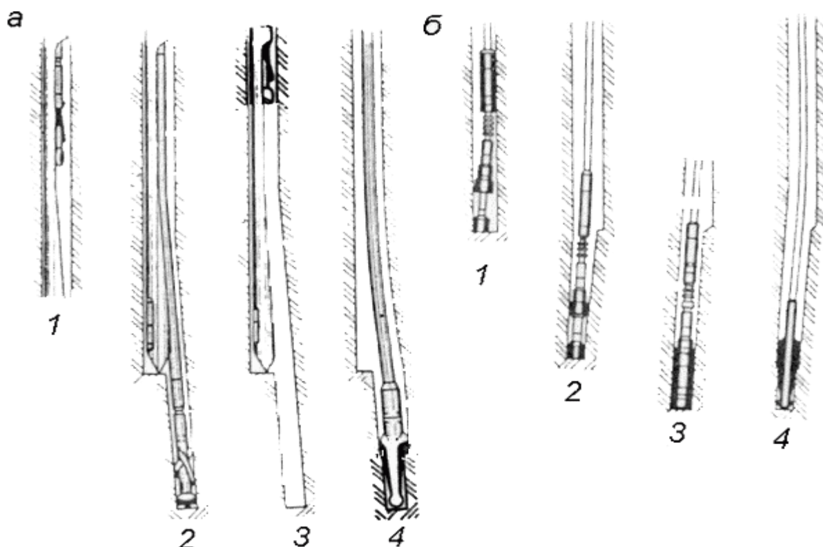
50-rasm. Rotor usulida qiya yo'naltirilgan quduqlarni burg'lashda qo'llaniladigan qiyalantiruvchi moslamalar.
