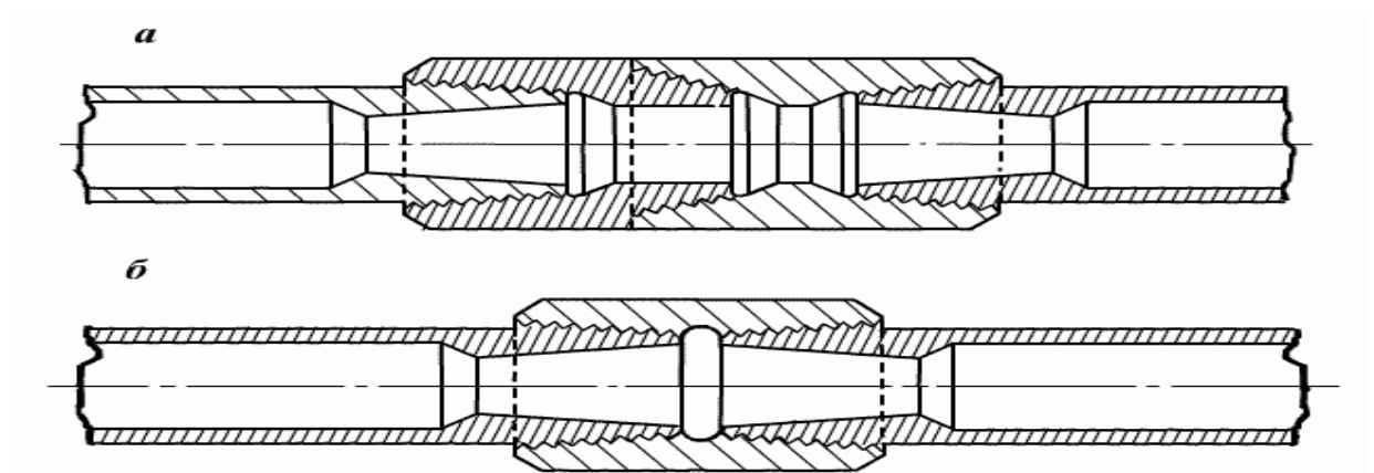
25-rasm. Yakunlari chiqarilgan burg'ilash quvurlarining bog'lanishi.
