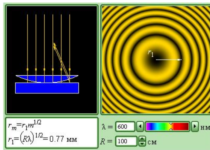
8-rasm. Nyuton halqasi.
