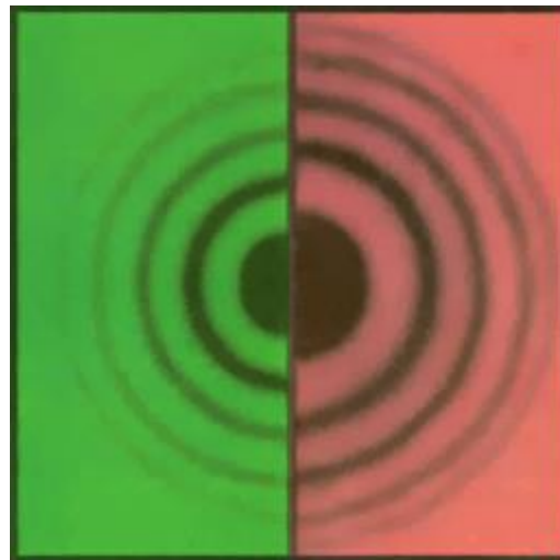
4-rasm. Nyuton halqalarining yashil va qizil nurlarda hosil bo'lishi.
