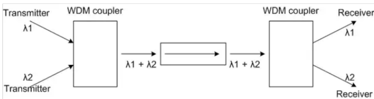
Рис.12.1. WDM мультиплексирование
