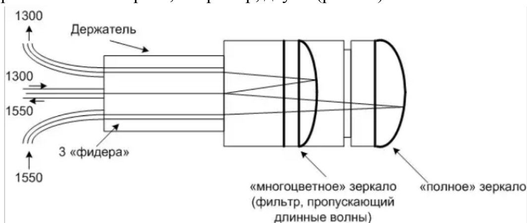
Рис.12.5. SCR-каплер с двумя зеркалами
