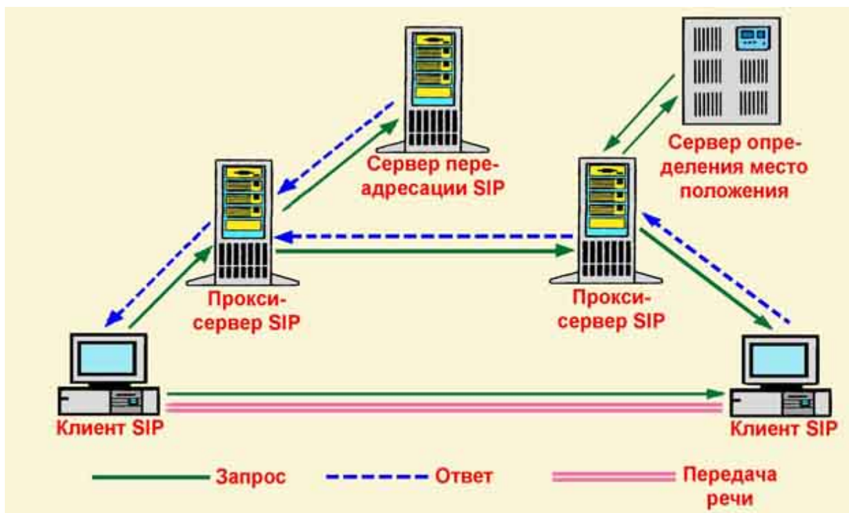
Рис.2.2. Архитектура SIP сети
