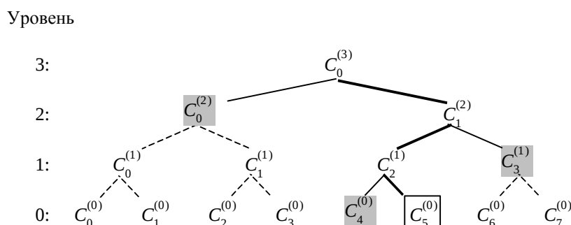
Рис. 4.1. Двоичное дерево для схемы ЭЦП на 8 сообщений
