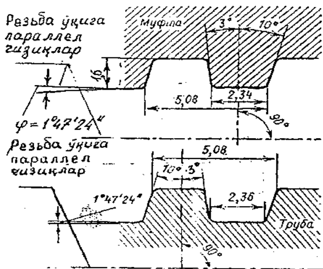
7-расм. Россия стандарти бўйича трапецеидал резьба профили
