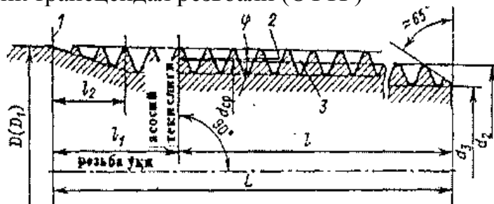
6-расм. Конуссимон учбурчакли резьба профилининг катталиклари.
