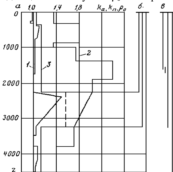
4- расм. k_a аномаллик коэффициентини ва k_n босим индексининг ўзгартириш характери графиги
