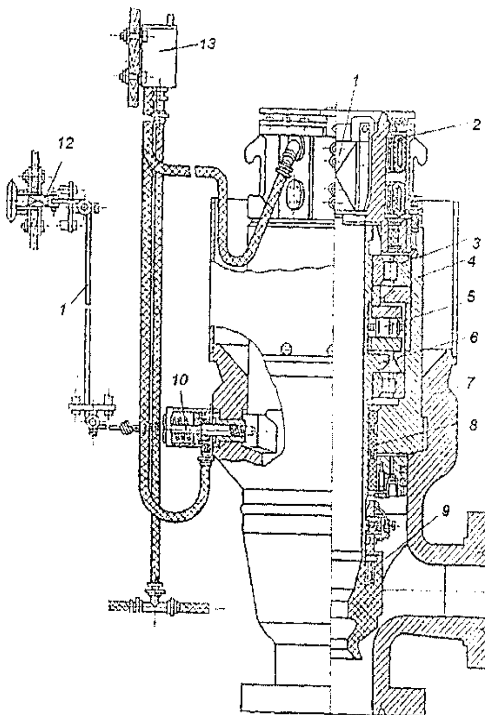
24- расм. Айлантурувчи превентор.
