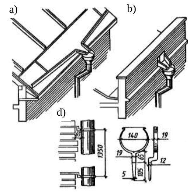
2.66-rasm. Yog'in-sochin suvlarini oqizib yuborishga mo'ljallangan tarnovlar:
