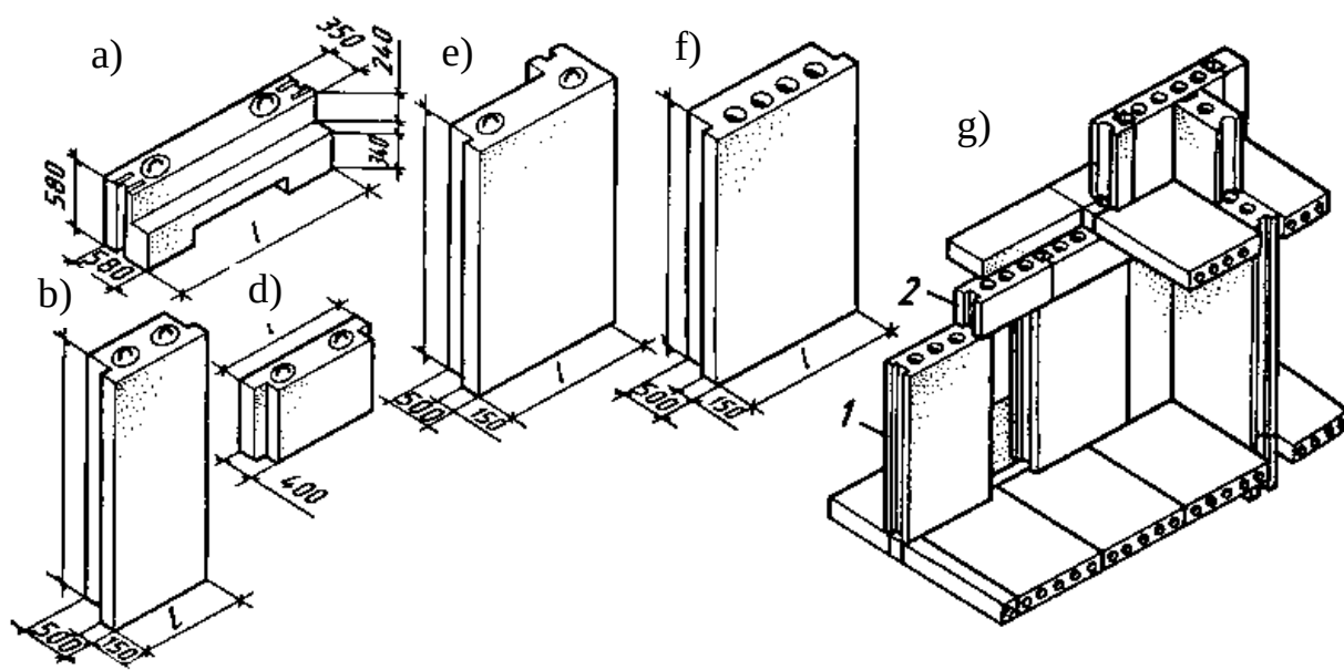
2.77-rasm. Turar-joy binolarida ishlatiladigan yirik bloklar turlari:
