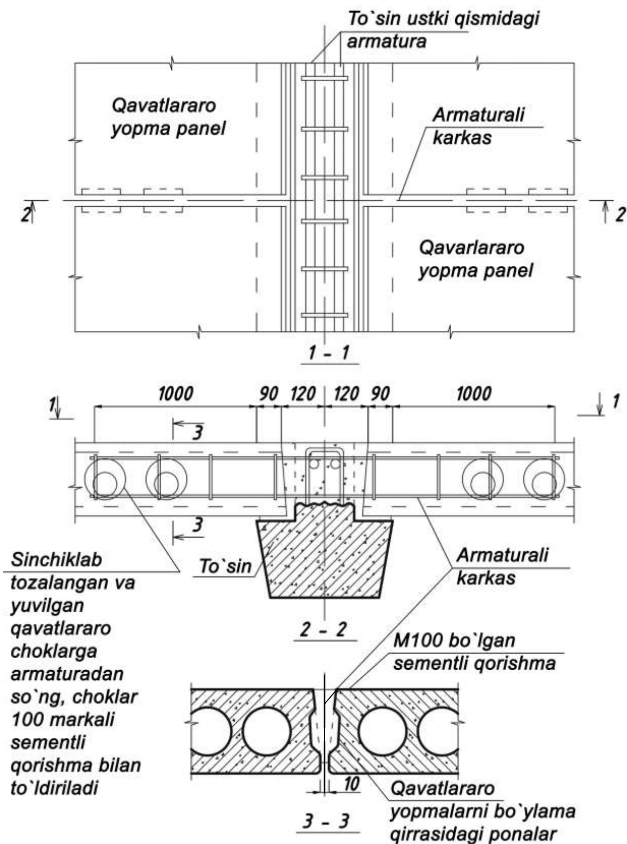
3.17-rasm. Qavatlararo yopmalar orasidagi choklarini quyma beton bilan to'ldirish.
