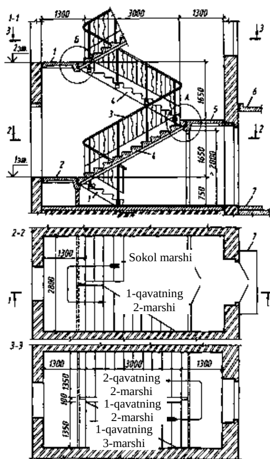
2.72-rasm. Ikki marshli zina:
