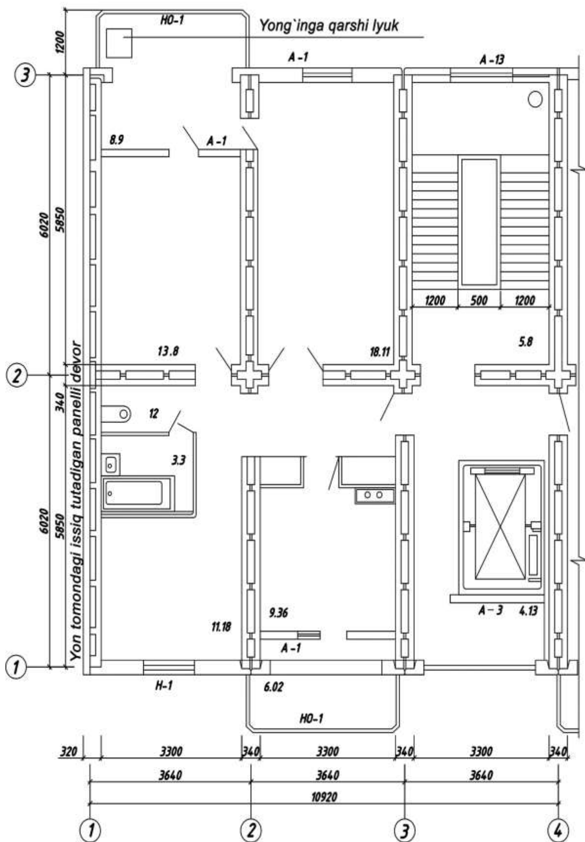
5.4-rasm. Blok-seksiyaning namunaviy qavatining element tarxi.
