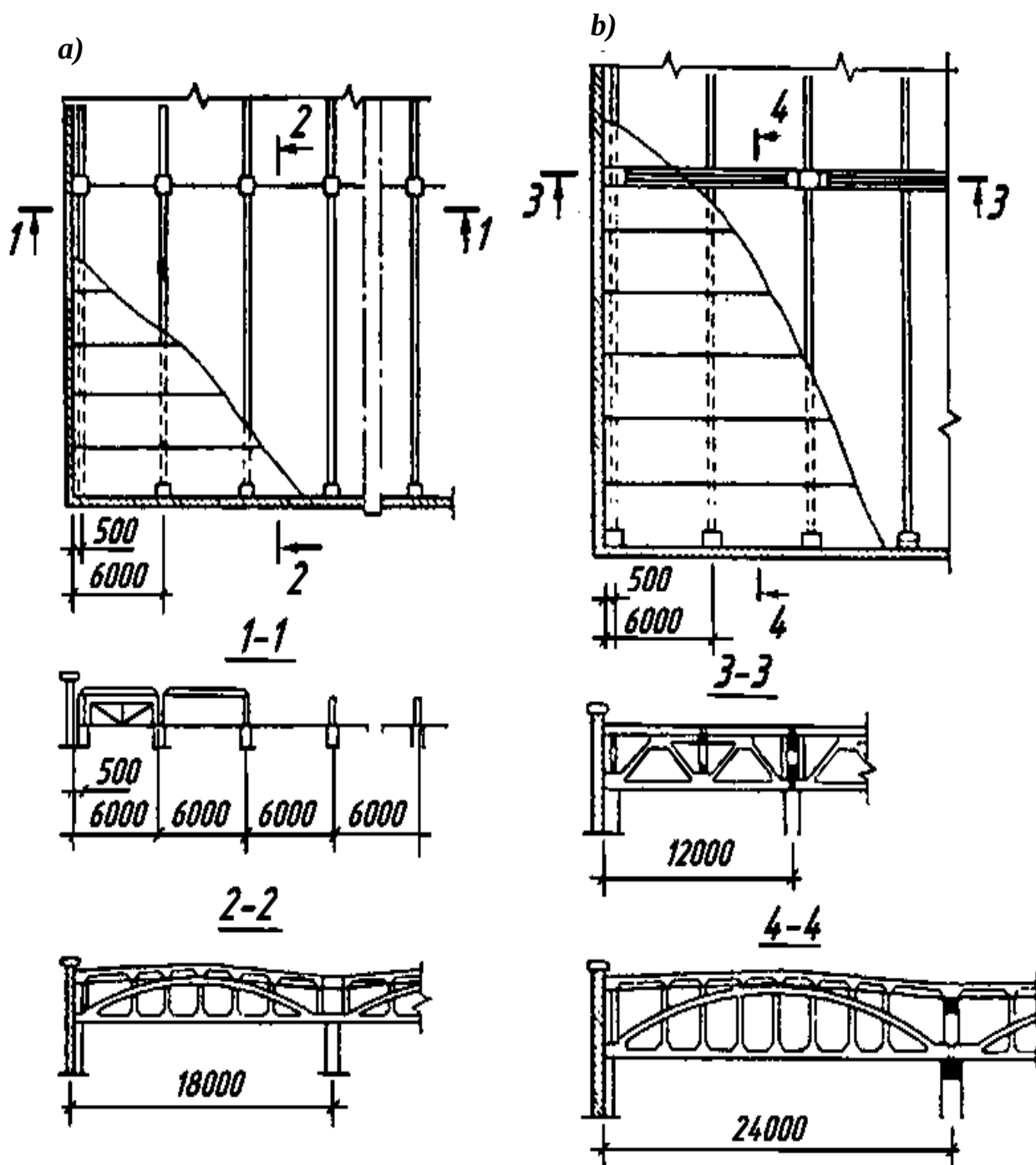
7.2-rasm. Bir qavatli sanoat binolarining konstruktiv sxemalari:
