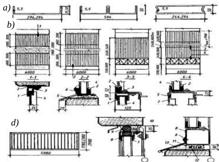
7.49-rasm. Shisha profillardan ishlangan deraza konstruksiyalari:
