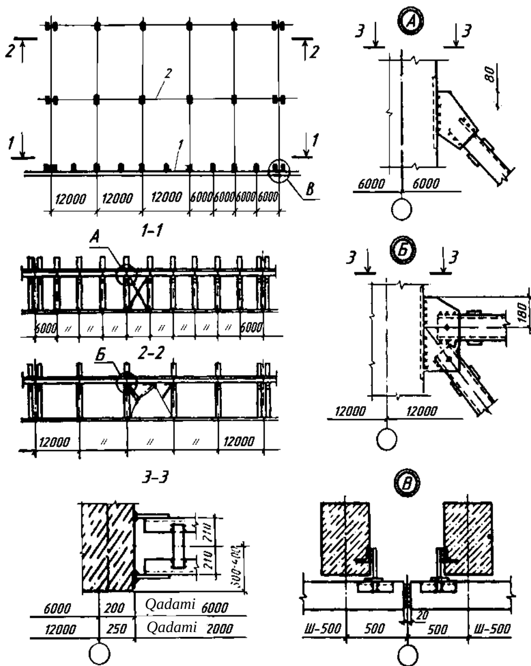
7.10-rasm. Ustunlararo vertikal bog‘lanishlar va harorat choklarini o‘rnatish:
