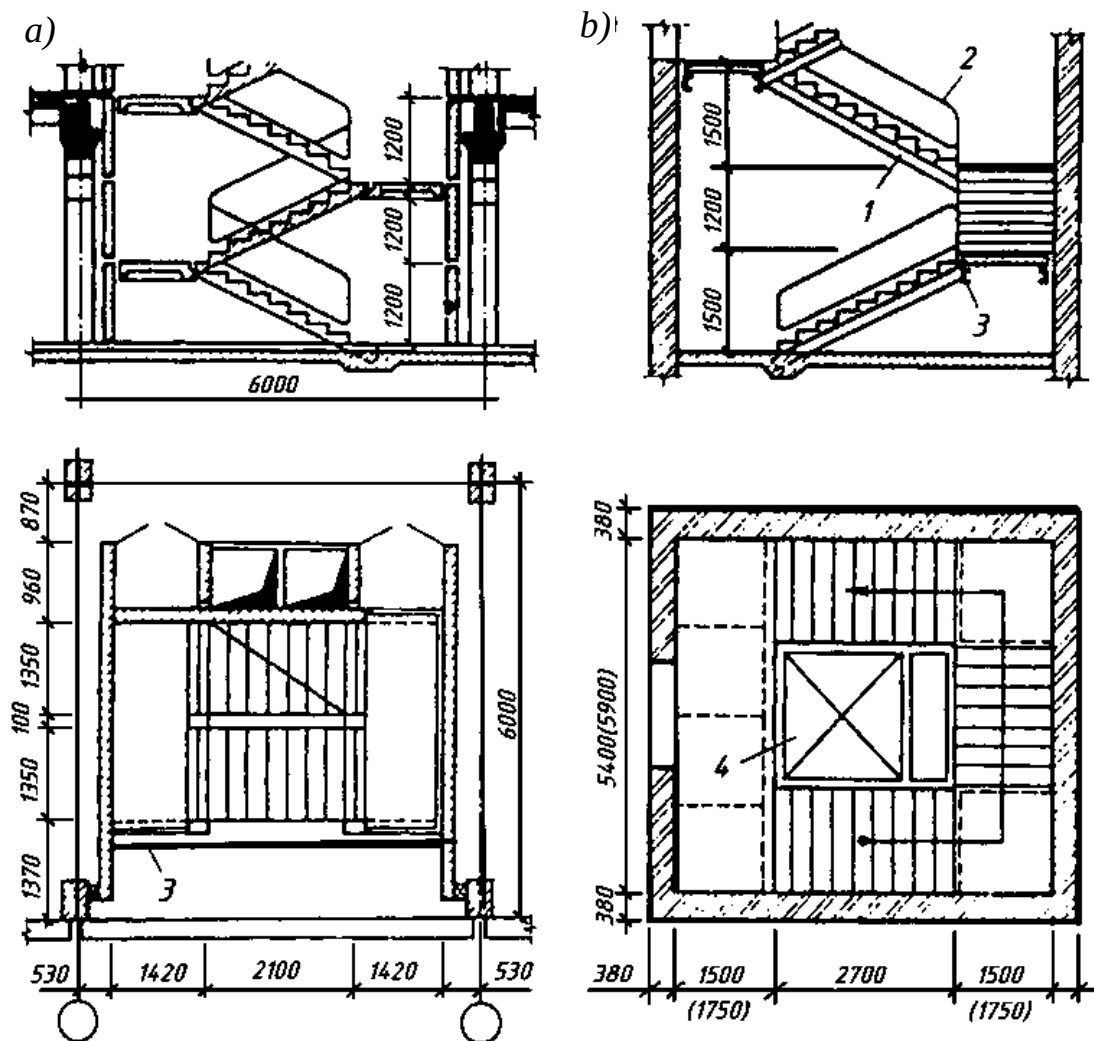
7.54-rasm. Ko‘p qavatli sanoat binosi zinalari.
