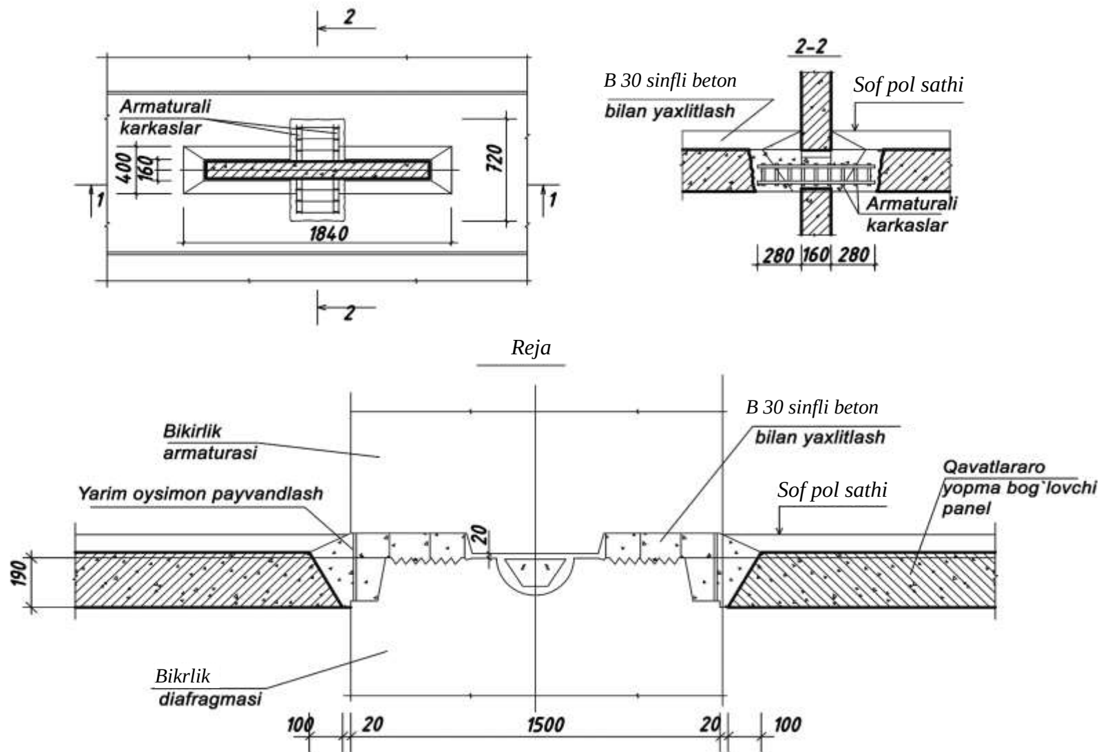
3.12-rasm. Qisqa bikrlilik diafragmalarining balandligi bo'yicha o'zaro birikishi.
