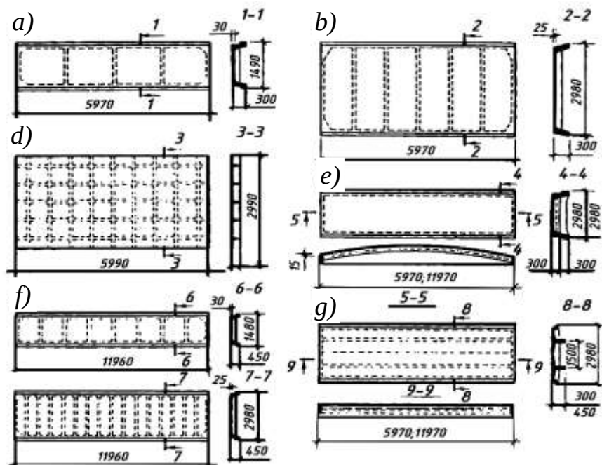
7.32-rasm. Tom yirik o'lchamli temirbeton panellari: a–3x6m o'lchamli; b–3x6m o'lchamli prokatli; g–ikki tomonga egilgan, armosementli; d–1,5x12 va 3x12m o'lchamli oldindan zo'riqtirilgan; e–3x6m va 3x12m o'lchamli ikki tokchali.
