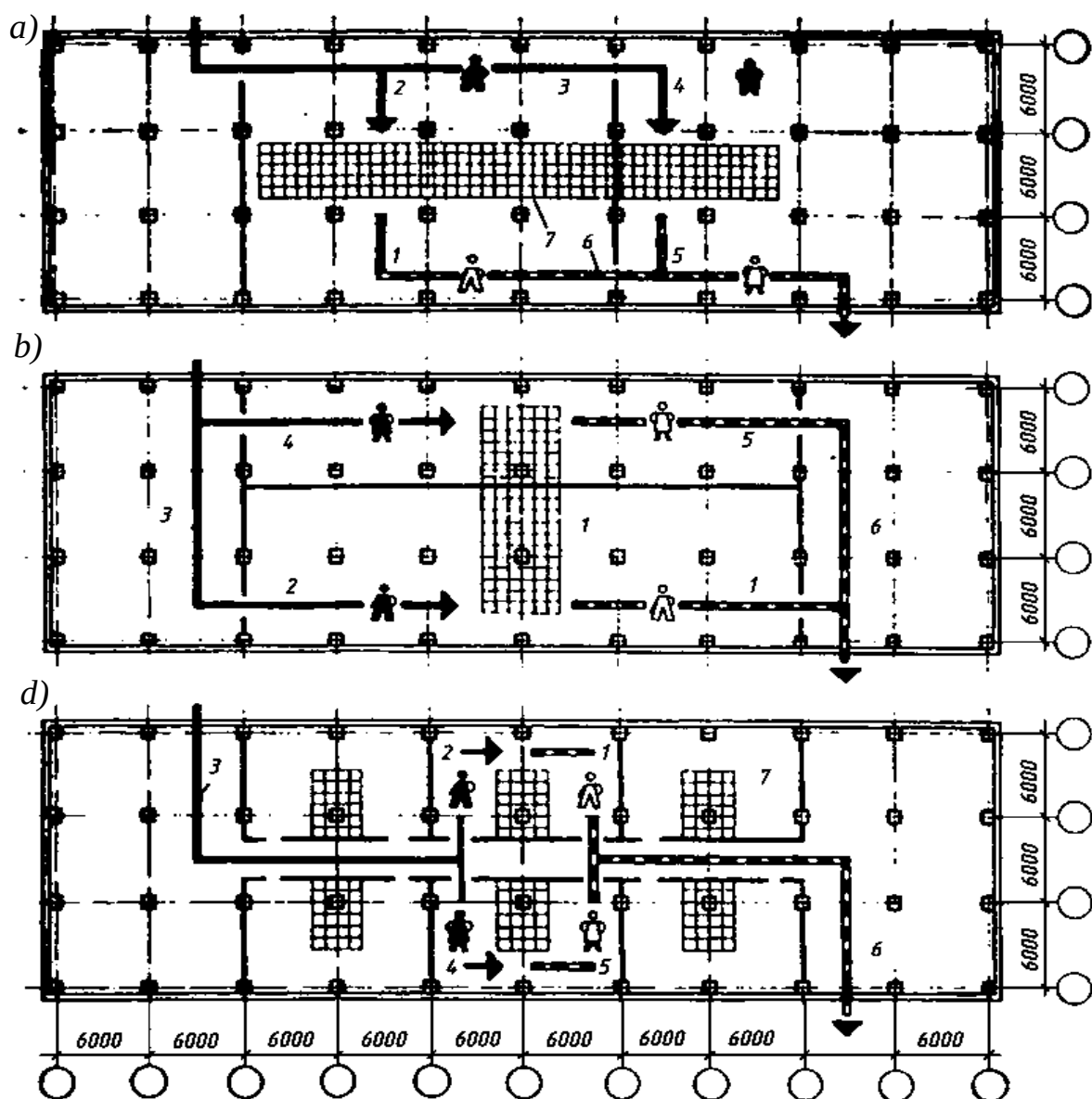
7.63-rasm. Garderob - dush bloki ayrim rejalarining sxemasi: a – markaziy bo‘ylama – joylashgan; b – bunda ham, ko‘ndalang – markaziy joylashgan; d – bunda ham, alohida seksiyali; 1 – erkaklar ko‘cha kiyimi uchun garderob; 2 – bu ham ish kiyimi uchun; 3 – ishlab chiqarishdan qaytayotgan ishchilar oqimi; 4 – ayollarning ish kiyimi garderobi; 5 – bu ham uy kiyimi uchun; 6 – ishlab chiqarishdan qaytayotgan kishilar oqimi; 7 – dushxona.
