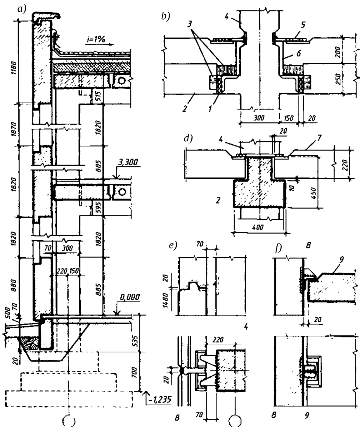
7.62-rasm. Ma'muriy-maishiy binolarni konstruktiv yechimlari: a – tashqi devor bo'yicha qirgimda; b – ustun tokchasiga rigellarning tutashishi; d – tom bog'lovchi plitalarni qotirish; e – devor panellarini ustunlarga qotirish; f – devor panellarini qotirish. 1 – bog'lovchi sterjen; 2 – rigel; 3 – rigel quyma detali; 4 – ustun; 5 – yuqori biriktiruvchi element; 6 – beton; 7 – bog'lovchi plita; 8 – devor paneli; 9 – devor oldi (chekka) plita.
