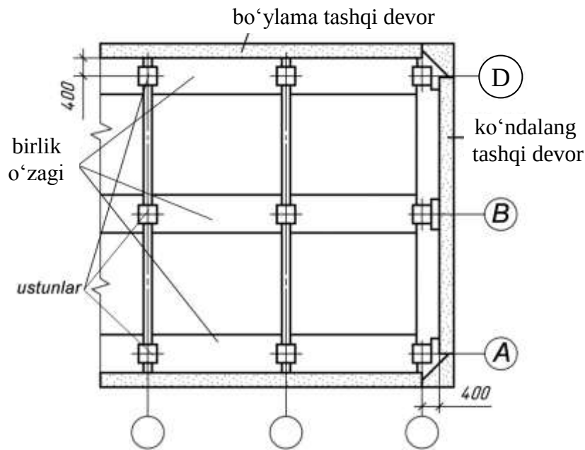
1.2-rasm. Devorlar va kolonnalarni koordinata reja o'qlariga bog'lash:
