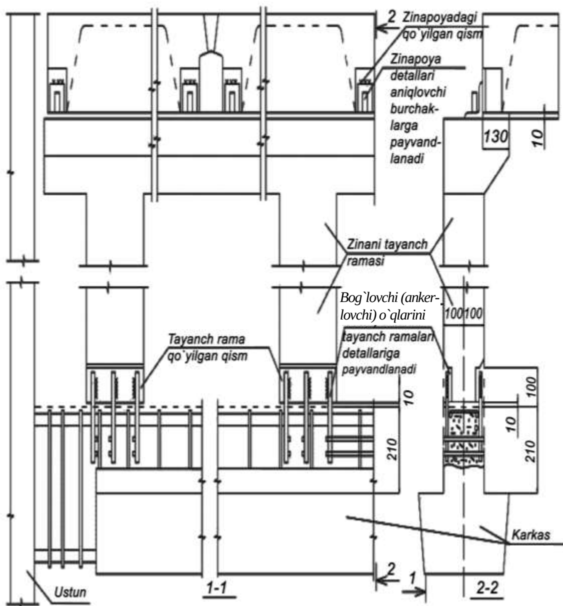
4.19-rasm. Panellardan reja urish uchun chiqib turgan armaturalarni biriktirish hollarida /betonning siqilgan qismi/ qo‘shimcha armaturasiz ichki va tashqi devor panellarining taraqqiy etgan yaxlit tutashishi.
