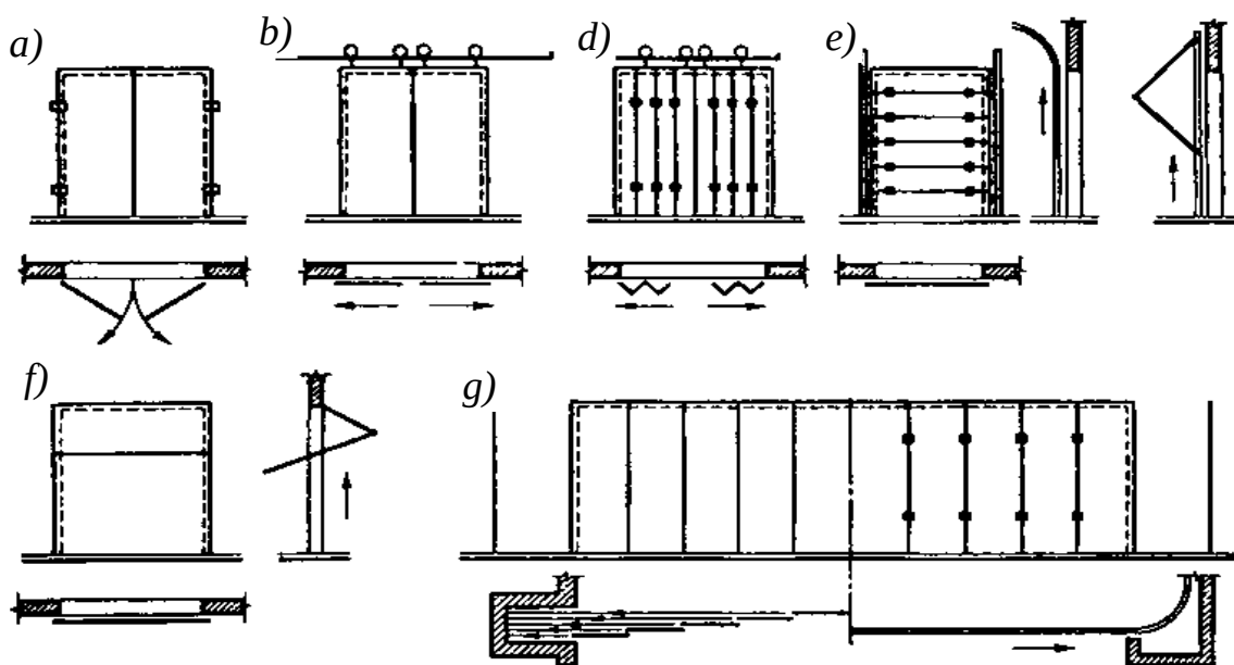
7.59-rasm. Sanoat binolari darvozalarining asosiy turlari.
