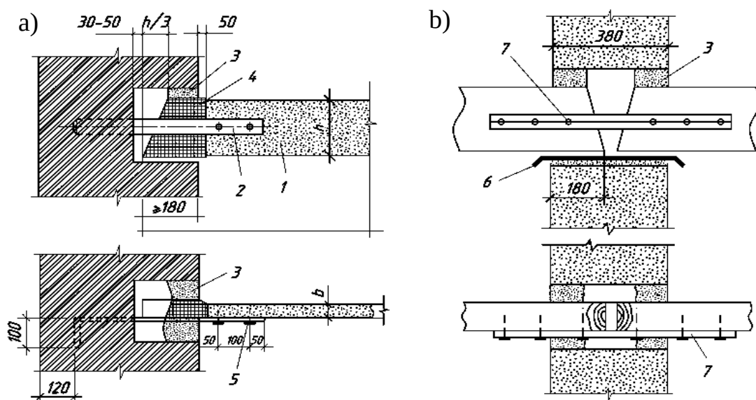
2.34-rasm. Yogʻoch toʻsinlarni gʻisht devorga ilintirish:
