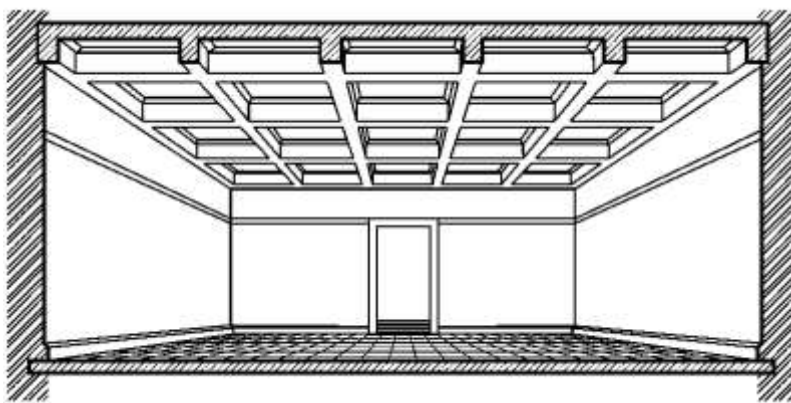
2.36-rasm. Quyma temirbetondan kesson tipida tayyorlangan yaxlit plita.
