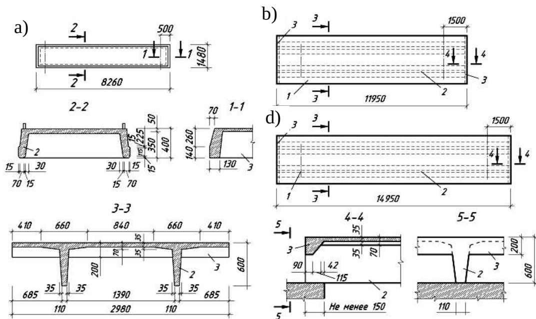
2.44-rasm. Oʻlchamlari 9,12 va 15 m boʻlgan plita-toʻshmalar: 1–montaj elementi; 2–boʻylama qovurgʻa; 3–koʻndalang qovurgʻa.
