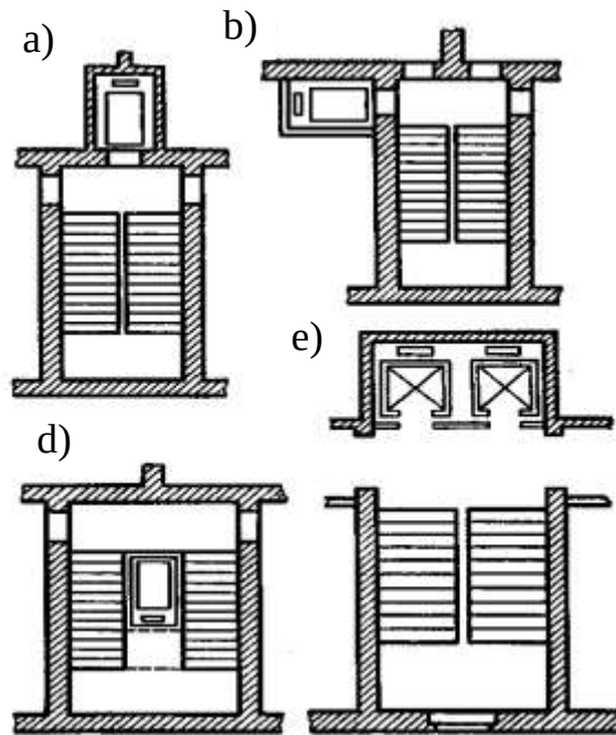
2.75-rasm. Lift shaxtalarini turar-joy binolarida joylashtirish sxemalari:
