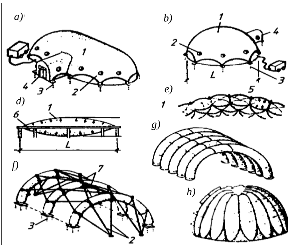
7.44-rasm. Havo berib shishiriladigan tom qobiqlarining ko‘rinishlari:
