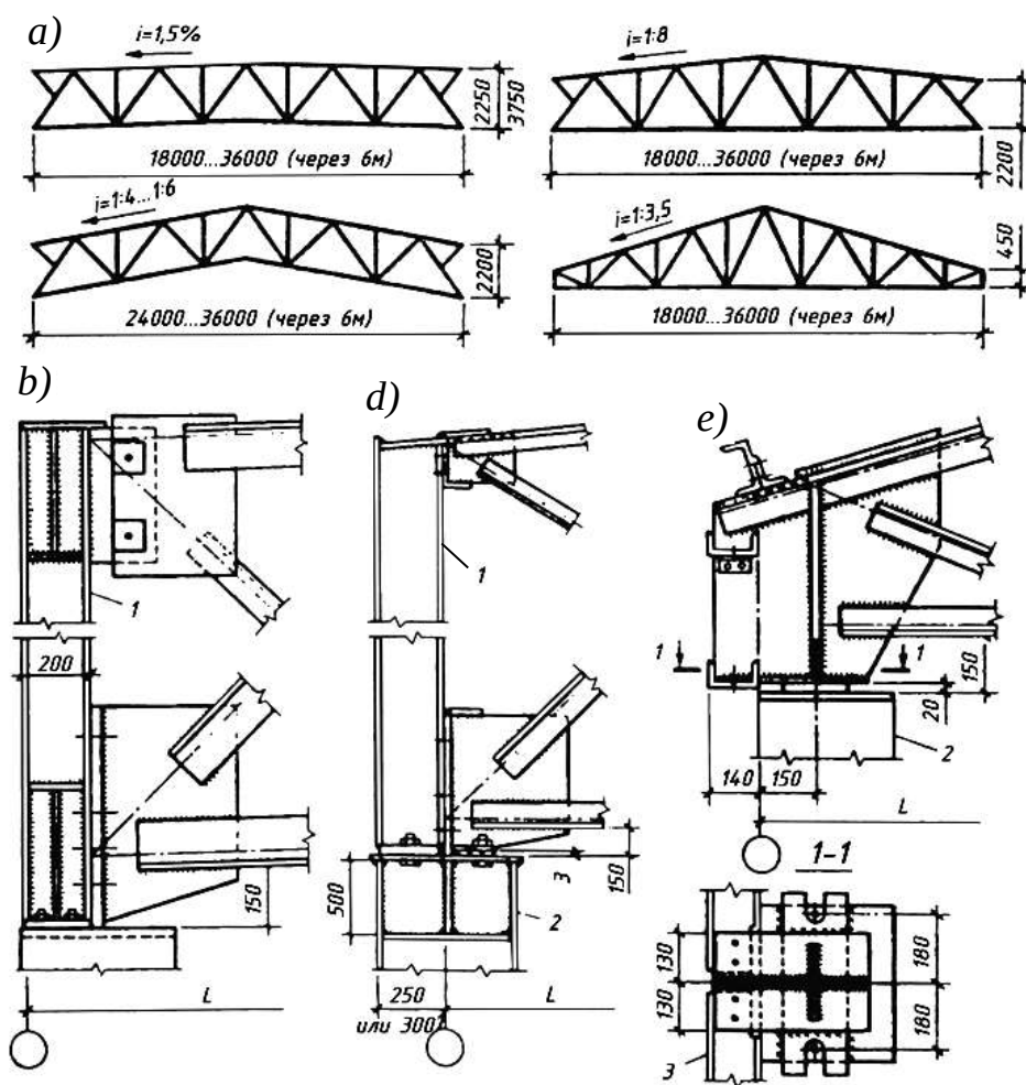
7.40-rasm. Po'latdan ishlangan storopil fermalari:
