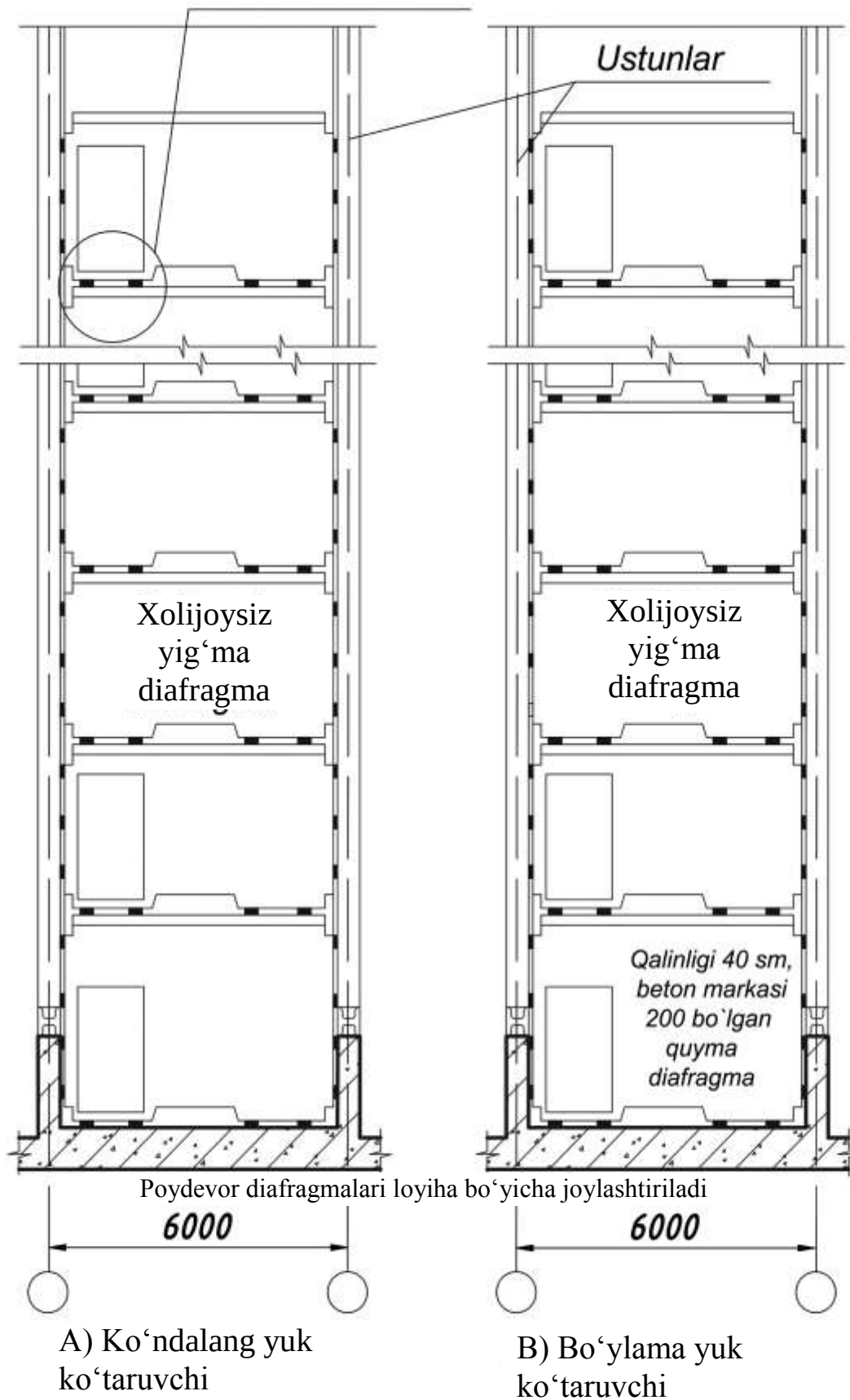
3.5-rasm. Bikrlik diafragmasini joylashtirish sxemasi.
