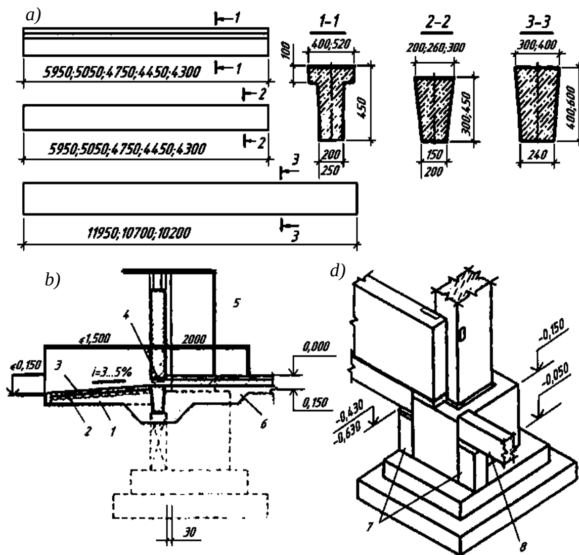
7.7-rasm. Chekka qator ustuni poydevorlari detallari: a – poydevor to‘sinlari turlari; b, d – detallar.
