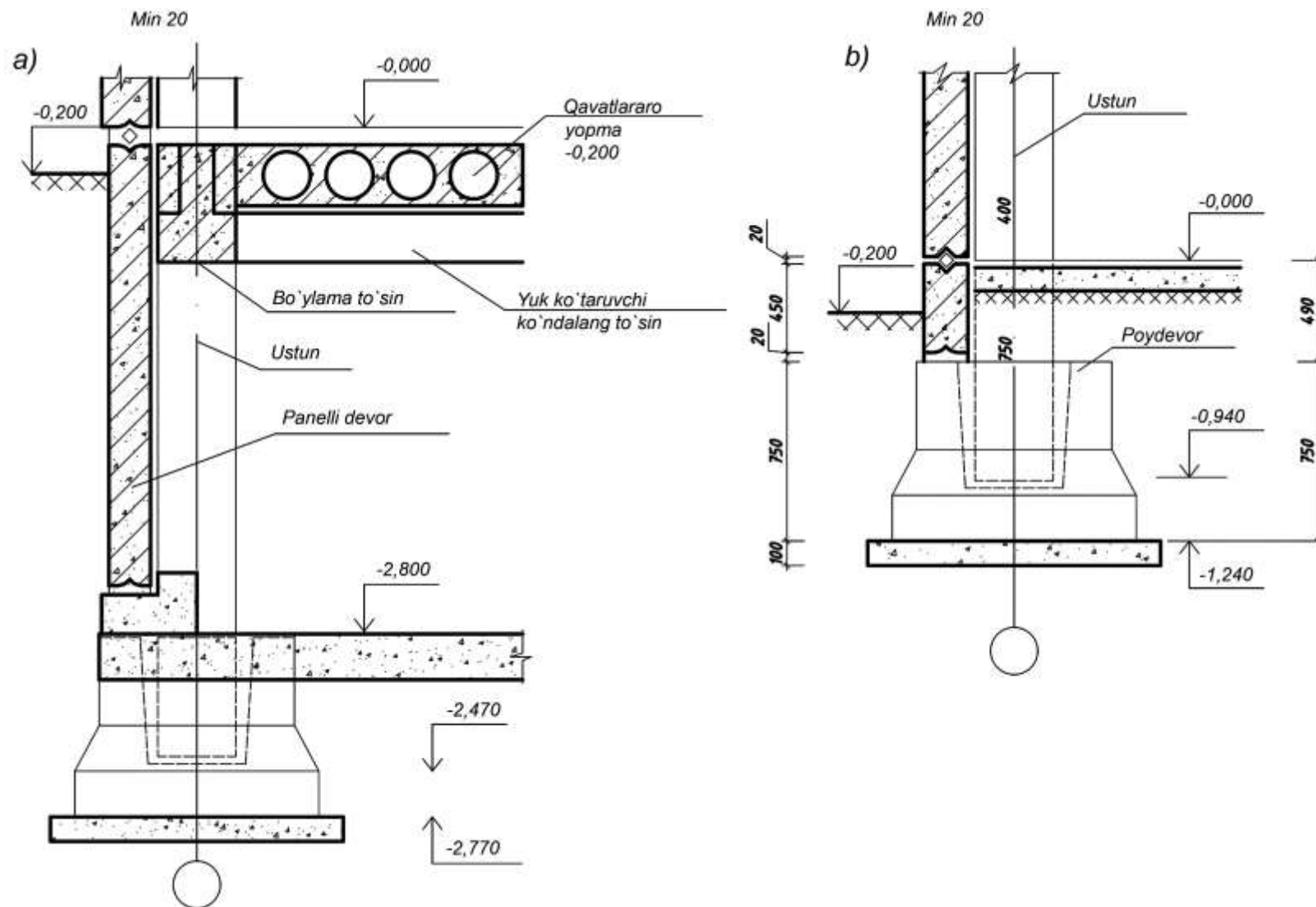
3.1-rasm. Bino yer ostki qismining tashqi o'q bo'yicha qirqimi:
