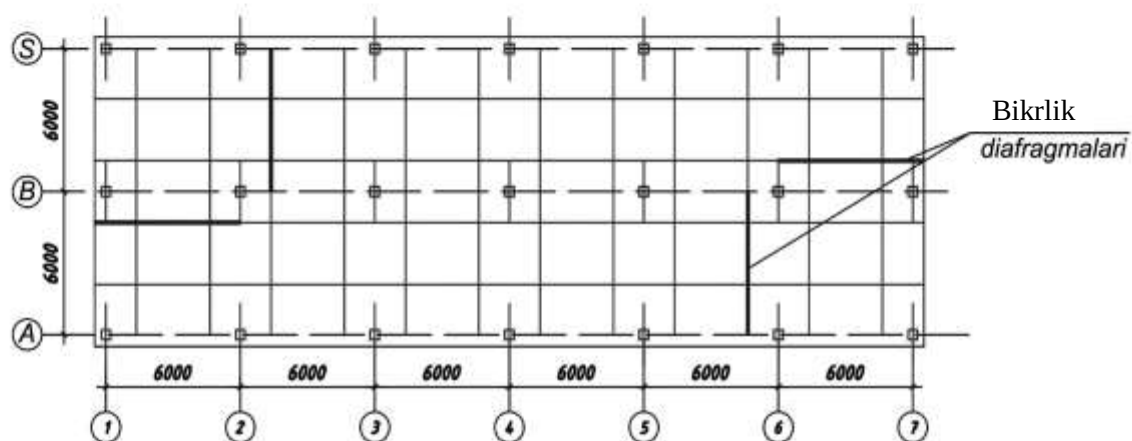
B) Ko'ndalang va bo'ylama yo'nalishda qavatlararo yopmalarni va bikrlik diafragmalarini joylashishi
