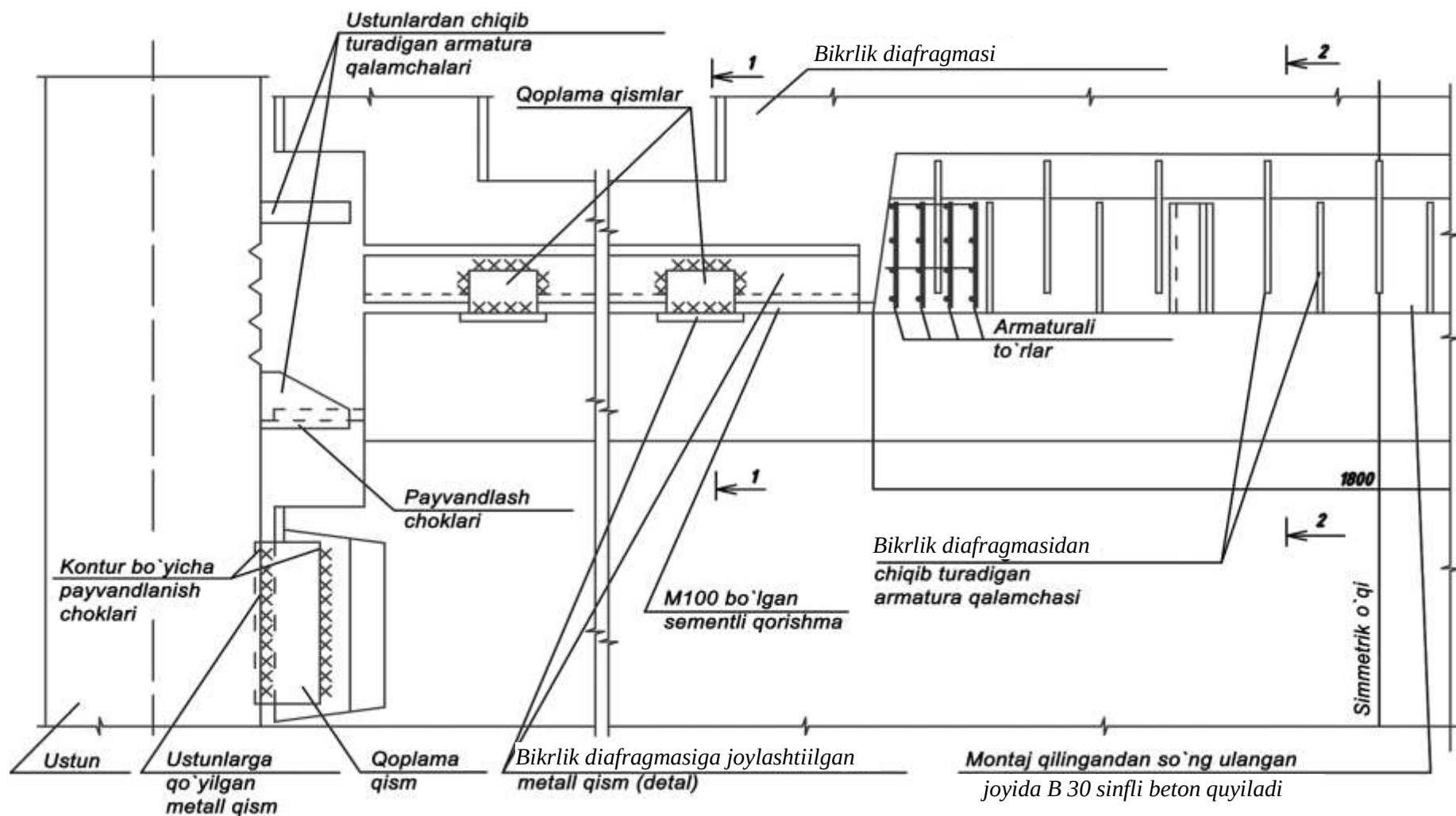
3.13-rasm. Bikrlik diafragmalarining balandligi bo'ylab bir-biri va ustun bilan bog'lanishi.
