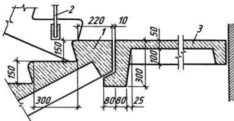
2.71-rasm. Yig‘ma temirbeton konstruksiyadan ishlangan zina detali:
