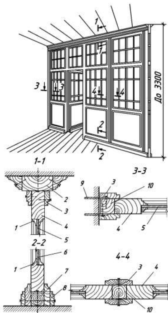
2.52-rasm. Jamoat binolarida uchraydigan parda devorlar:
