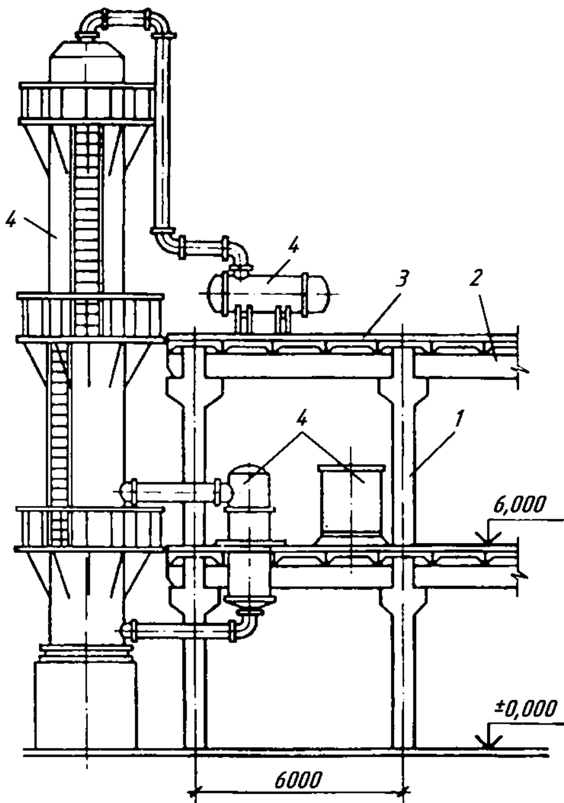
7.57-rasm. Sanoat binosi etajerkasi: 1 – ustun; 2 – ishchi maydon; 4 – texnologik jihozlar.
