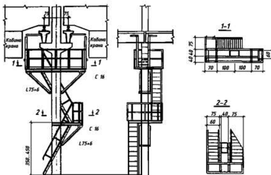
7.56-rasm. Ko'prik kraniga chiqish uchun mo'ljallangan xizmat zinasining sex ichki ustunlarida joylashish sxemasi.
