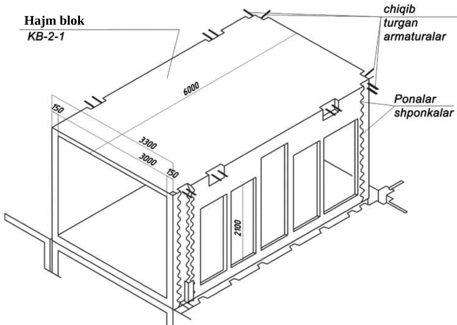
5.10-rasm. Hajm-blokni montaj vaqtidagi aksonometrik sxemasi.
