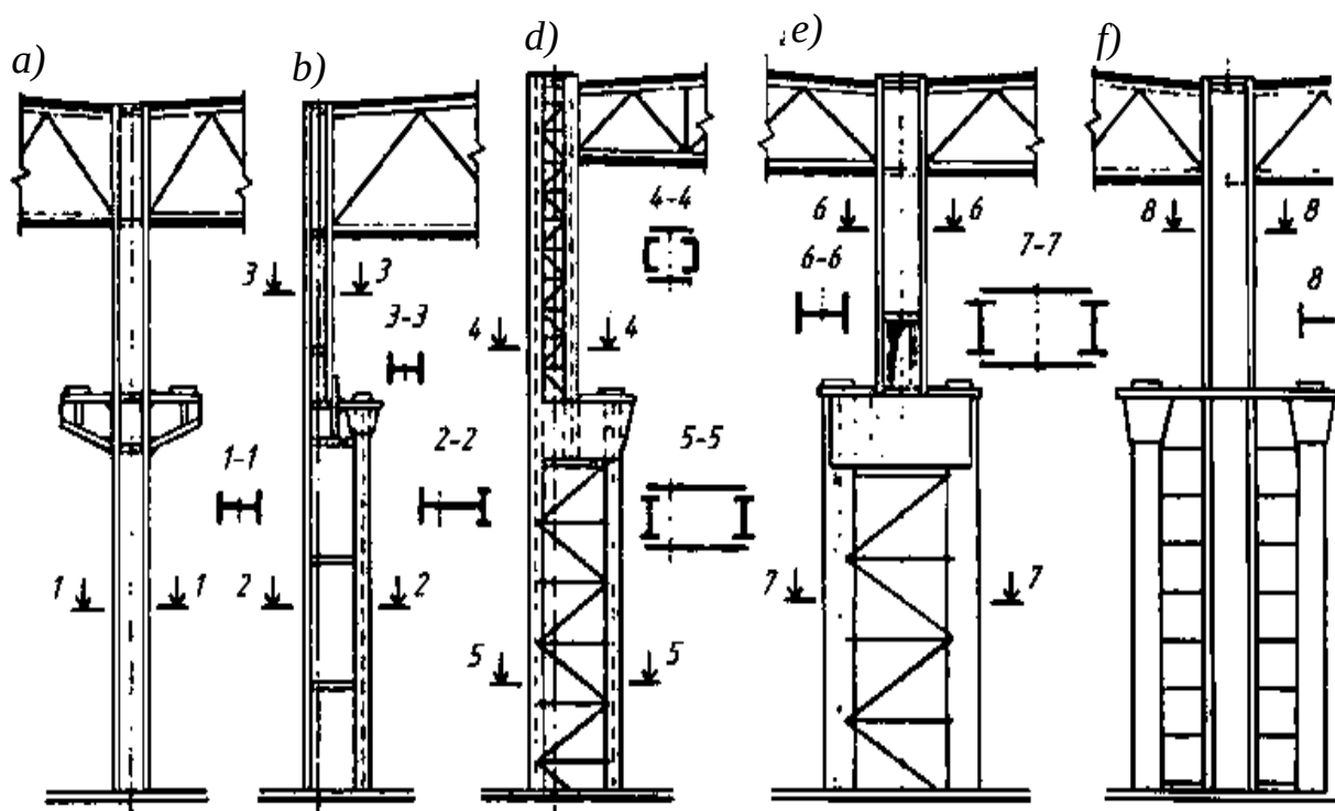
7.19-rasm. Po‘lat ustunlarning asosiy turlari:
