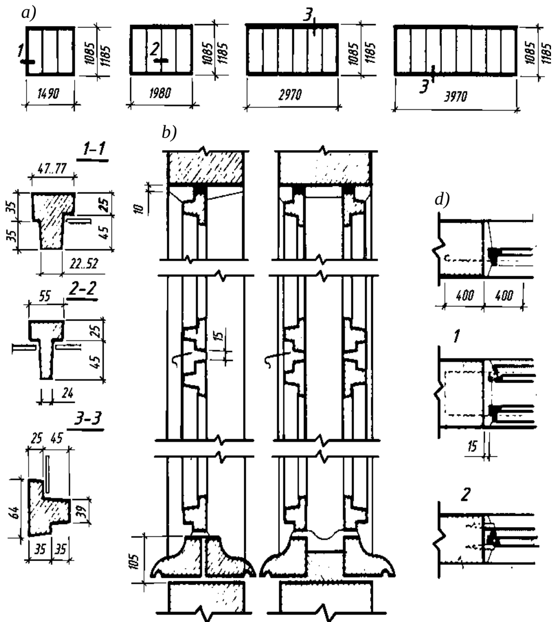
7.47-rasm. Temirbeton deraza tavaqalari:
