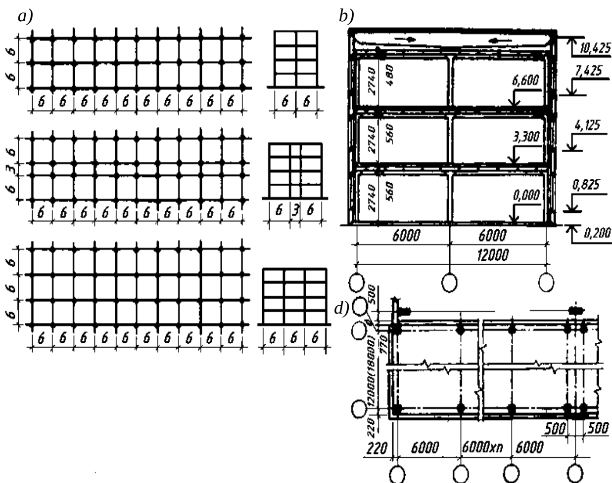
7.65-rasm. Ma'muriy-maishiy binosini hajmiy-tarxiy yechimlariga doir misollar.
