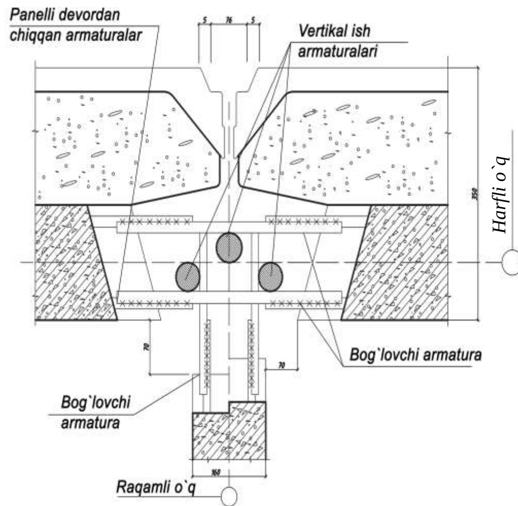
4.18-rasm. Panellardan urish uchun chiqib turgan armaturalarni biriktirish hollarida /betonning cho‘zilgan qismi/ qo‘shimcha armaturalash bilan ichki va tashqi devor panellarining taraqqiy etgan yaxlit tutashishi.
