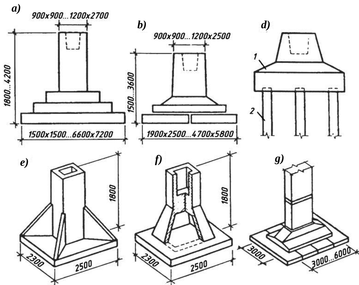
7.5-rasm. Sanoat binolarining poydevorlarini turlari:
