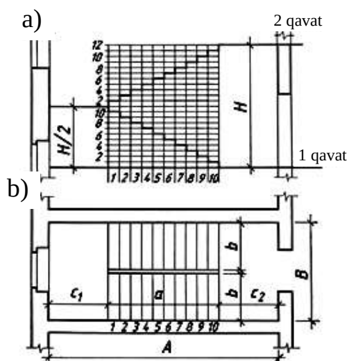
2.73-rasm. Zinalarni grafik usulda hisoblash: a – kesimda; b – tarxda ko‘rinishi.
