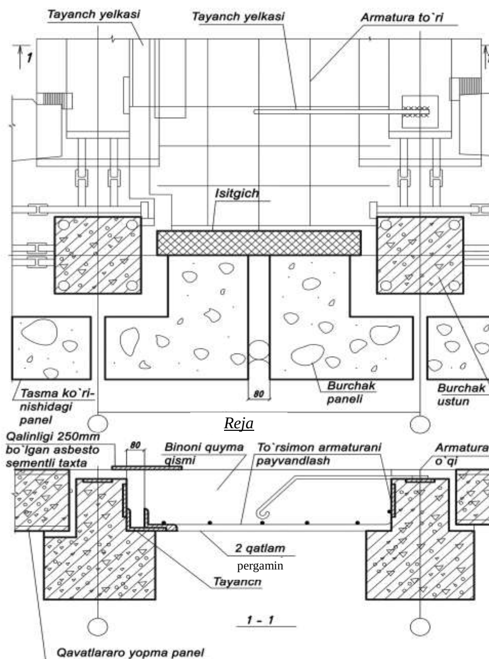
3.23-rasm. Zilzilaga qarshi choraklarda qavatlararo yopmalarni o'rnatish.
