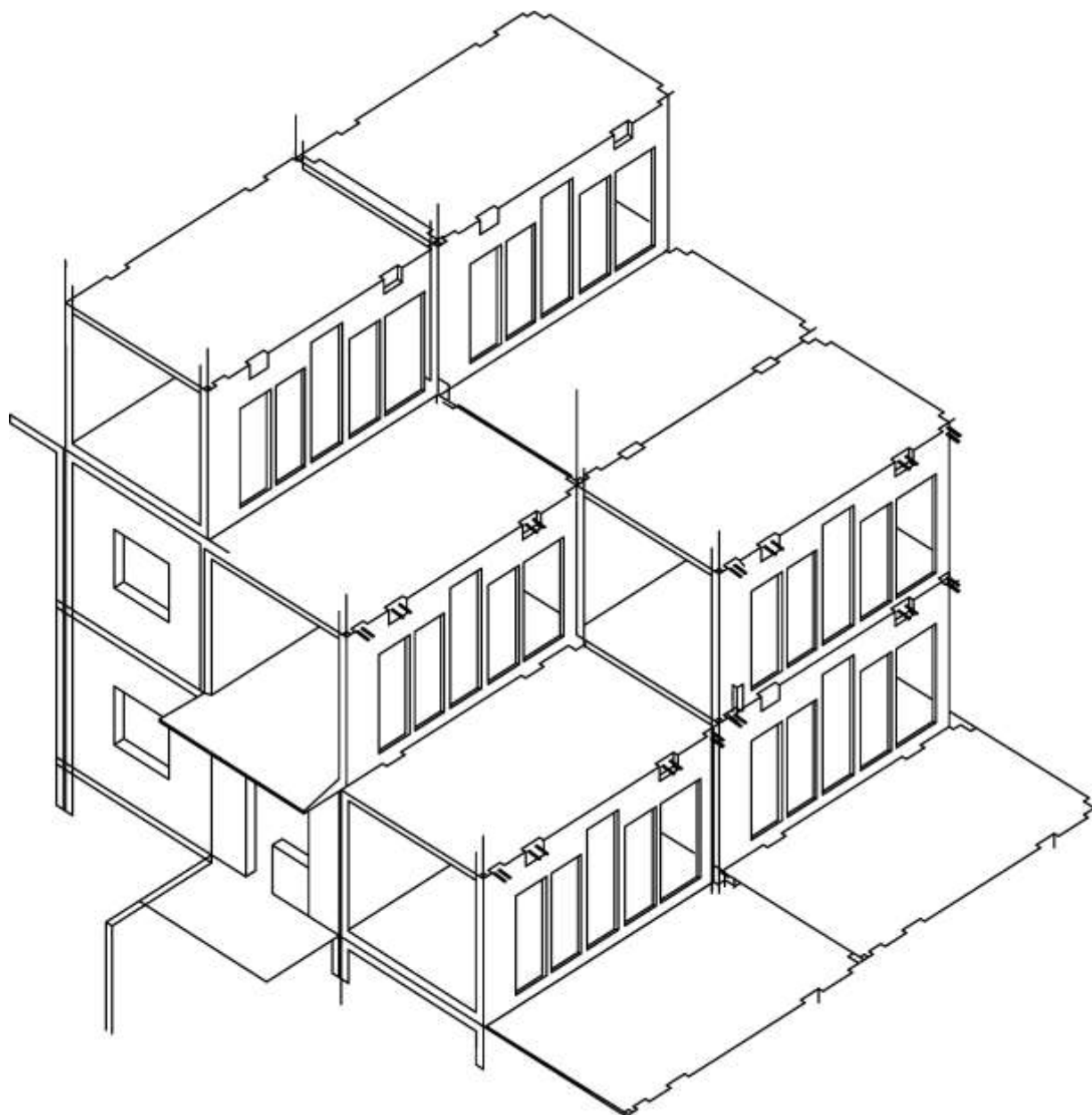
5.1-rasm. Hajm-blokli uyning montaj jarayonining bir qismi.
