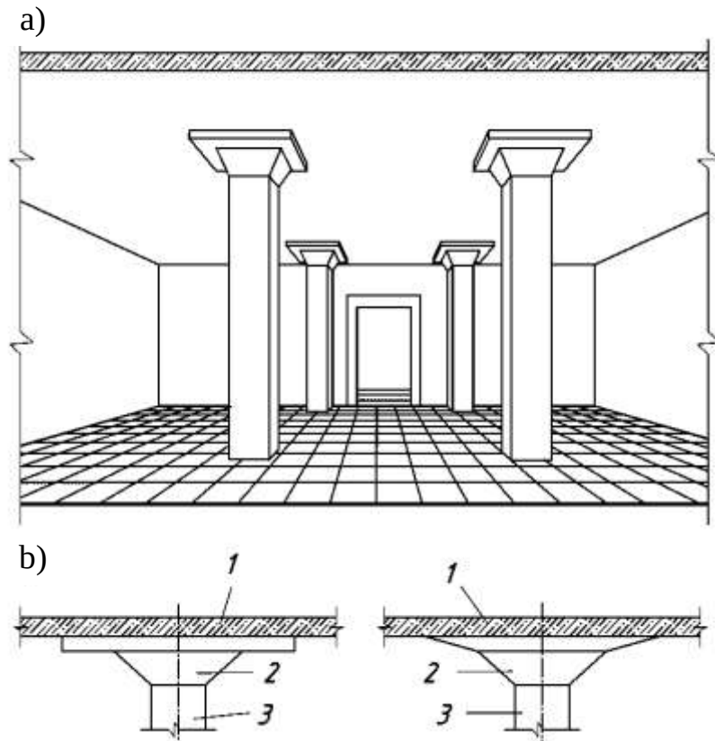
2.39-rasm. To‘sinsiz quyma temirbeton ora yopmalar: a – umumiy ko‘rinishi; b – plitalarning ustunlarga tayanish sxemalari; 1 – plita; 2 – kapitel; 3 – ustun.
