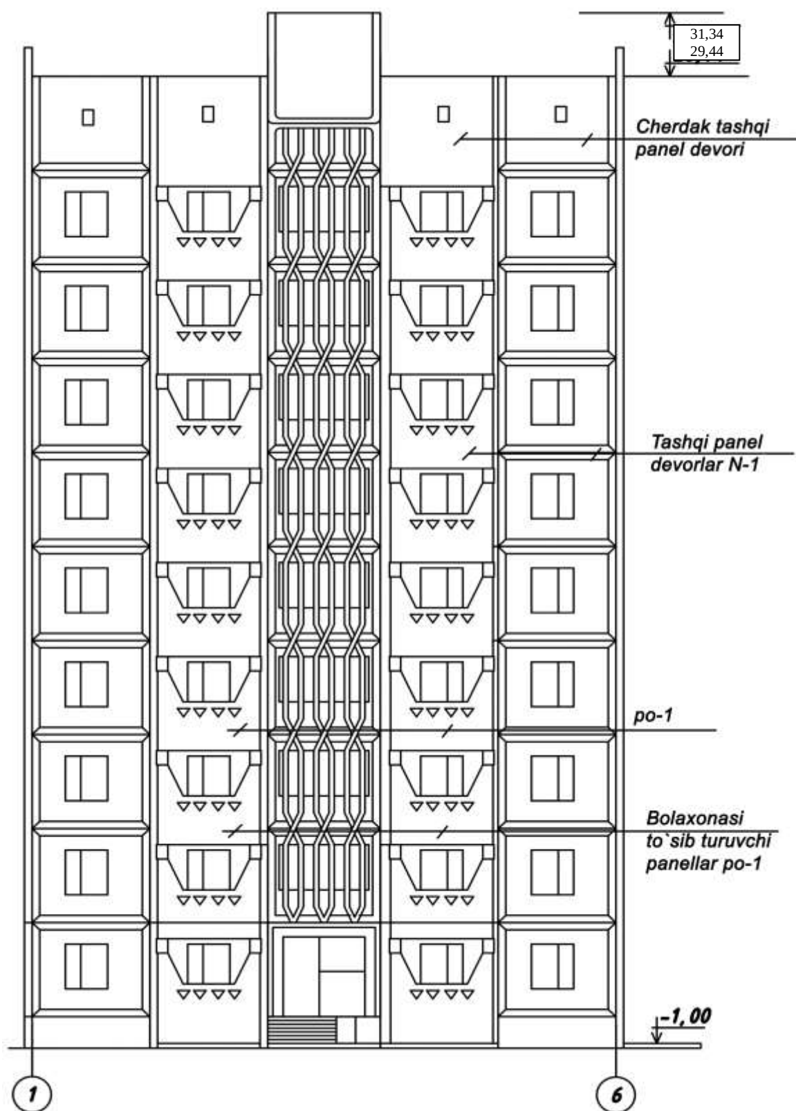
5.6-rasm. Blok-seksiyaning tarzi.
