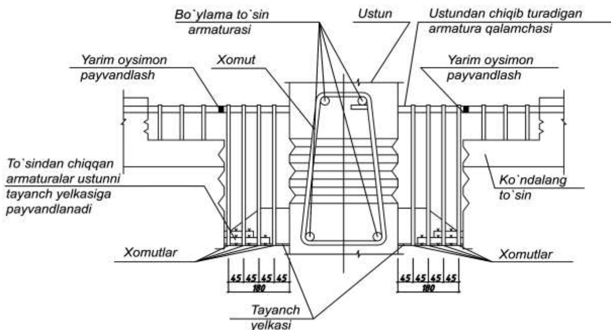
3.9-rasm. Yig'ma to'sinlarni ustun bilan ulanishida to'sin armaturalari ustunning yopiq yelkasiga o'rnatilishi.
