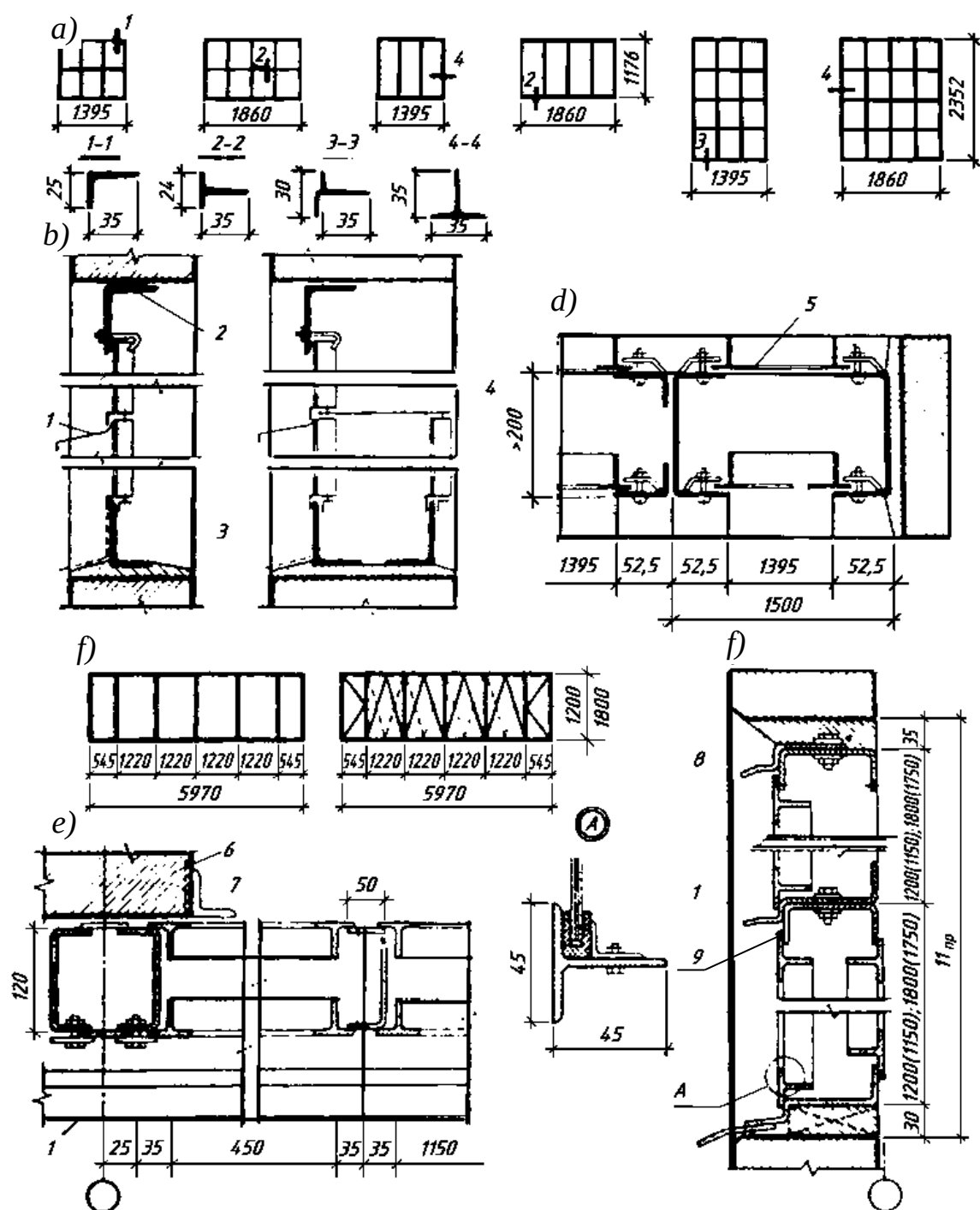
7.48-rasm. Po‘lat egilgan va prokat profillardan ishlangan deraza tabaqalari:
