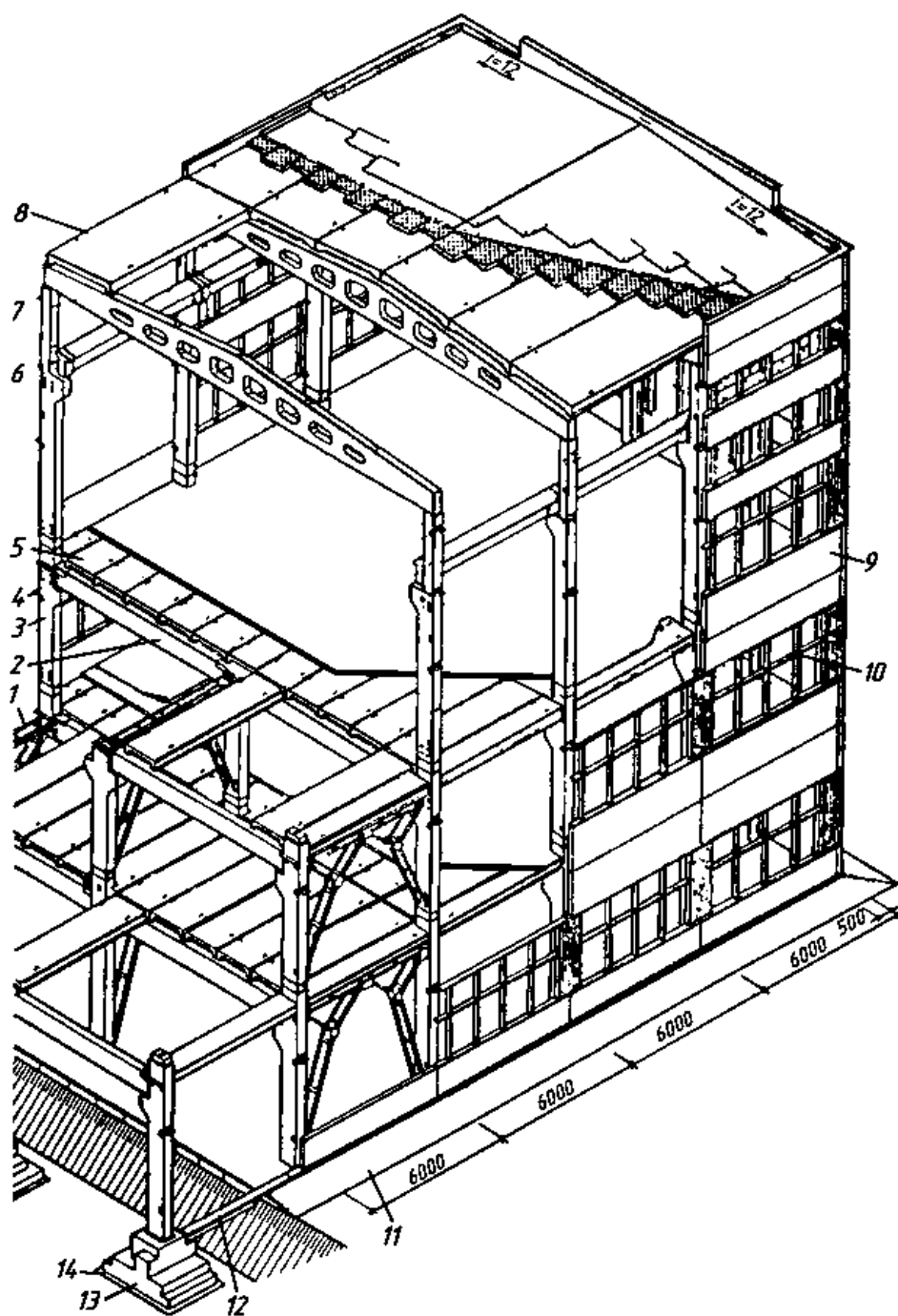
7.3-rasm. Ko‘p qavatli sanoat binosining konstruktiv yechimi: 1–ustunlar oralig‘idagi vertikal peshtoq shakldagi metall bog‘lanish; 2– to‘sin (to‘sin, rigel); 3–ustun; 4–devor panelini tayanishi uchun moslashtirilgan tayanch; 5– qavatlararo yopma plitasi; 6–kranosti to‘sini; 7–tom to‘sini; 8–tom temirbeton yopma plitasi; 9–devor paneli; 10–deraza konstruksiyasi; 11–otmostka; 12–temirbeton poydevor to‘sini; 13–temirbeton poydevor; 14–qum shag‘al qatlami.
