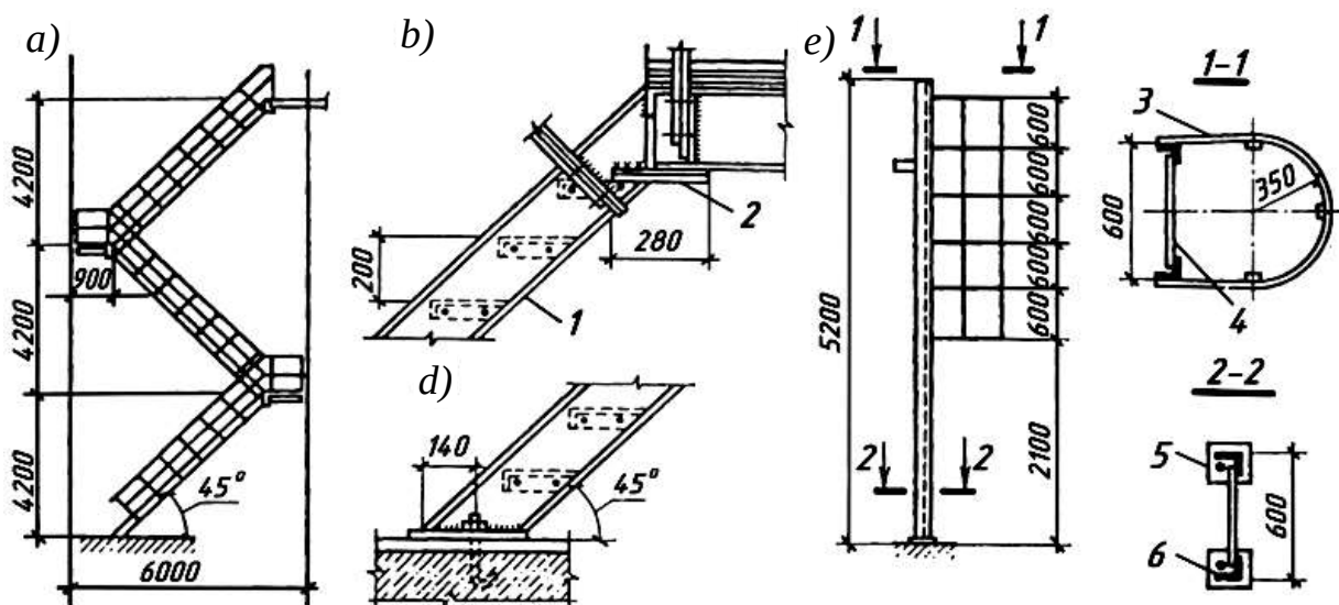
7.55-rasm. Xizmat zinalarining konstruktiv yechimlari:
