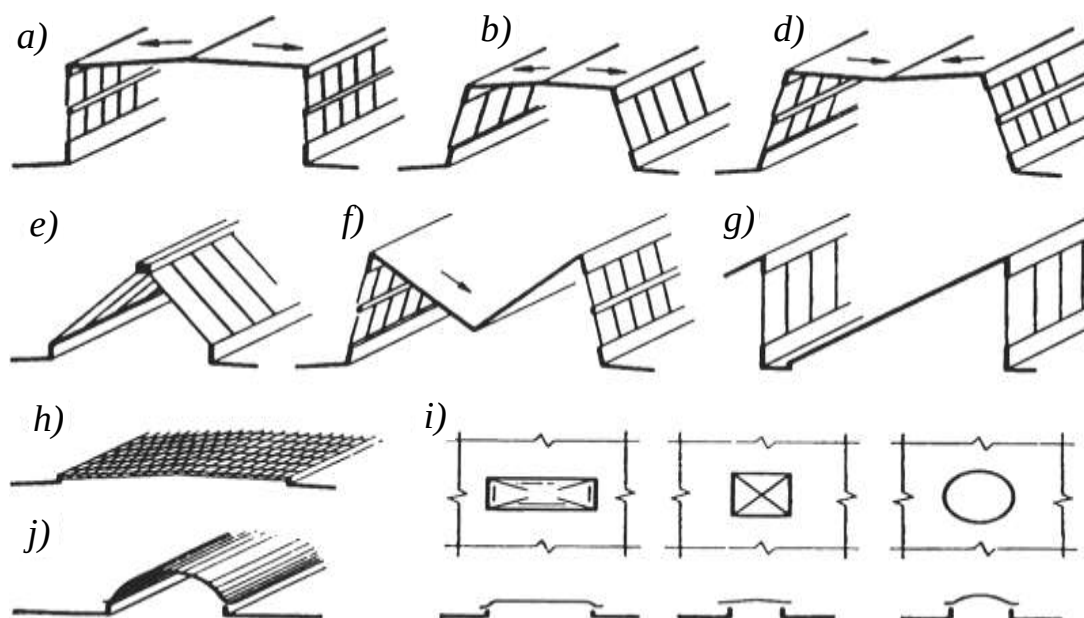
7.50-rasm. Yorug'lik va aeratsiya fonarlarining asosiyl profillari:
