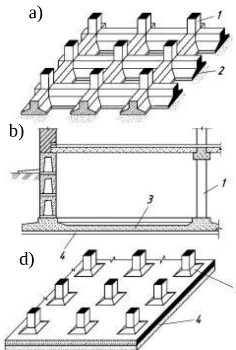
2.13-rasm. Yaxlit poydevorlarning ko'rinishi.
