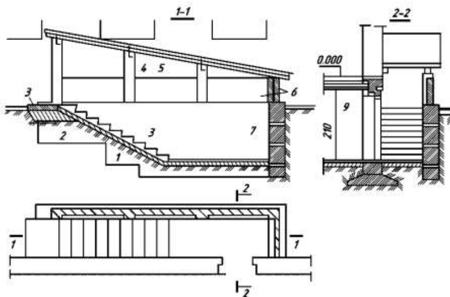
2.15-rasm. Yerto‘la qavati xonalariga kirish:
