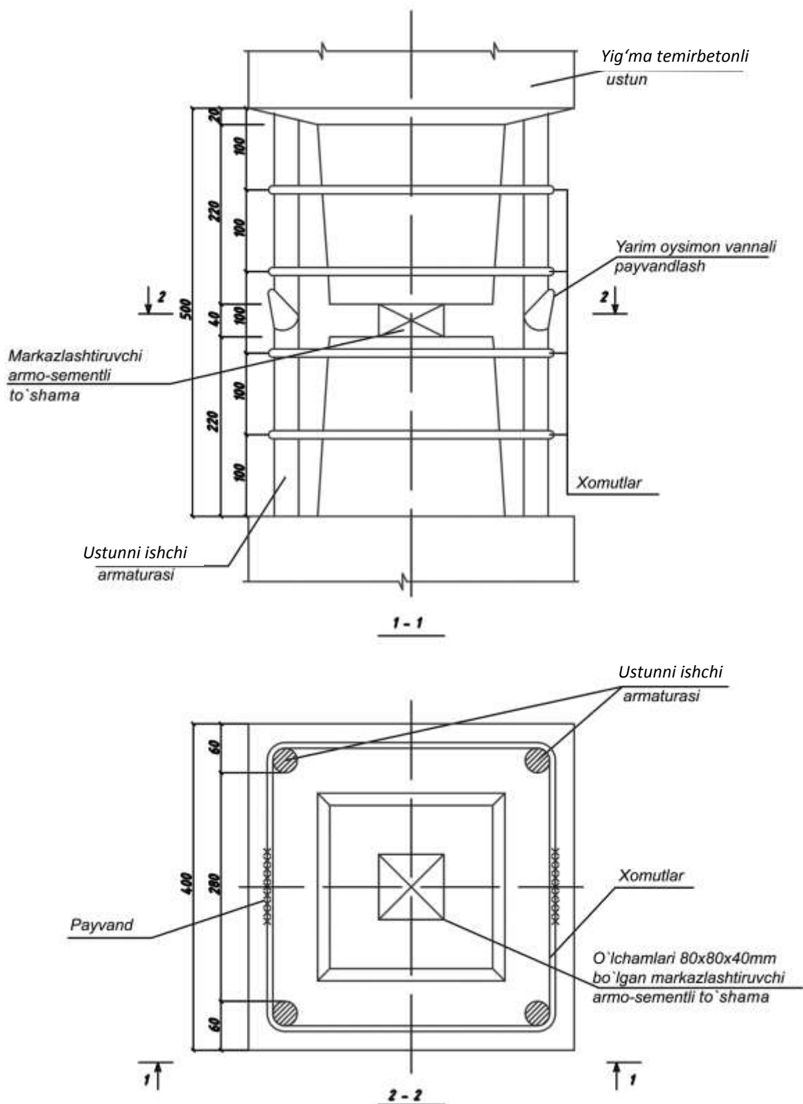
3.8-rasm. Markazlashtiruvchi toʻshama yordamida ustunlarning birikish joyi.
