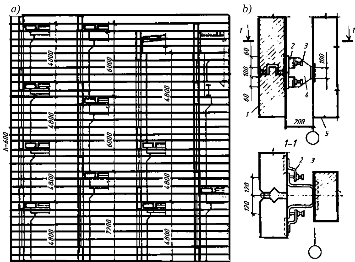
7.26-rasm. Ko‘p qavatli sanoat binolarining devorlari: a – panellarni bino balandligi bo‘yicha joylanishi; b – panellarni ustunlarga qotirish detallari. 1 – panel; 2 – tortuvchi bolt kronshteyni; 3 – tortuvchi bolt; 4 – bog‘lovchi detal; 5 – ustun.
