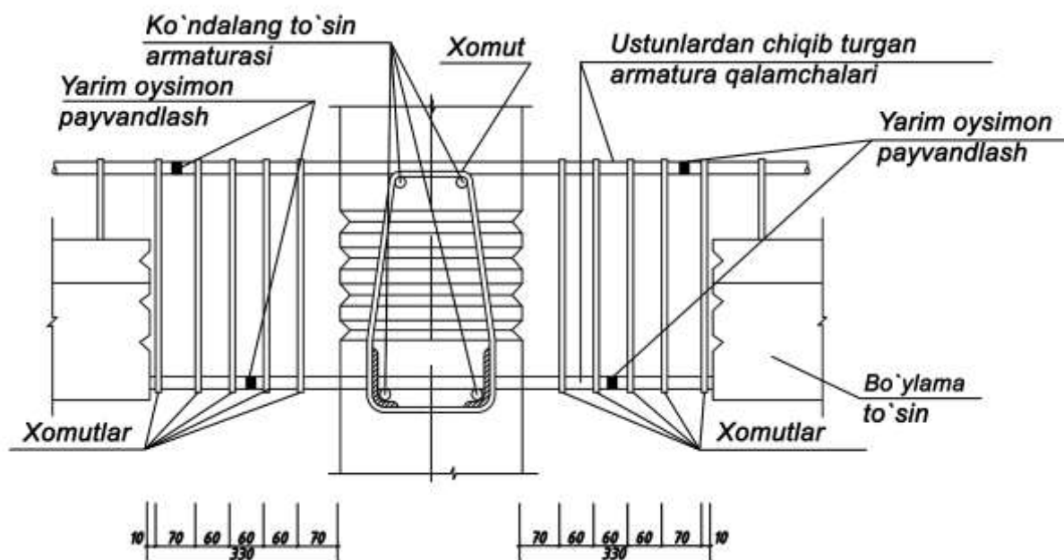
3.10-rasm. Tayanch tirsaklarsiz ustun bilan yig'ma to'sinlarning bir-biri bilan bog'lanishi.
