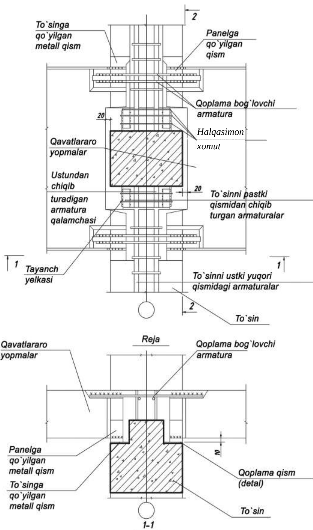
3.15-rasm. Qavatlararo yopmalarning to'sinlar bilan bog'lanishi.
