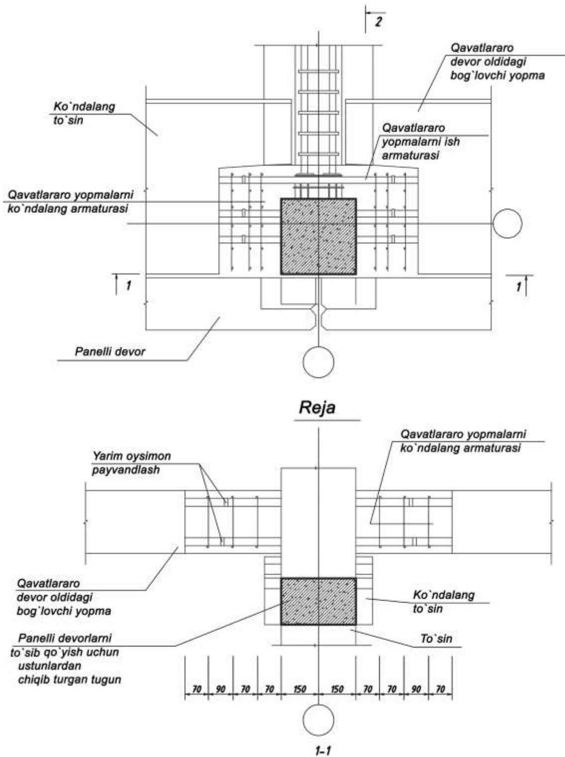
3.14-rasm. Devor oldidagi bogʻlovchi yopmalarning va koʻndalang toʻsinlarni ustun bilan bogʻlanishi.
