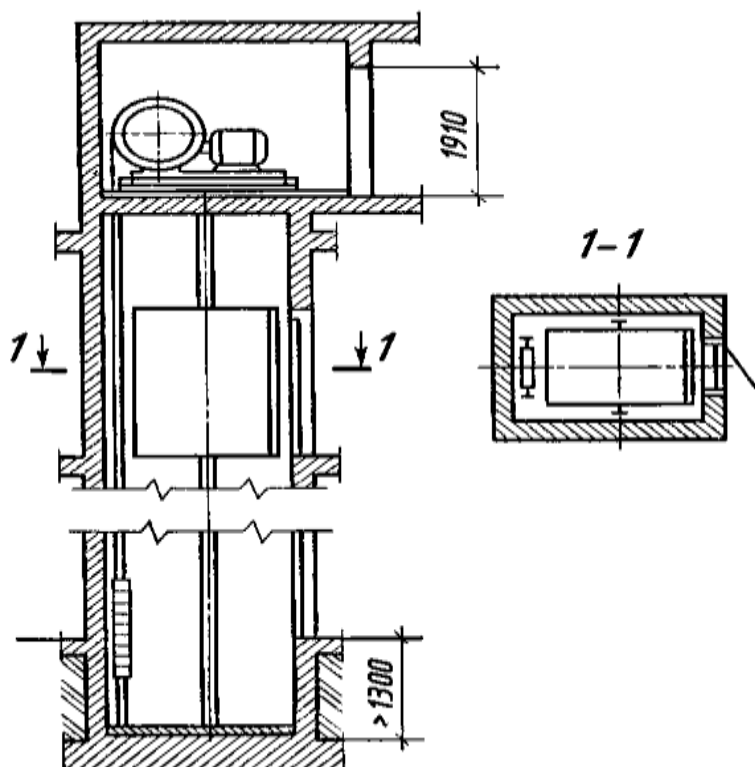
2.74-rasm. Mashina bo'limi yuqorida joylashgan turar-joy binolariga mo'ljallangan lift.
