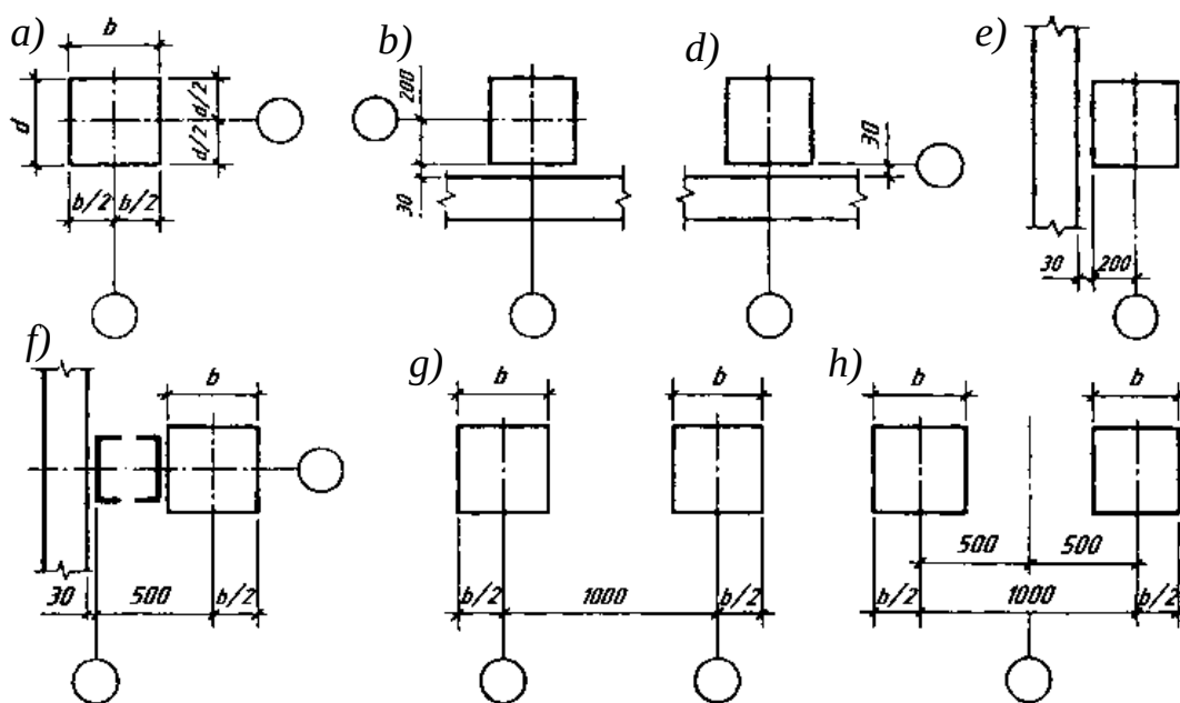
7.16-rasm. Ko‘p qavatli sanoat binolarining ustun va devorlarini koordinatsiya o‘qlariga bog‘lash:
