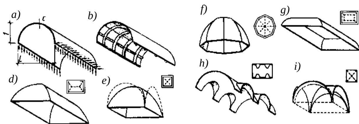
7.42-rasm. Sanoat binolari tomlarida ishlatiladigan qobiqlar.
