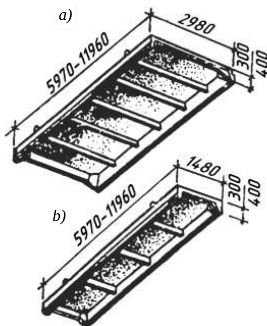
7.31-rasm. Yirik o'lchamli temirbeton panellarini ko'rinishi: a – yopmaning asosiy plitasi; b – yopmaning qo'shimcha plitasi.
