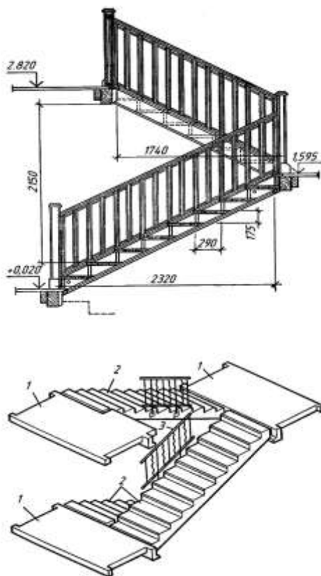
2.70-rasm. Yig‘ma elementlardan tuzilgan zina:
