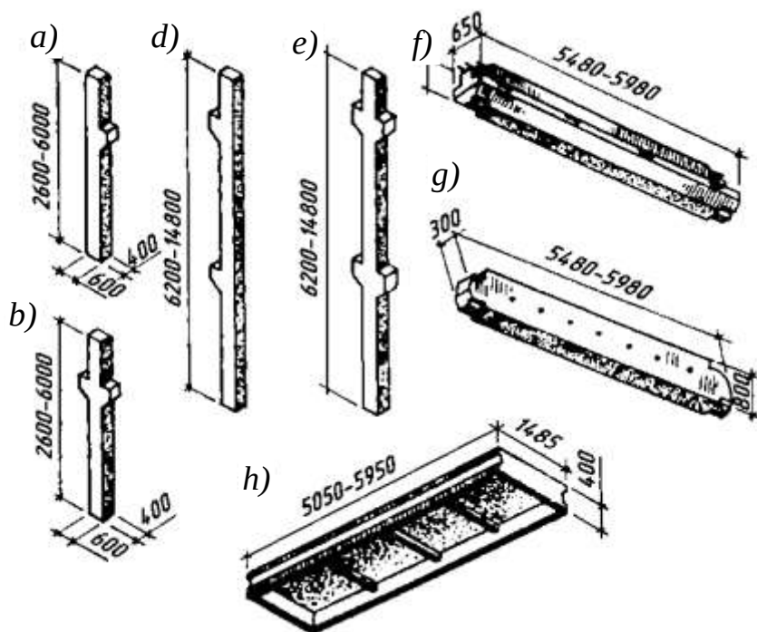
7.15-rasm. Ko‘p qavatli binolarda ishlatiladigan temirbeton konstruksiyalar:
