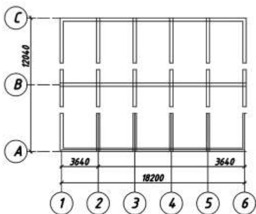
5.7-rasm. Yerto'la panelning joylashish sxemasi.
