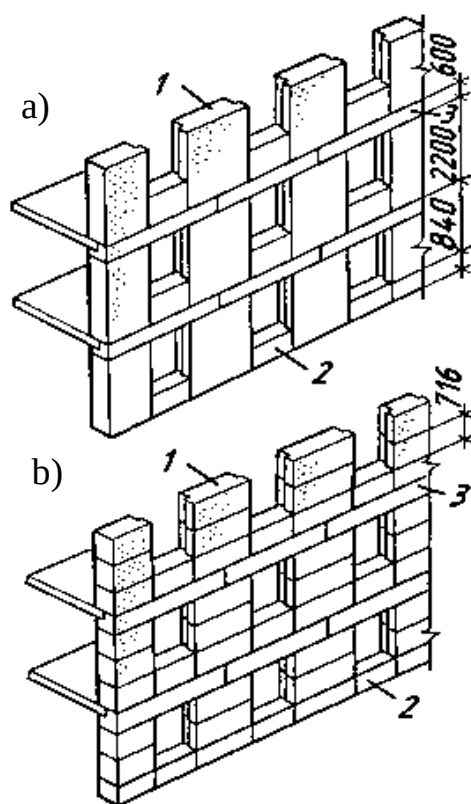
2.76-rasm. Yirik blokli bino sxemalari:
