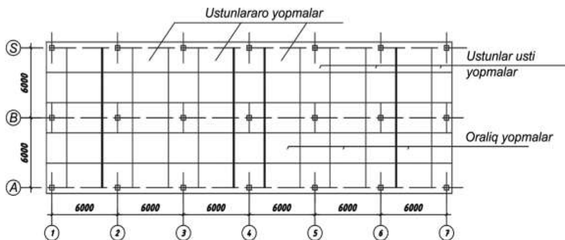
A) Ko'ndalang va bo'ylama yo'nalishda qavatlararo yopmalarni joylashishi
