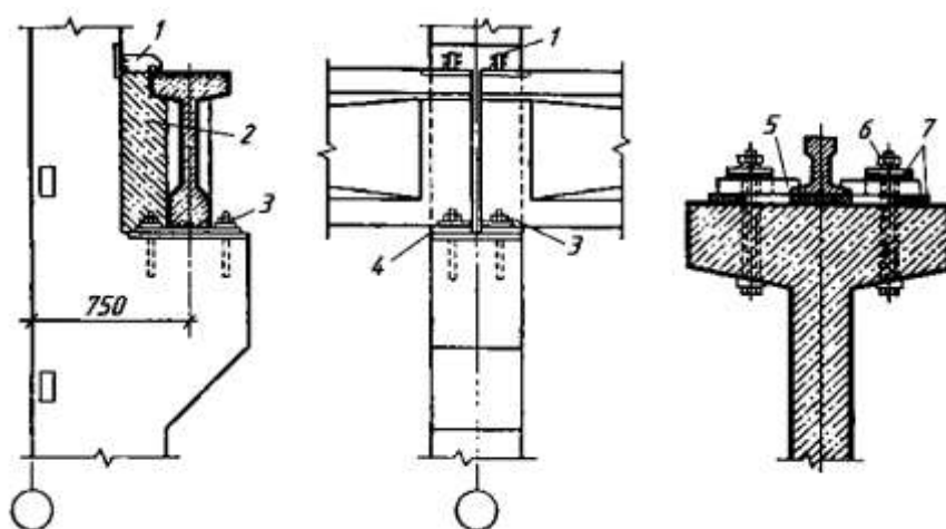
7.11-rasm. Kranosti temirbeton to‘sinlarini ustunlarga qotirish konstruksiyalari: 1 – po‘lat qotirgich plankasi; 2 – beton «to‘sinni montaj va qotirilishidan so‘ng qo‘yiladi»; 3 – shaybalar; 4 – tayanch listi; 5 – siquvchi planka; 6 – bolt; 7 – plastik ostquyma;
