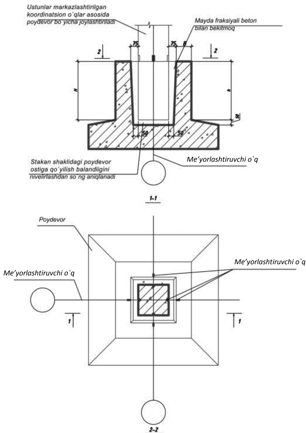
3.7-rasm. Yig'ma ustunlarni stakansimon shakldagi poydevor bilan birikish joyi.
