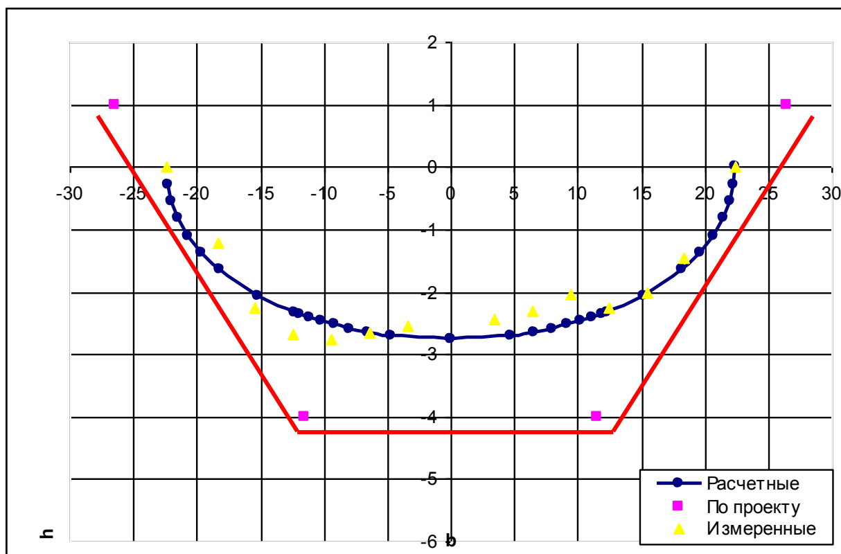
Поперечные сечения канала ПК 620 Q=21,0 м 3 /с (2009г)
