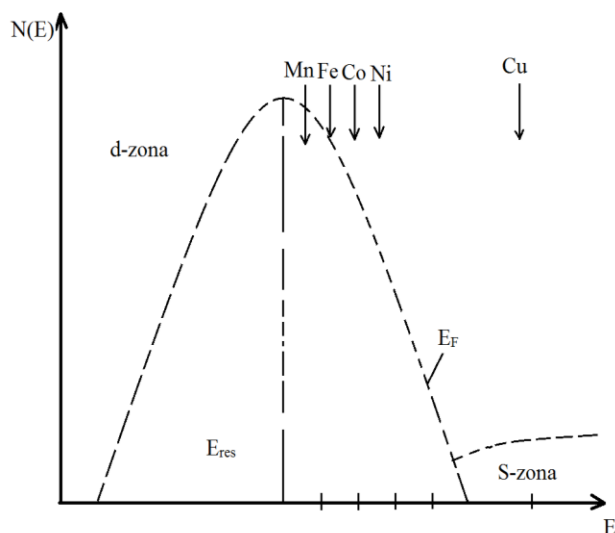
3.2.10.–rasm. E_{res} va E_F ning sxematik ko'rinishi.
