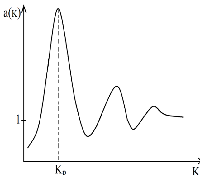
3.2.2.–rasm. Struktura faktorining sxematik ko'rinishi.
