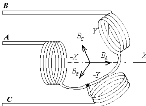
2.1 - Rasm. Uch fazali tok yordamida aylanuvch magnet maydoni hosil qilish sxemasi.
